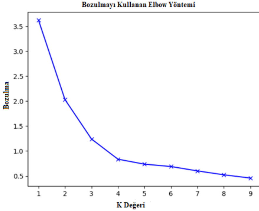
Şekil 2.4. Elbow grafiği [16].
