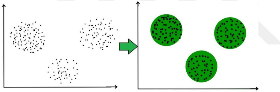
Şekil 2.1. Dairesel gruplama [14].
