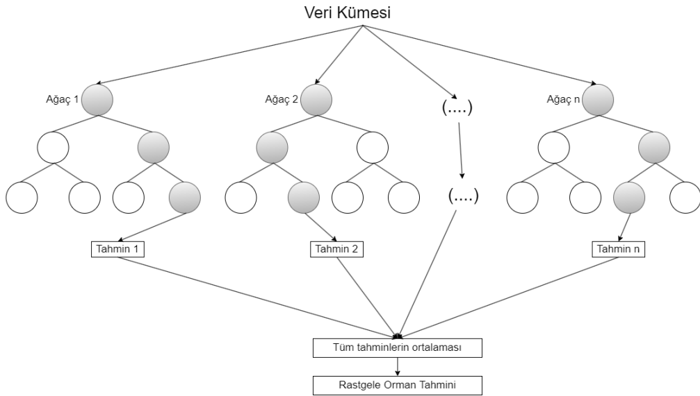
Şekil 3.5. Rastgele Orman Regresyonu
