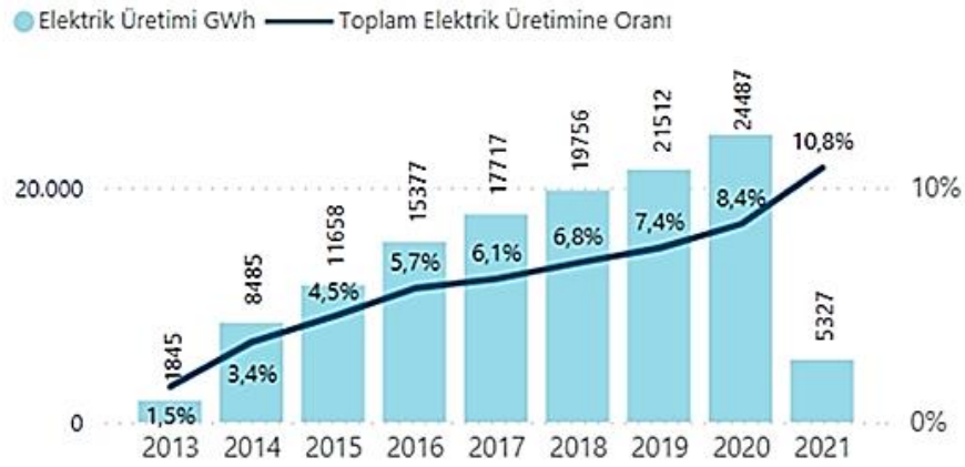
Şekil 3.3. Rüzgar enerjisi yıllık elektrik üretimi ve oranları (TÜREB, 2021b)
