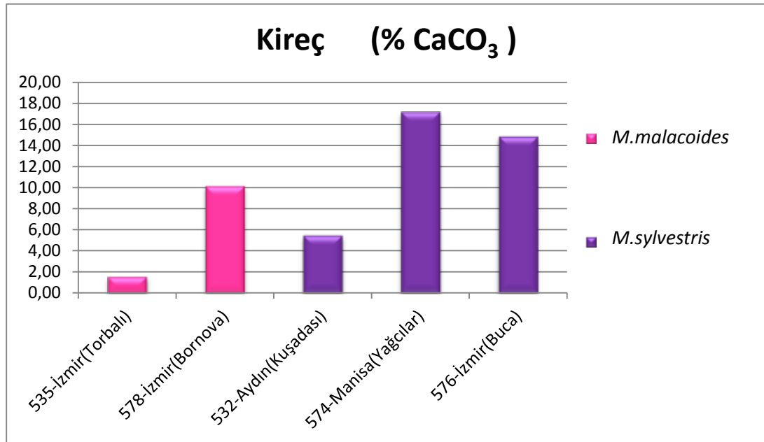
Şekil 4.24. Toprak analizlerine dayalı Kireç ( % \text{CaCO}_3 ) grafiği
