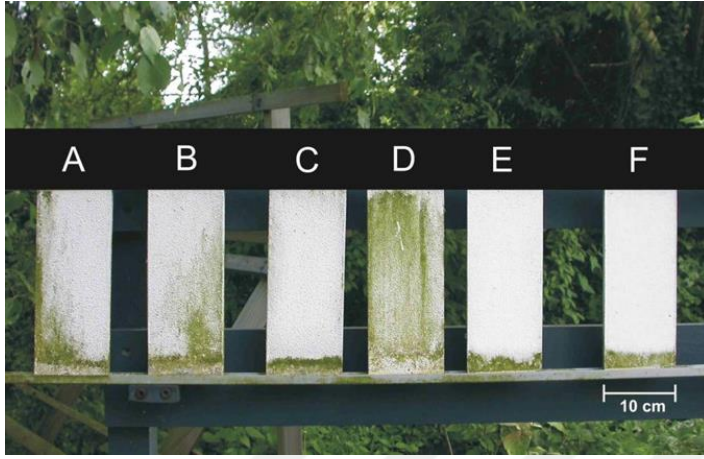
Resim 4.4. Geleneksel boya (A-B-C- D) ve lotus etkili boya (E-F) (Barthlott ve diğerleri, 2007)
