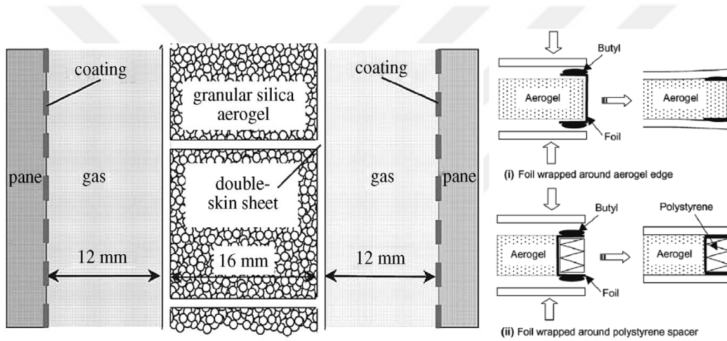
Şekil 4.12. a. Granül silika aerojel b. Monolitik silika aerojel ((Jelle, Beatens ve Gustavsen, 2010)
