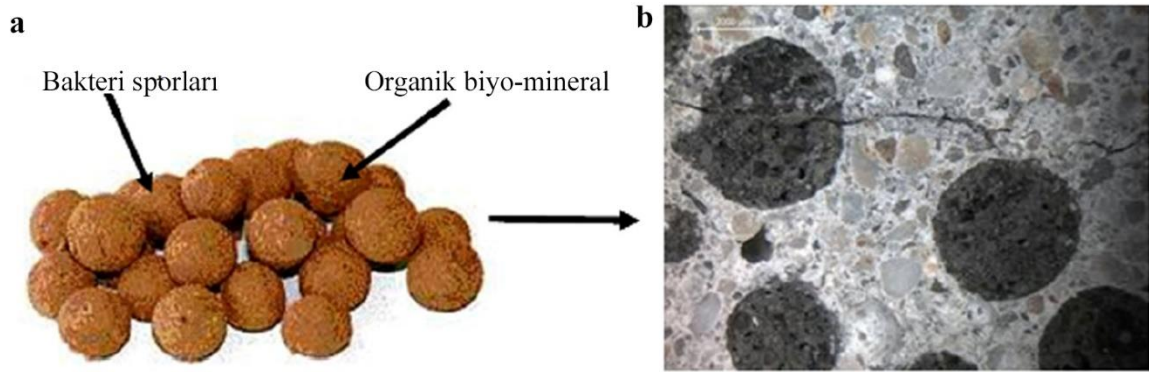
Resim 4.5. a. Bakteri sporları ve organik biyo-mineral (kalsiyum laktat) b. Beton matrisi içine gömülü onarım maddesi (bakteri ve kalsiyum laktat) (Jonkers, 2011)
