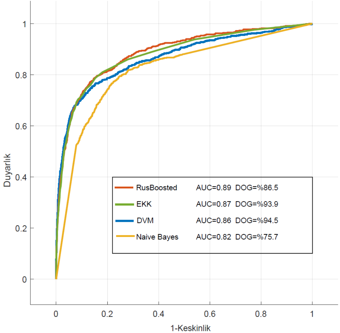
Şekil 3.4. Tüm öz nitelikler için farklı sınıflandırıcıları metodlarının ROC Eğrileri
