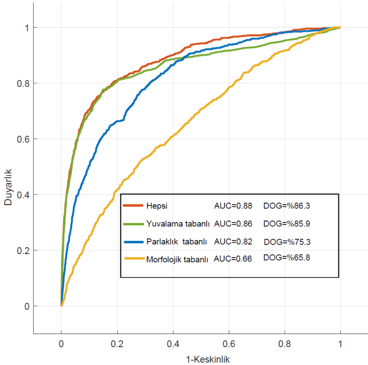
Şekil 3.6. İstatiksel özniteliklerin gruplandırılması ile oluşturulan ROC Eğrileri
