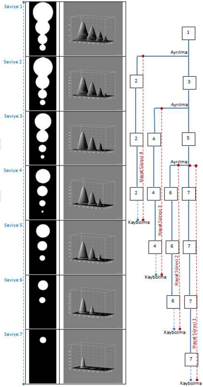
Şekil 2.11. Eşik seviyesi büyürken değişirken ilgi bölgelerinin değişimi
