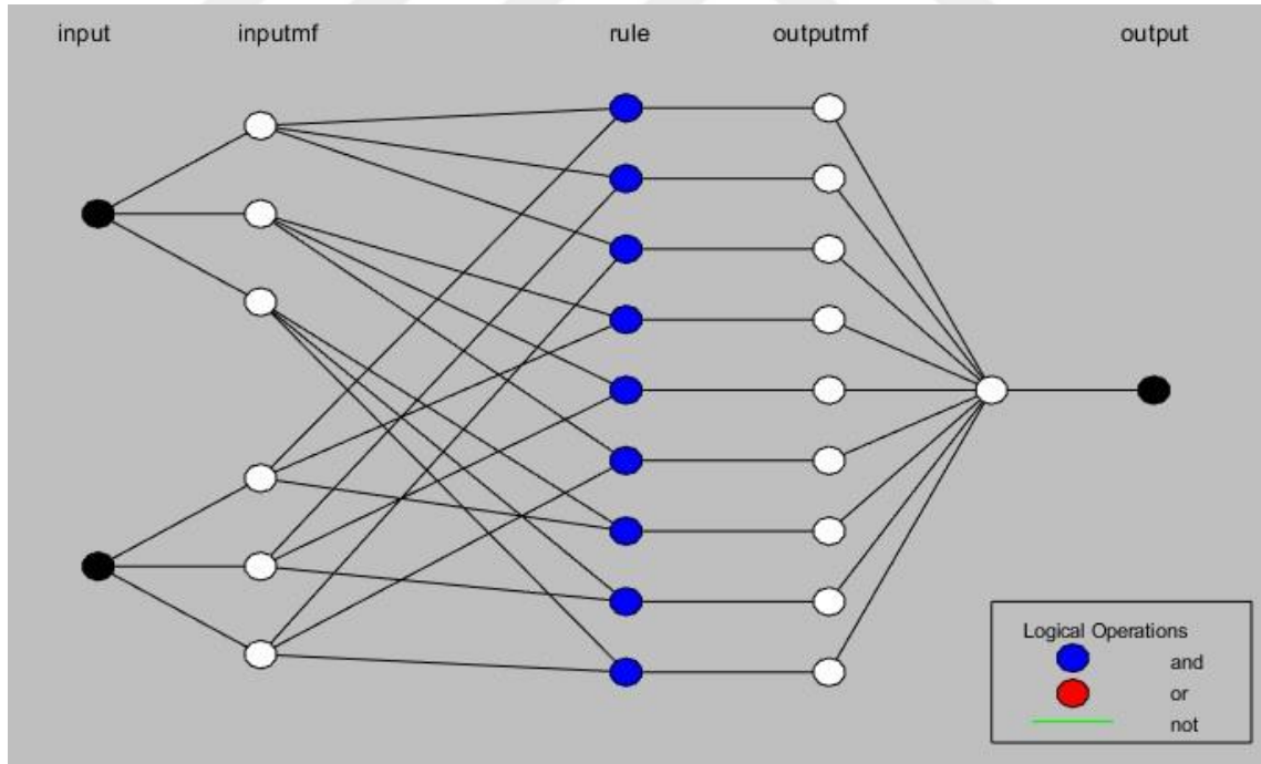
Şekil 4.9. ANFIS modelinin ağ yapısı
