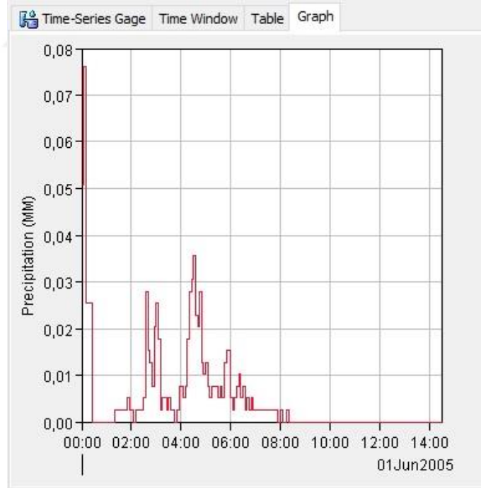
Şekil 3.12. HEC – HMS'de yağış için zaman serisi (Validasyon)
