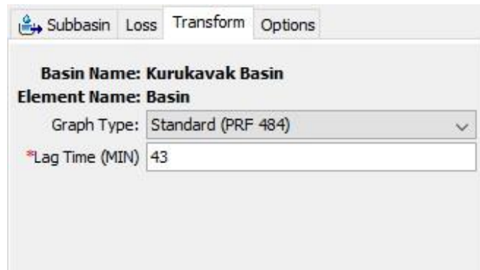
Şekil 3.9. HEC – HMS’de SCS UH dönüşüm metodu
