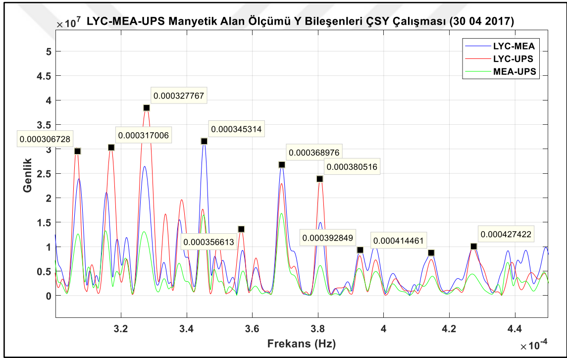
Şekil 32: Gözlemvleri Kaynaklı Manyetik Alan Ölçümü Y Bileşenleri ÇSY
