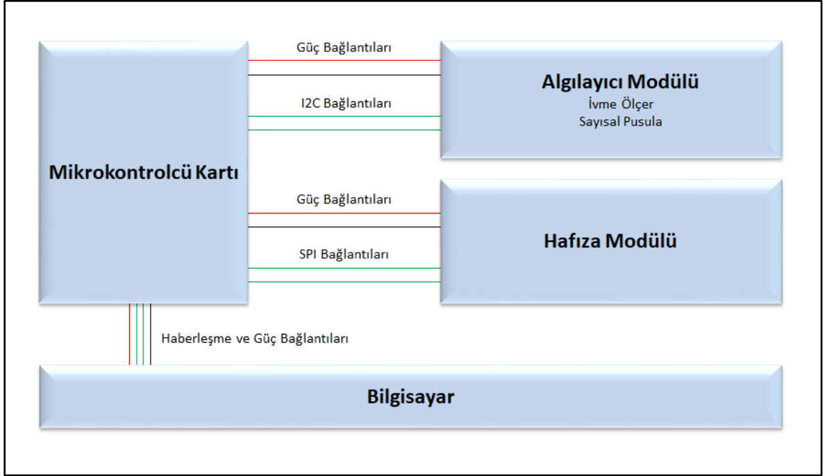
Şekil 15: Test Kurulumu Şematik Gösterimi
