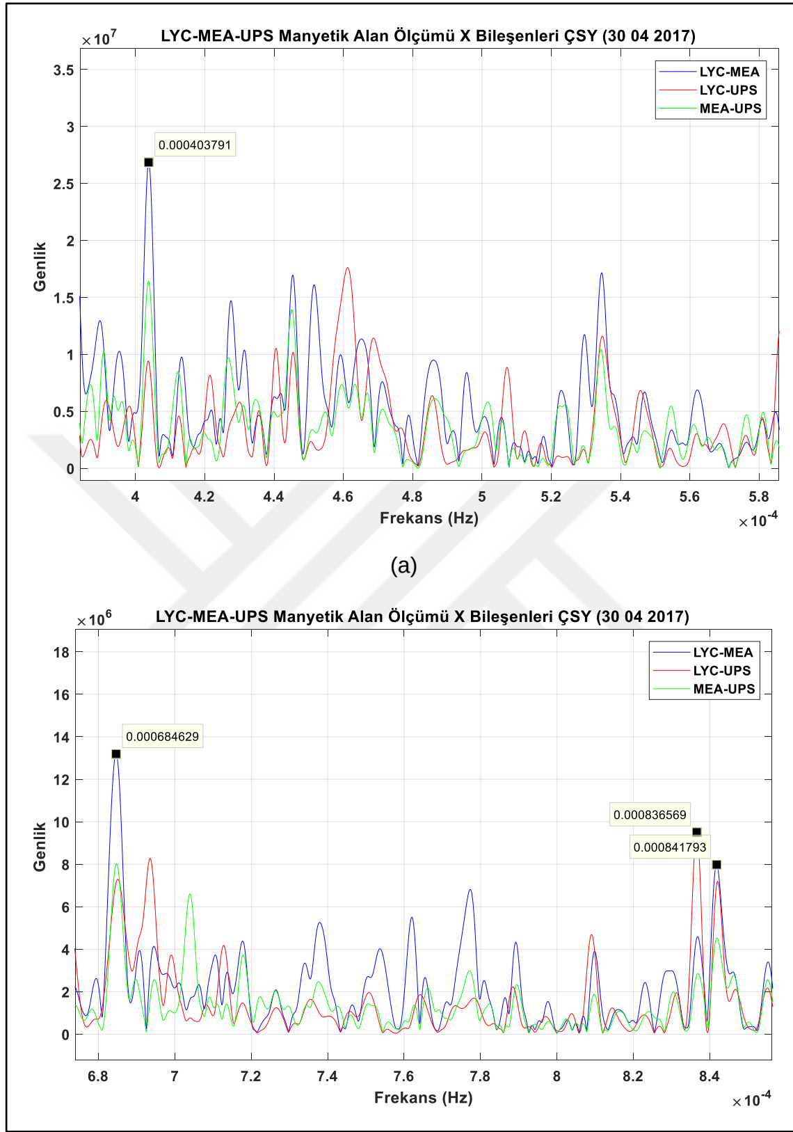
Şekil 33: Gözlemleri Kaynaklı Manyetik Alan Ölçümü X Bileşenleri ÇSY
