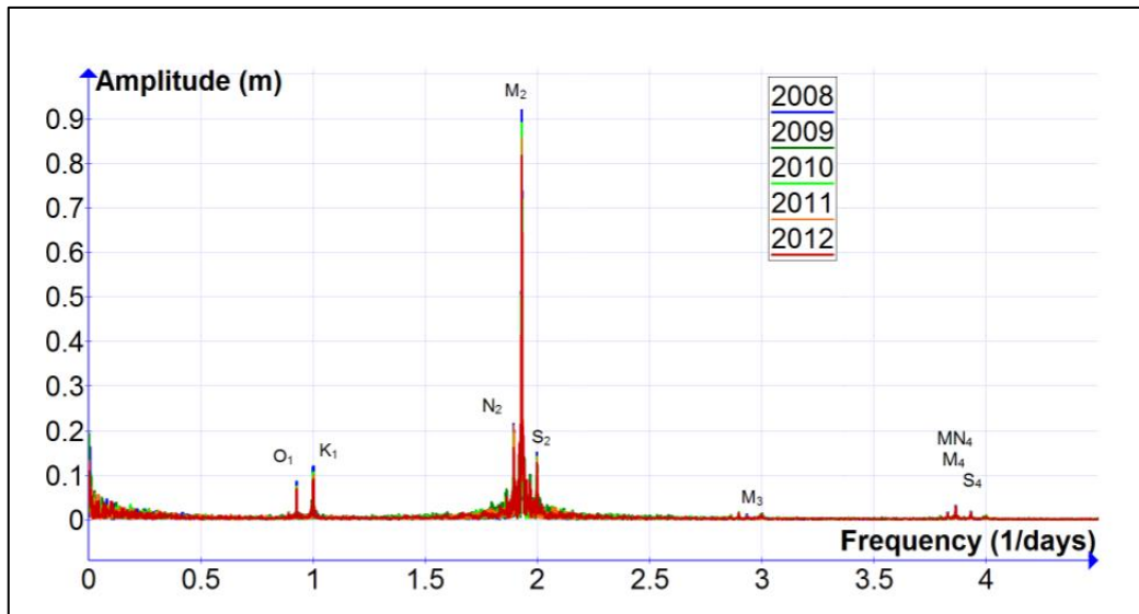
Şekil 14: Gelgit Dalgalarının Frekans-Genlik Gösterimi [41]
