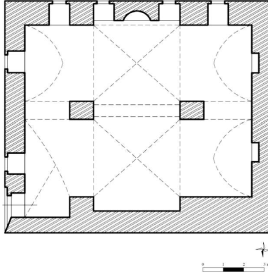
Şekil 25. Molla Hari (Halil / Süleyman Paşa) Cami'nin Planı (Arslan, 2017, s. 1050)
