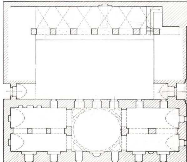
Şekil 19. Abdullatif Cami 'nin planı (Altun, 1978a, s. 102; 2011, s. 40)
