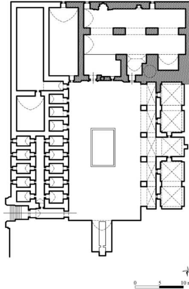
Şekil 38. Şehidiye Medresesi'nin planı / Aptullah Kuran'dan işlenerek (Arslan, 2017, s. 2130)
