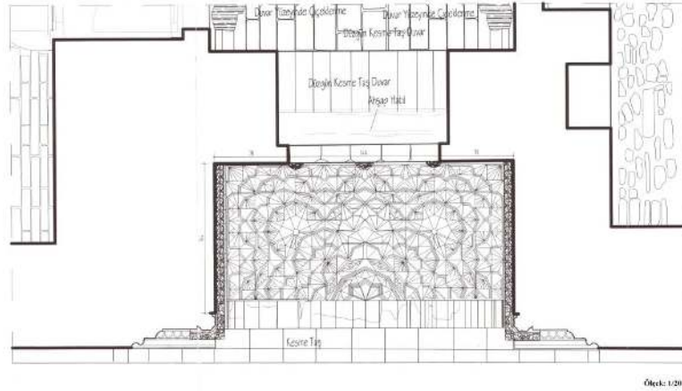
Şekil 22. Taç kapı örtü unsurunun yatay kesit planı / ö: 1/20 (Mimar Duyan ve Karaşin vd., D.V.B.M. arşivi, 2016)
