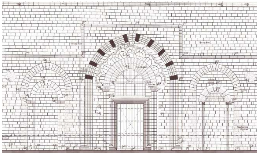
Şekil 11. Taç kapının cephe çizimi / ö: 1/50 (Ş.K.V.K.B.K.M. arşivi)
