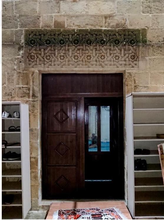
Görsel 93. Harimin giriş açıklığı ve yenilenen süsleme şeridi
