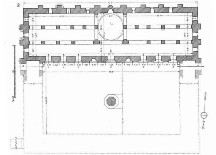
Şekil 8. Kızıltepe Ulu Cami'nin planı / 1932 (Gabriel, 2014, s. 58)
