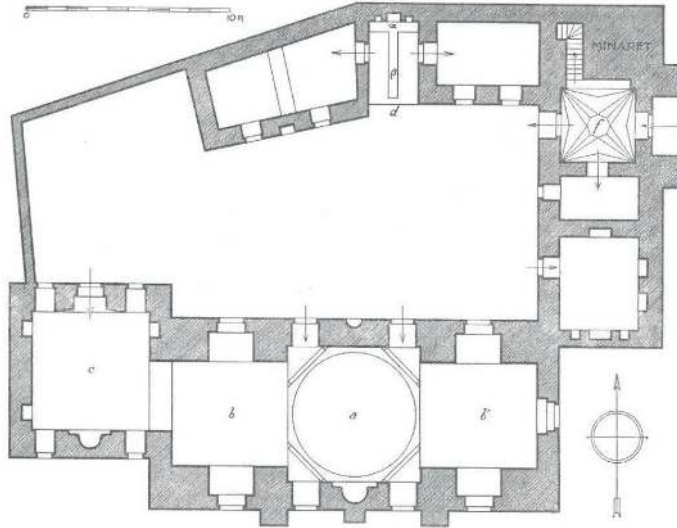
Şekil 14. Melik Mahmud Cami'nin planı / 1932 (Gabriel, 2014, s. 38)
