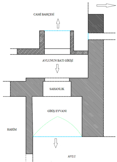
Şekil 23. Avlunun batı girişinin ve eyvanının yatay kesit planı
