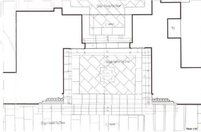
Şekil 21. Taç kapının yatay kesit planı / ö: 1/20 (Mimar Duyan ve Karaşin vd., D.V.B.M. arşivi, 2016)
