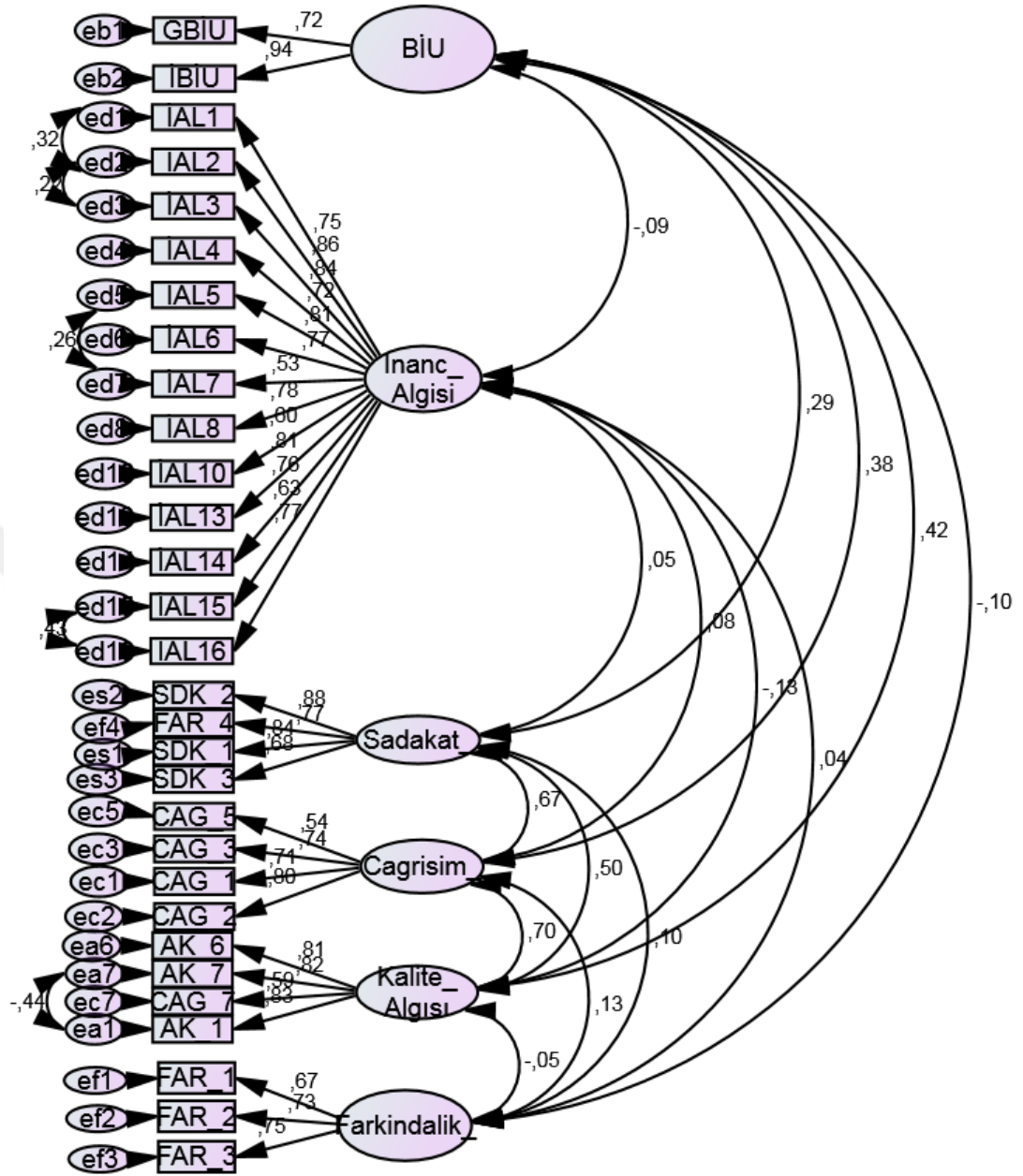
Şekil 19: Ölçüm Modeli İçin Birinci Dereceden DFA Modeli
