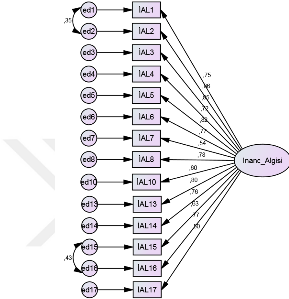
Şekil 17: 1. Modifikasyon Sonrası İnanç Algısı Gizil Değişkenine Ait 1. Dereceden DFA Modeli
