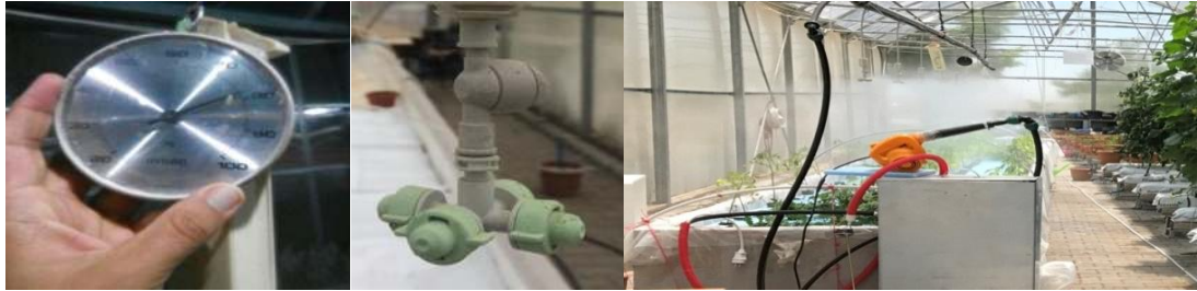
Şekil 17. Nem ölçümü ve kullanılan düşük basınçlı sisleme sistemi
