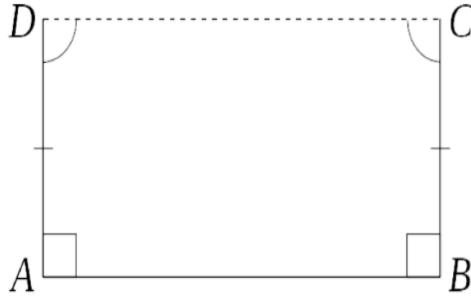
Şekil 1.1: Saccheri dörtgeni Kaynak: Yıldırım, 2018, s.36
