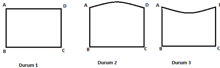
Şekil 1. 2: Saacheri'nin 5. Postulatı reddettiği durumda ulaştığı üç hipotez Kaynak: Kökcü, 2017, s.4
