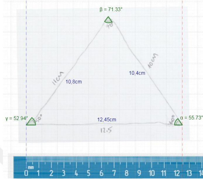
Şekil 45. Sena'nın KKK benzerliğiyle ilgili pantograftaki üçgen çizimi ve kontrolü
