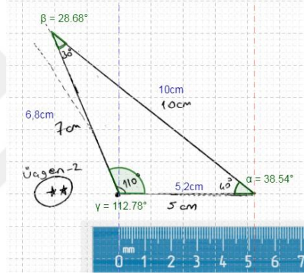
Şekil 145. Sema'nın AKA benzerliğiyle ilgili üçgen çizimi ve kontrolü
