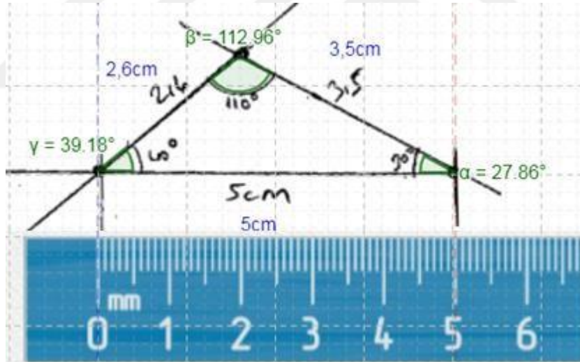
Şekil 65. Esma'nın KKK benzerliğiyle ilgili üçgen çizimi ve kontrolü
