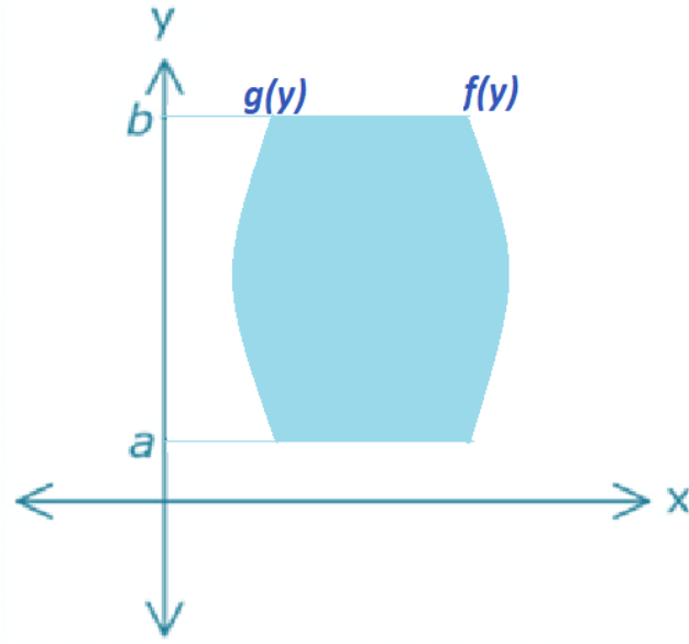
Şekil 2.5. x = f(y) ve x = 0 eğrisi altında kalan alan
