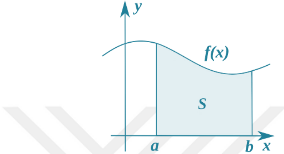
Şekil 2.3. Bir fonksiyon eğrisinin altında kalan alan
