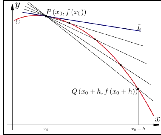
Şekil 2. y=f(x) eğrisinin P(x_0, f(x_0)) noktasındaki teğetinin eğimi \lim_{h \rightarrow 0} \frac{f(x_0 + h) - f(x_0)}{h}
