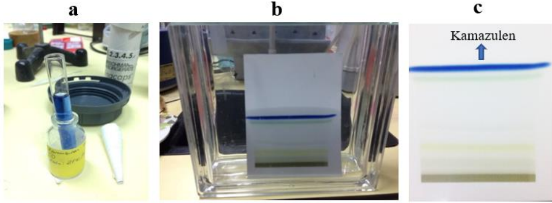
Şekil 4.11. Kamazulenin prep-İTK ile izolasyonu [kamazulen-etanol çözültisi (a); aseton/ n -hekzan 1,5:98,5 çözücü sisteminde develope edilen kamazulen (b); kamazulenin gün ışığında görüntülenen İTK kromatogramı (c)]
