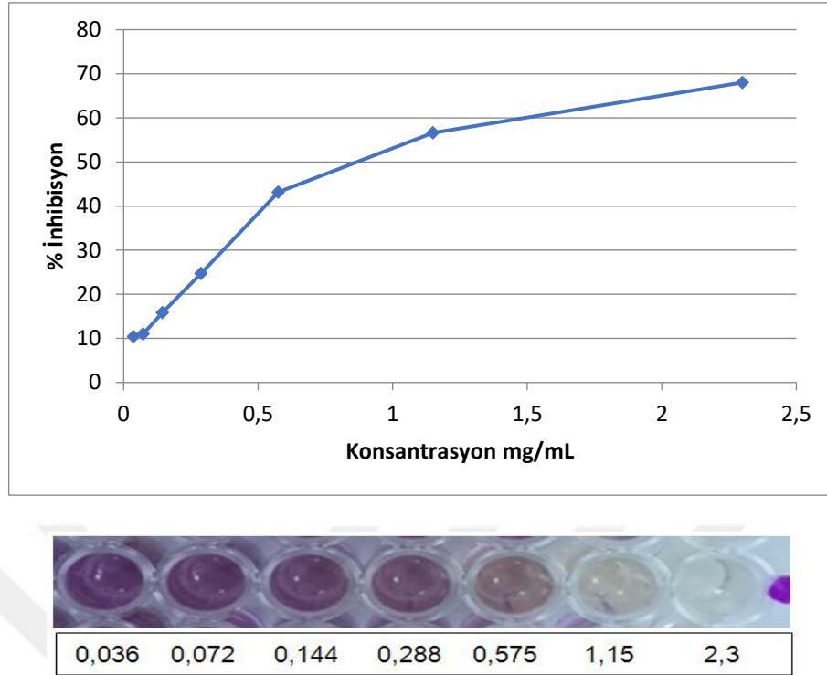
Şekil 4.34. B. cinerea ekstresinin DPPH radikal süpürücü etkisi [Ekstrenin farklı konsantrasyonlarının 517 nm’de ölçülen DPPH absorpsiyona bağlı %inhibisyon grafiği (üstte) ve ekstenin farklı konsantrasyonlarda (mg/mL) DPPH* ile reaksiyonu sonucu mikroplakada gözlenen renk değişimi (altta)]
