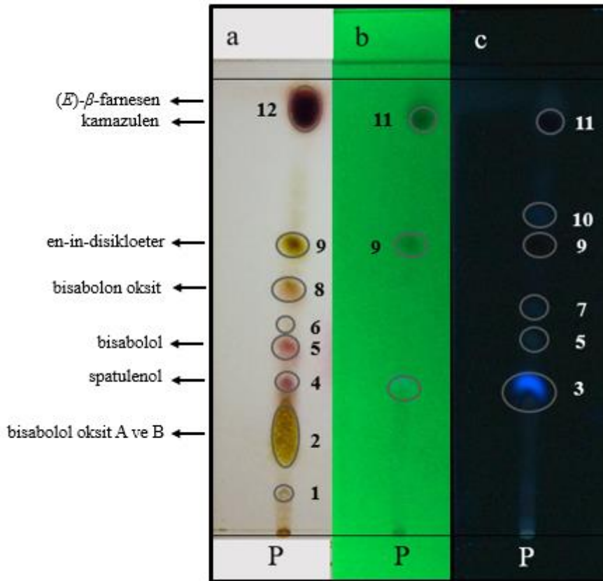
Şekil 4.8. Papatya uçucu yağının İTK profilindeki spotların belirlenmesi
