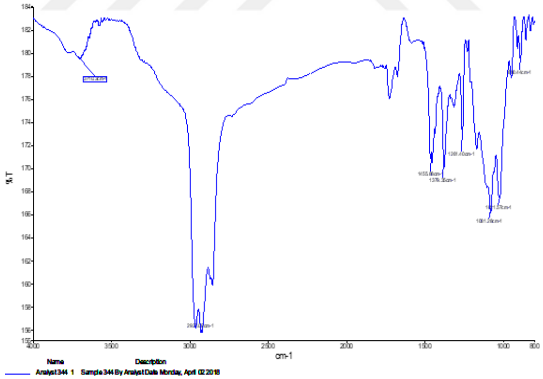
Şekil 4.29. BE1 metabolitin FT-IR spektrumu
