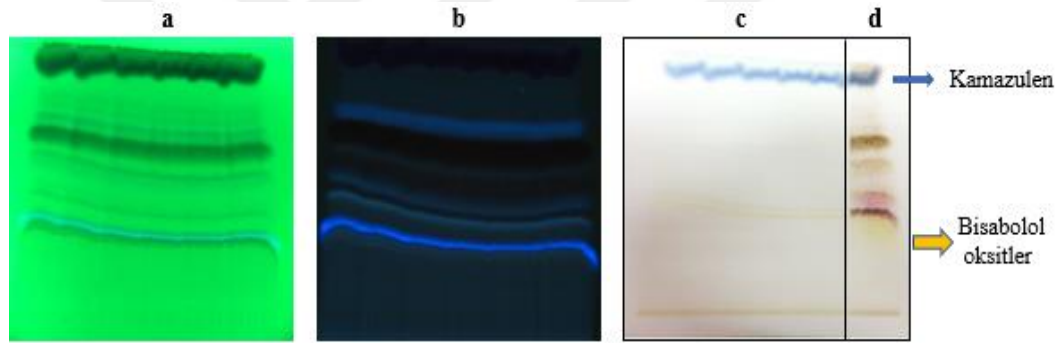
Şekil 4.9. Papatya uçucu yağının prep-İTK kromatogramı [254 nm'de (a); 366 nm'de(b); gün ışığında (c) anisaldehyt-sülfürik asit reaktifi ve ısı muamelesi sonrası gün ışığında (d), çözücü sistemi kloroform/toluen 75:25]
