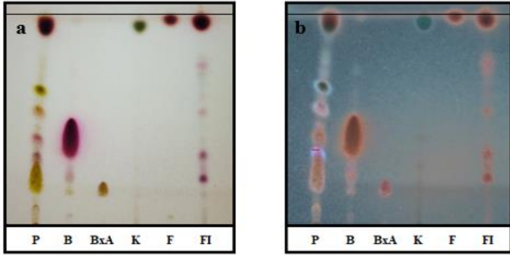
Şekil 4.5. Papatya uçucu yağı ve standart maddelerin İTK kromatogramları-II [anisaldehit-sülfürik asit reaktif ve ısı muamelesi sonrası gün ışığında (a); reaktif ve ısı muamelesi sonrası 366 nm 'de (b); papatya uçucu yağı (P); (-)- \alpha -bisabolol (B); bisabolol oksit A (BxA); kamazulen (K); (E)- \beta -farnesen (F); farnesen izomerleri karışımı (FI); çözücü sistemi kloroform/toluen 75:25; reaktif: anisaldehit-sülfürik asit]
