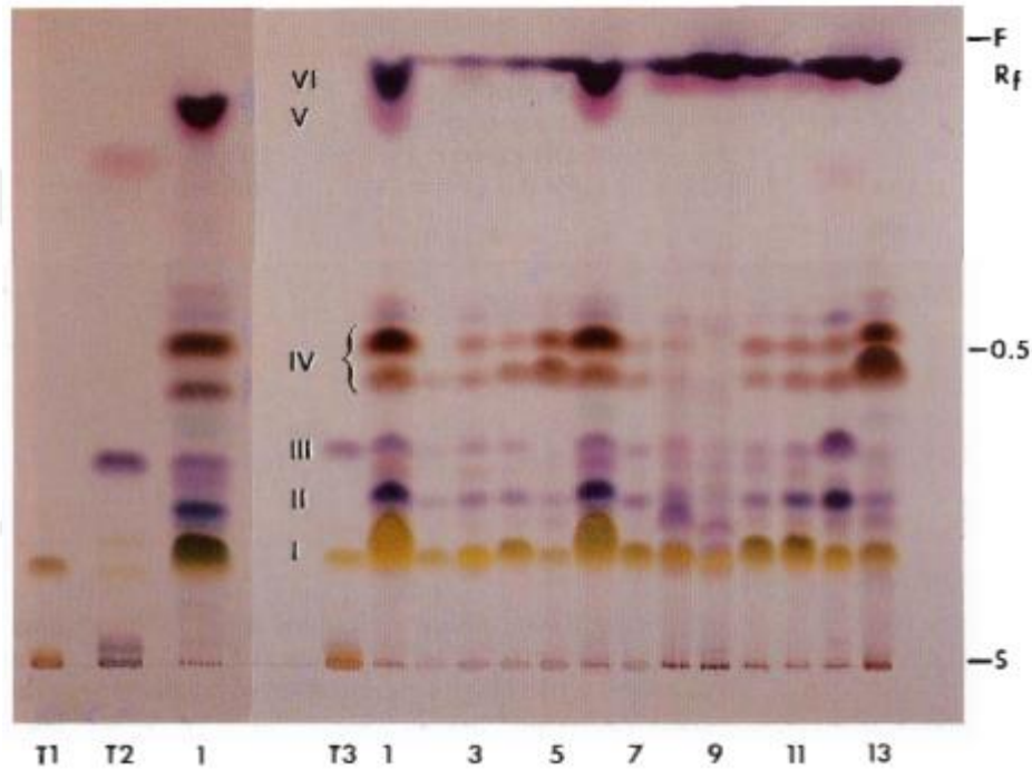
Şekil 4.7. Farklı tip papatya uçucu yağlarının İTK profili (Wagner ve Bladt, 1996) (Toluen/etil asetat 93:7 çözücü sistemi ile vanilin-sülfürik asit reaktifi ve ısı muamelesi sonrası gün ışığında. T1 bisabolol oksit A; T2 bisabolol ( R_f 0,35 ) ve azulen ( R_f 0,85 ); T3 bisabolol oksit A ve bisabolol; I bisabolol oksit A/B; II spatulenol; III bisabolol; IV poliinler, V azulen, VI farnesen)
