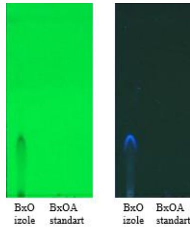
Şekil 4.12. Papatya uçucu yağından izole edilen bisabolol oksitler (BxO) ve bisabolol oksit A standardının (BxOA) İTK profili (Çözücü sistemi kloroform/ n -hekzan 95:5)
