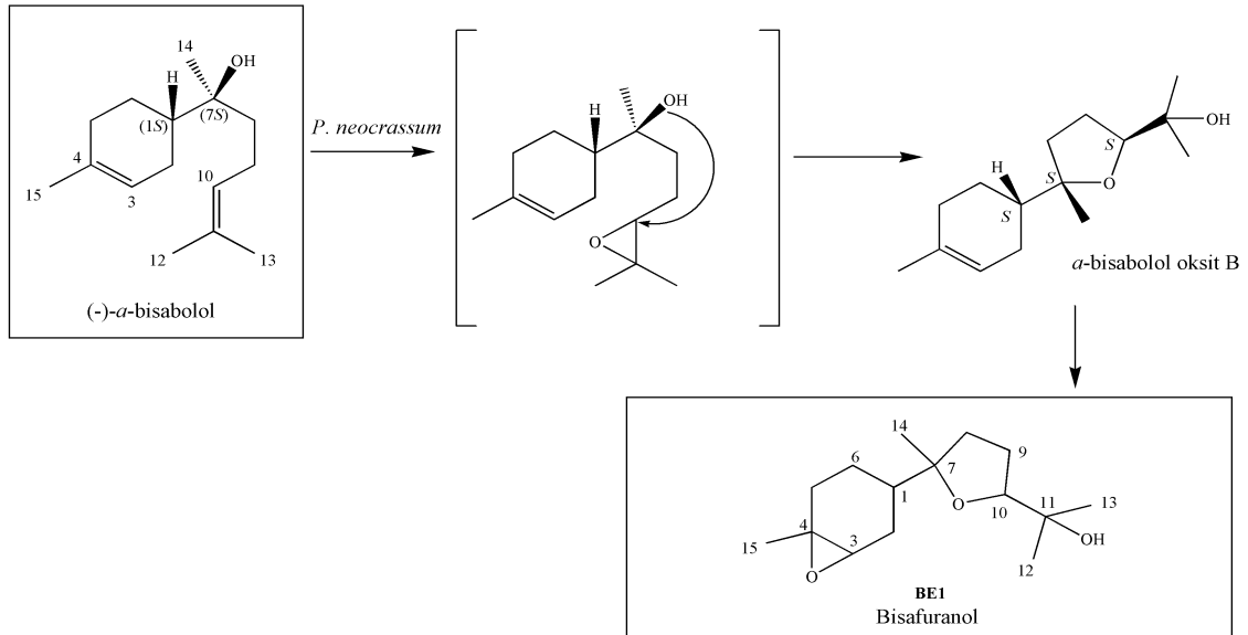
Şekil 4.22. BE1 ( P. neocrassum ) metabolitinin oluşum yolu (Miyazawa vd., 1995; Talapatra ve Talapatra, 2015)
