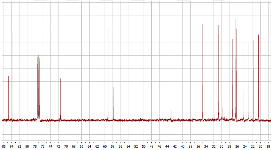
Şekil 4.25. BE1 metabolitin ^{13}\text{C} NMR spektrumu
