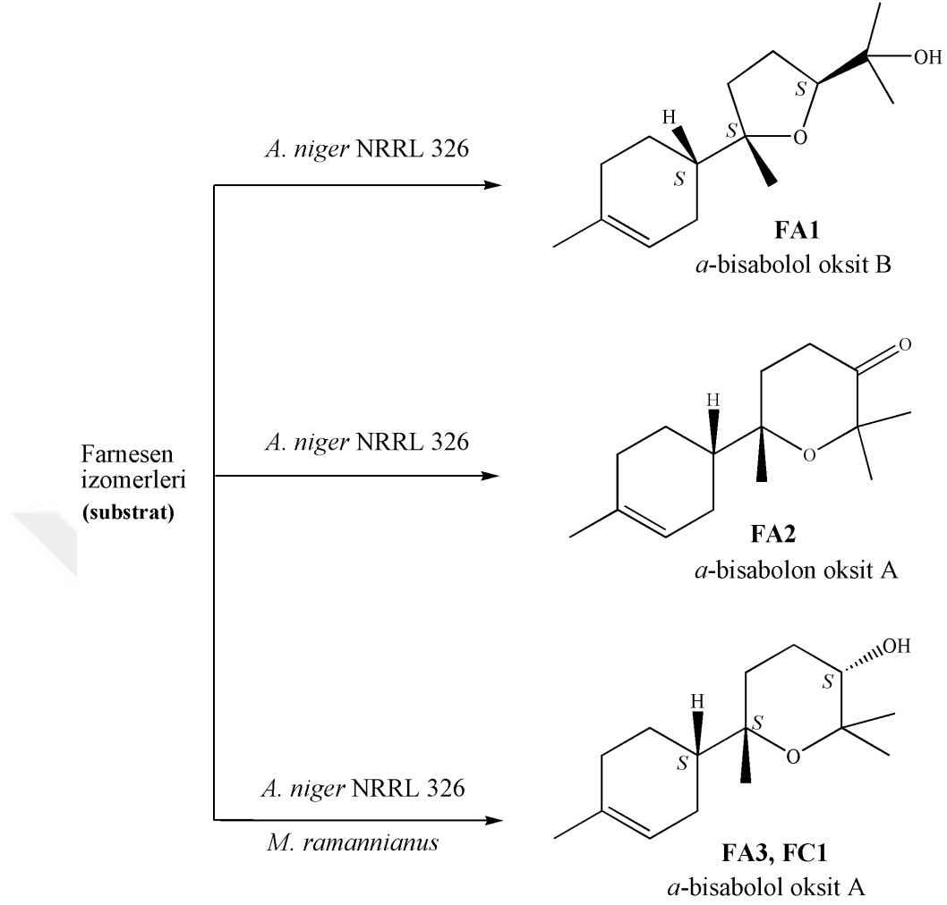
Şekil 4.31. Farnesen izomerleri karışımının A. niger NRRL 326 ve M. ramannianus ile biyotransformasyonu sonucu oluşan metabolitler
