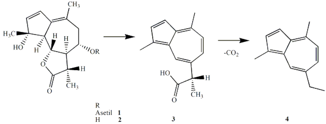
Şekil 2.4. Matrisinin kamazulen molekülüne dönüşümü (Ramadan vd., 2006).
