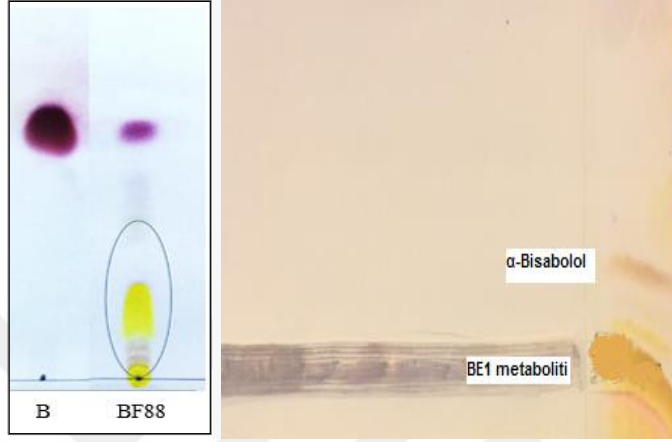
Şekil 4.20. BE1 metabolitinin İTK profili ve prep-İTK ile izolasyonu [ \alpha -Bisabolol ( B ) ve onun P. neocrassum ile biyotransformasyon ekstresi ( BF88 ); çözücü sistemi kloroform/toluen 75:25; reaktif: anisaldehit-sülfürik asit]
