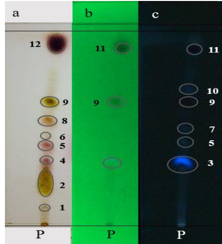
Şekil 4.6. Papatya uçucu yağı İTK profilinde gözlenen spotlar [anisaldehit-sülfürik asit reaktifi ve ısı muamelesi sonrası gün ışığında (a); 254 nm'de (b); 366 nm'de (c); çözücü sistemi klorofom/toluen 75:25]
