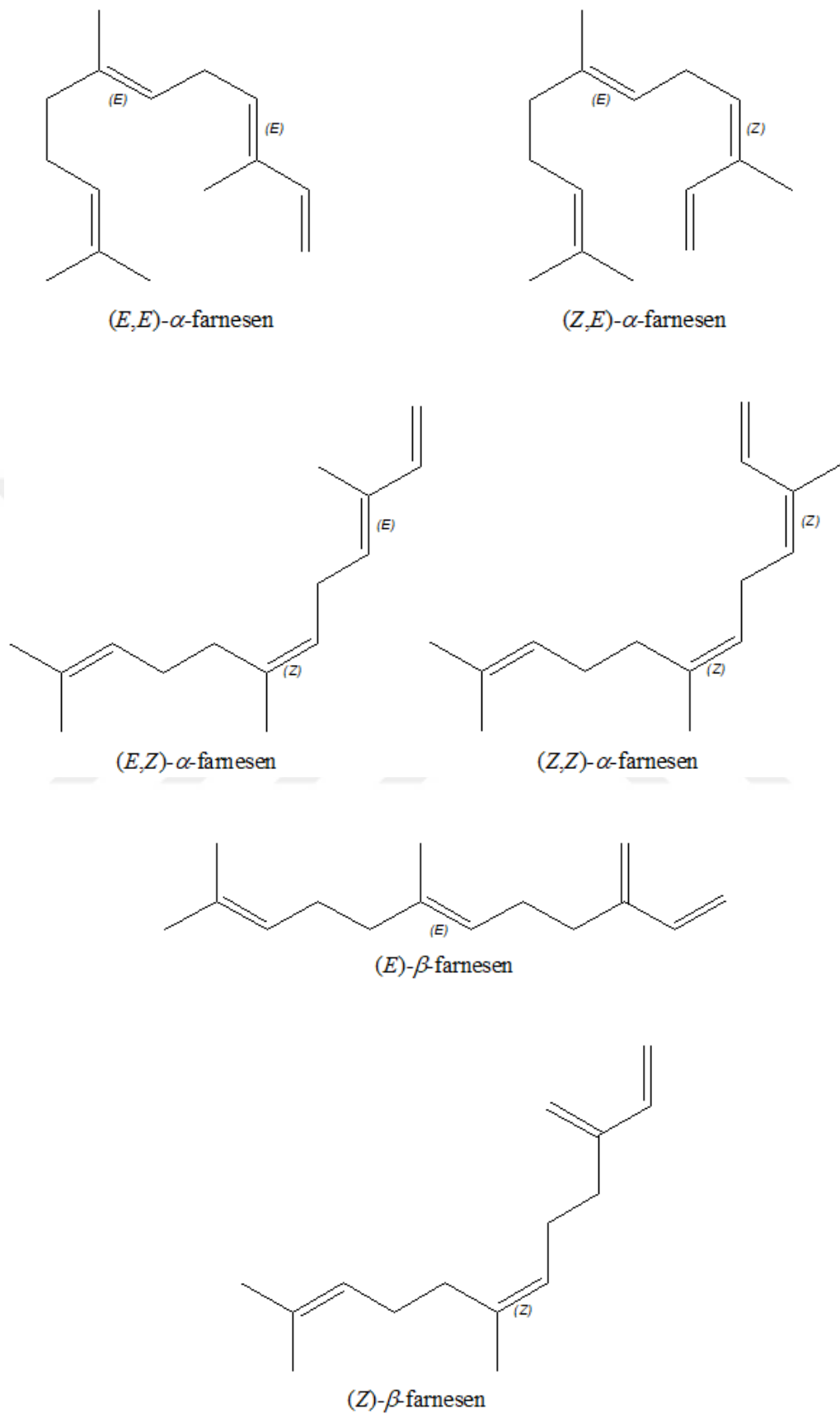
Şekil 2.8. Farnesenin stereoizomerleri
