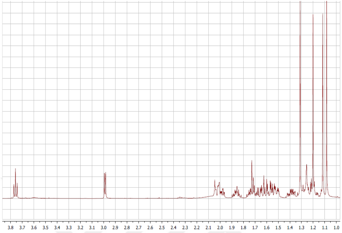
Şekil 4.24. BE1 metabolitin ^1\text{H} NMR spektrumu
