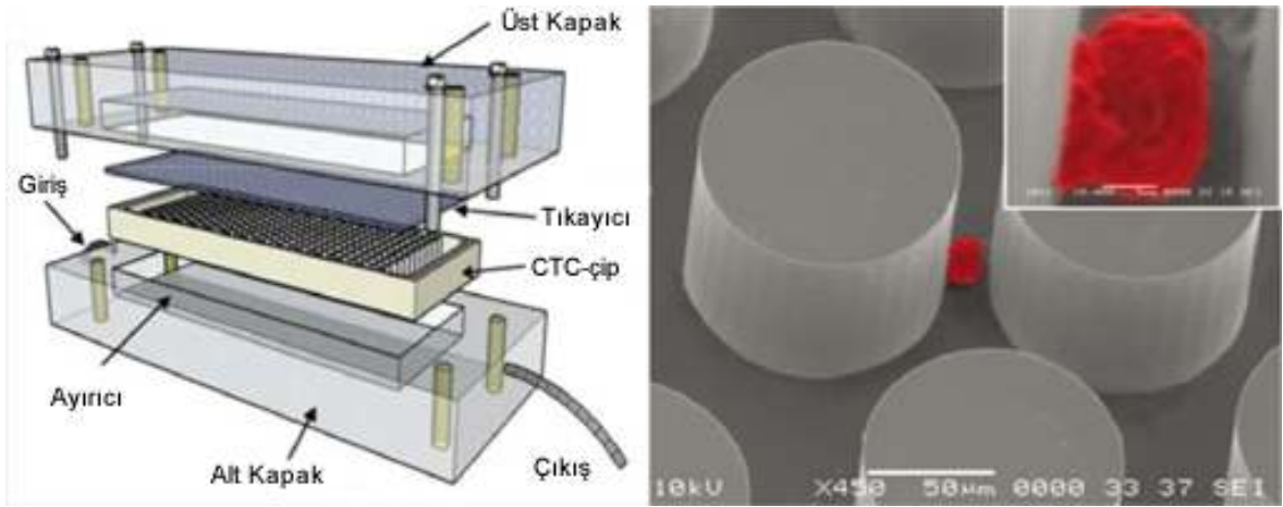
Şekil 2.14 CTC çip [31]
