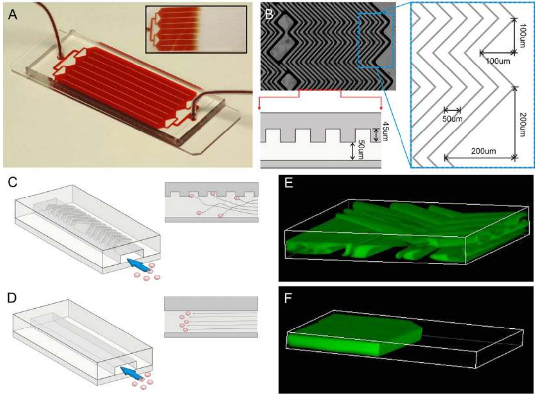
Şekil 2.15 HB çip [52]
