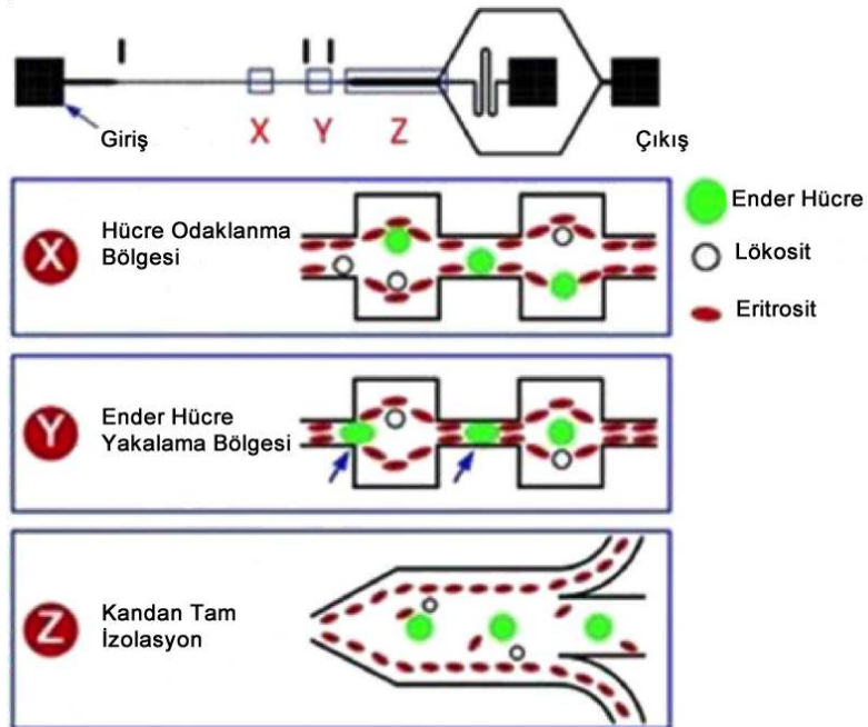
Şekil 2.9 Mikrosıvı akış ayırıştırması [4]
