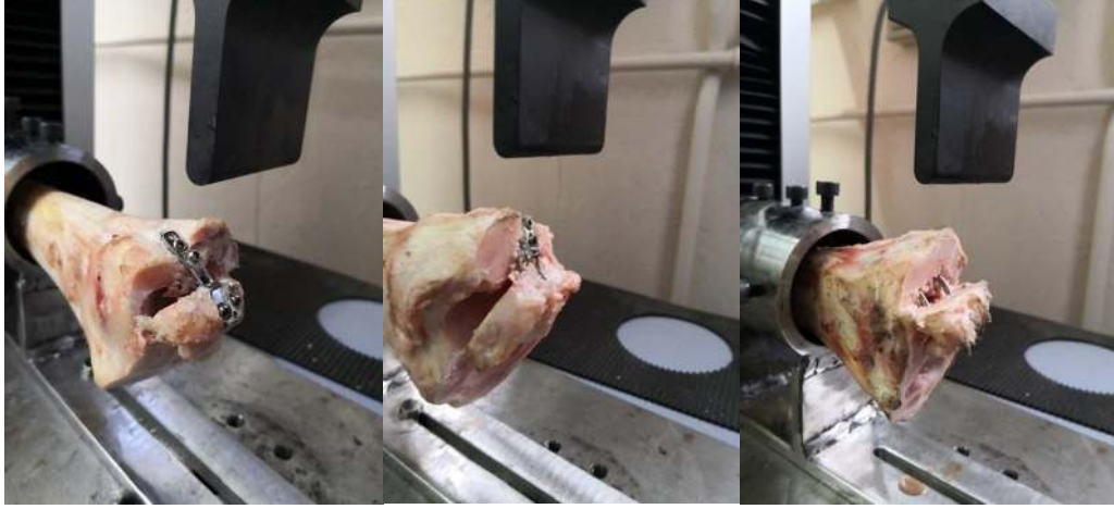
Şekil 34. Transvers kuvvetlerde katastrofik hasar anları
