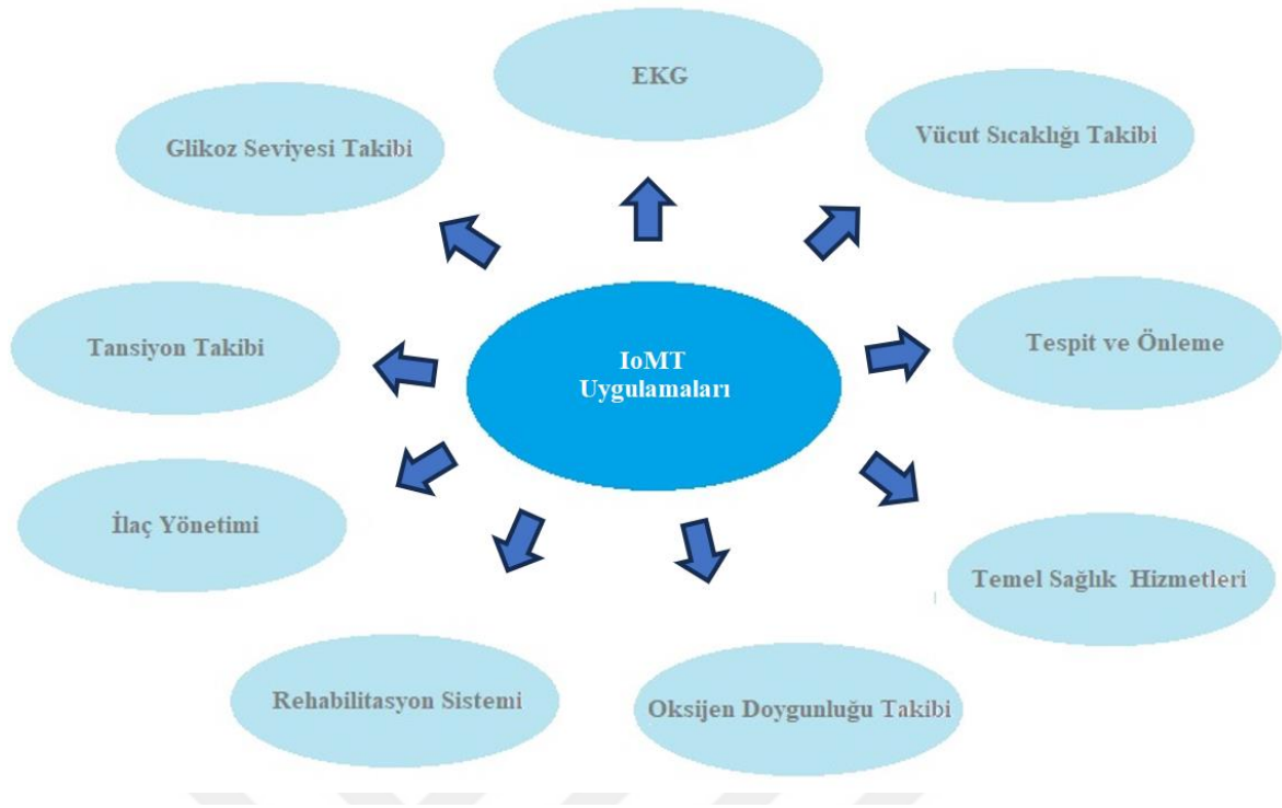
Şekil 1.2. IoMT Uygulamaları
