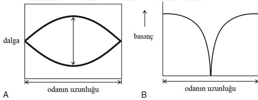
Şekil 3. 39. Bir dalga'nın yarısının oda boyutlarına tam olarak uyduğu frekansta, duran bir dalga oluşur, bu frekansta, basıncı iki duvarda yüksek ve odanın ortasında düşüktür
