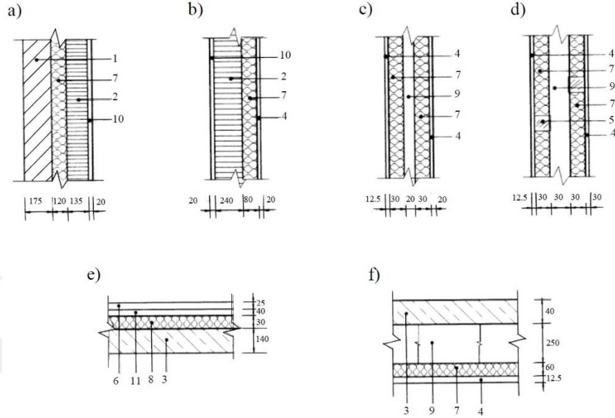
Şekil 3. 38. Değişik ses geçirmezliği bulunan, çok tabakalı elemanlardan oluşan duvar ve döşeme konstrüksiyonlarından örnekler a, b, c, d) Duvar e, f) Döşeme 1) Perde duvar; 2) Tuğla duvar; 3) Betonarme döşeme; 4) Alçı levha; 5) Ahşap; 6) Döşeme Kaplama; 7) Cam yünü; 8) Taş yünü; 9) Hava Katmanı; 10) Sıva; 11) Yapıştırıcı
