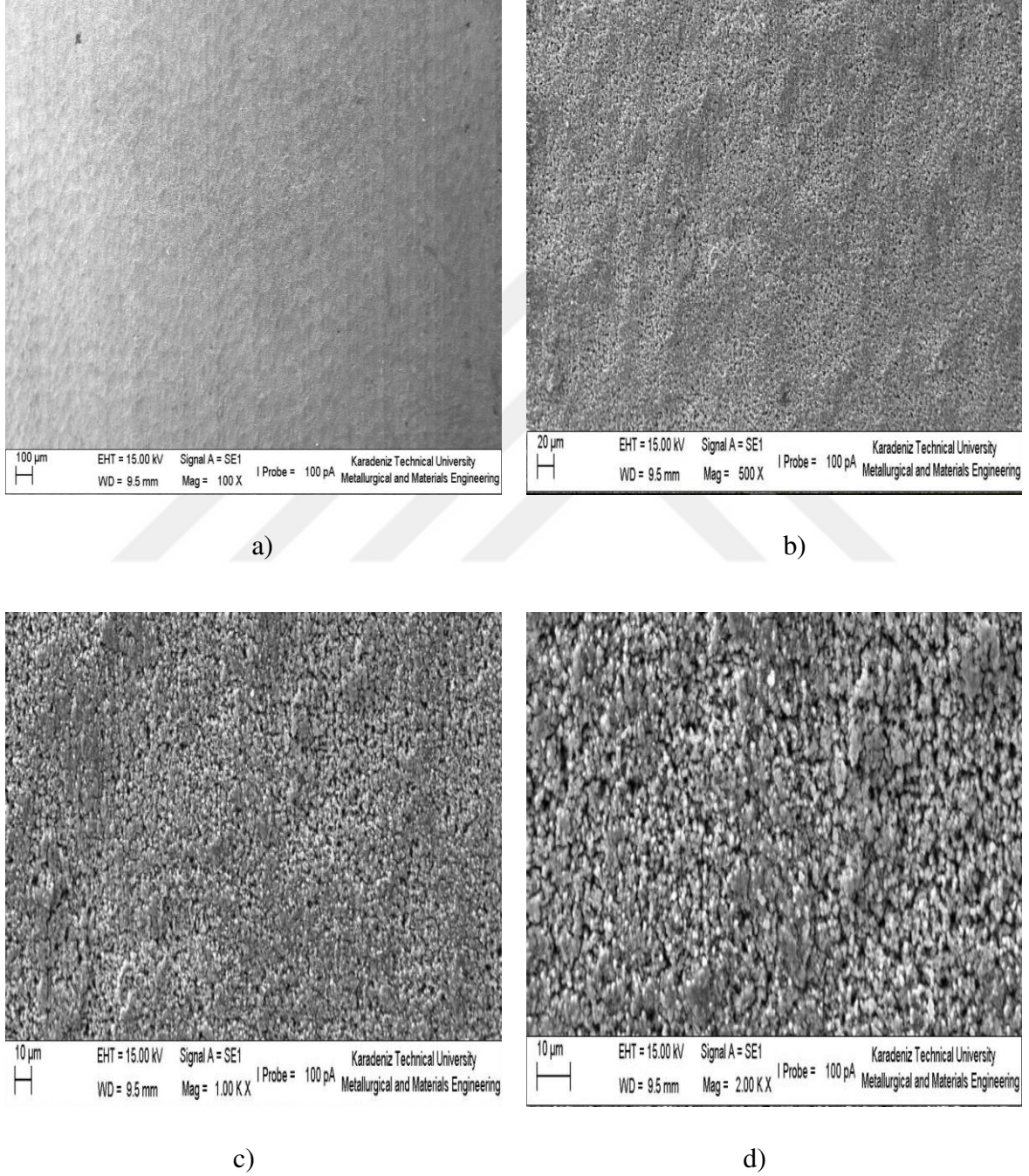
Şekil 3.1. 580°C’ de 2 saat melonite işlemine tabi tutulan numunelerin SEM görüntüleri (a-b-c-d)
