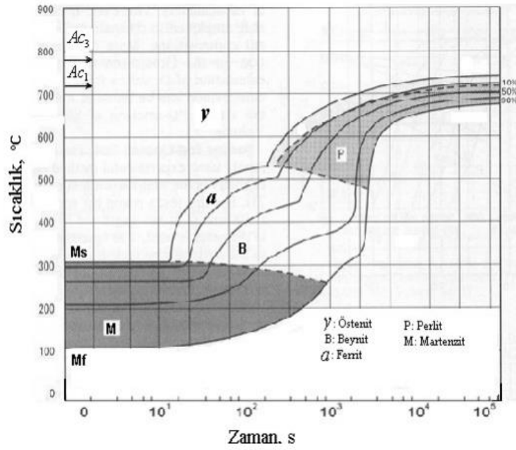
Şekil 1.3. 4140 çeliğine ait CCT diyagramı [18]
