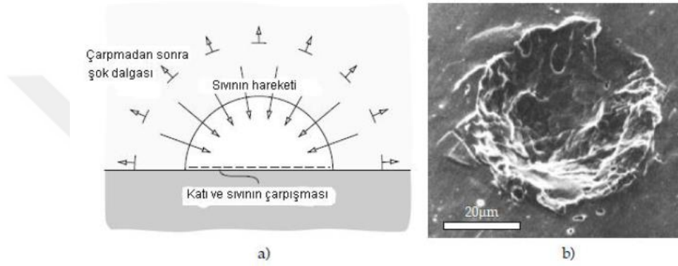
Şekil 1.6. a) Kabarcık çarpmasının mekanizması, b) Deney sonunda metalik malzemede oluşan hasar görüntüsü [19]
