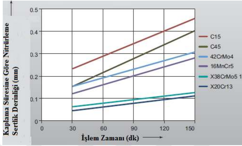
Şekil 1.11. İşlem süresine göre nitrülme sertlik derinliği [26]
