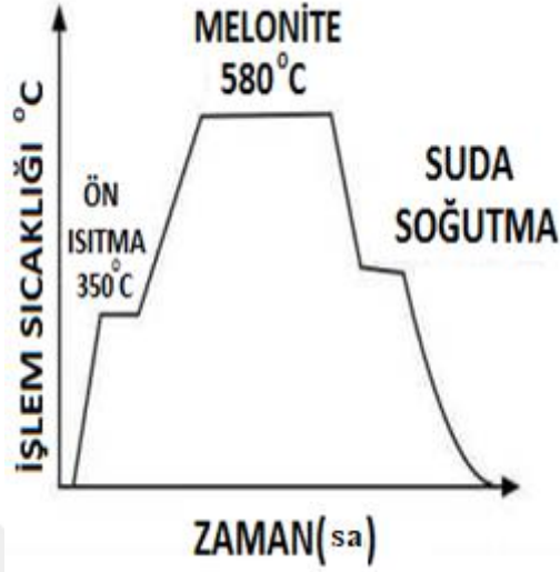
Şekil 1.9. Melonite kaplama yöntemi şematik gösterimi [25]
