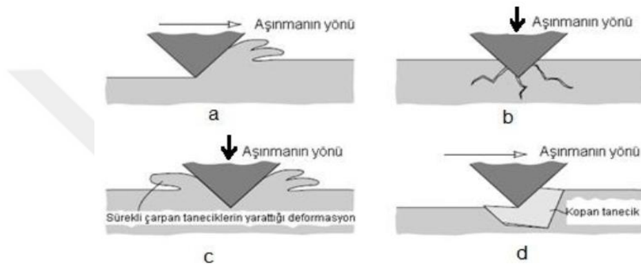
Şekil 1.4. a) Kesme, b) Çatlak, c) Tekrarlı yük nedeniyle yorulma çatlağı, d) Tane kopması [19]
