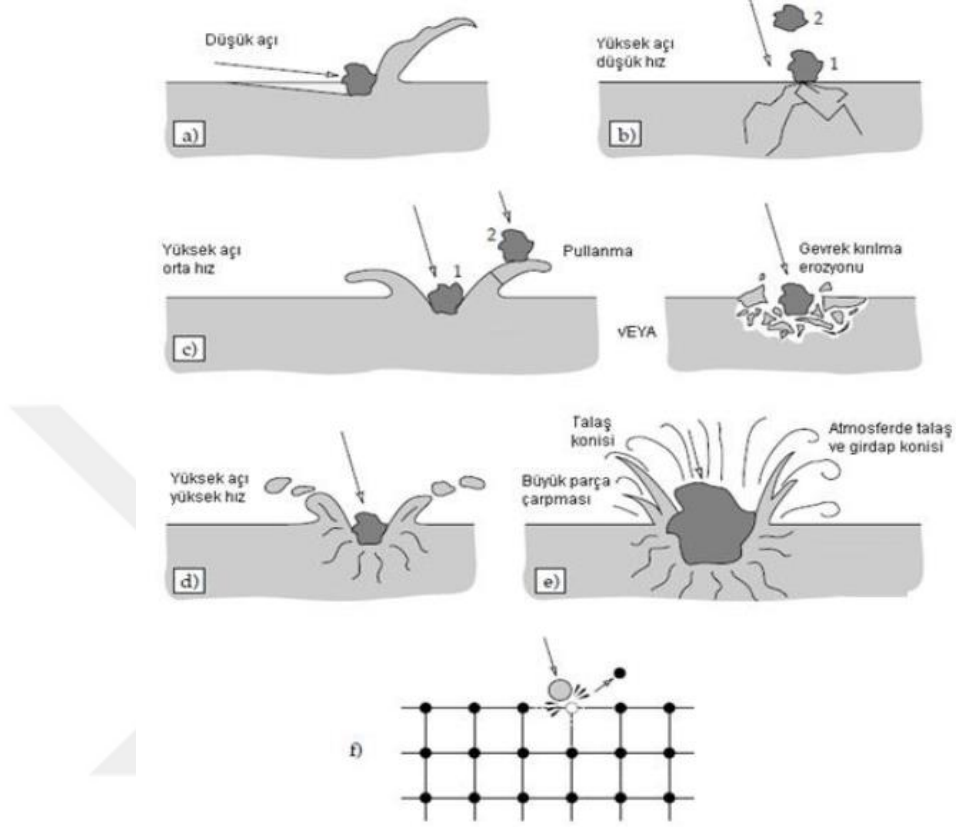
Şekil 1.5. a) Abrasif, b) Yorulma, c) Plastik deformasyon, d) Ergime, e) Ergime- Süperplastik akma, f) Atomik erozyon [19]
