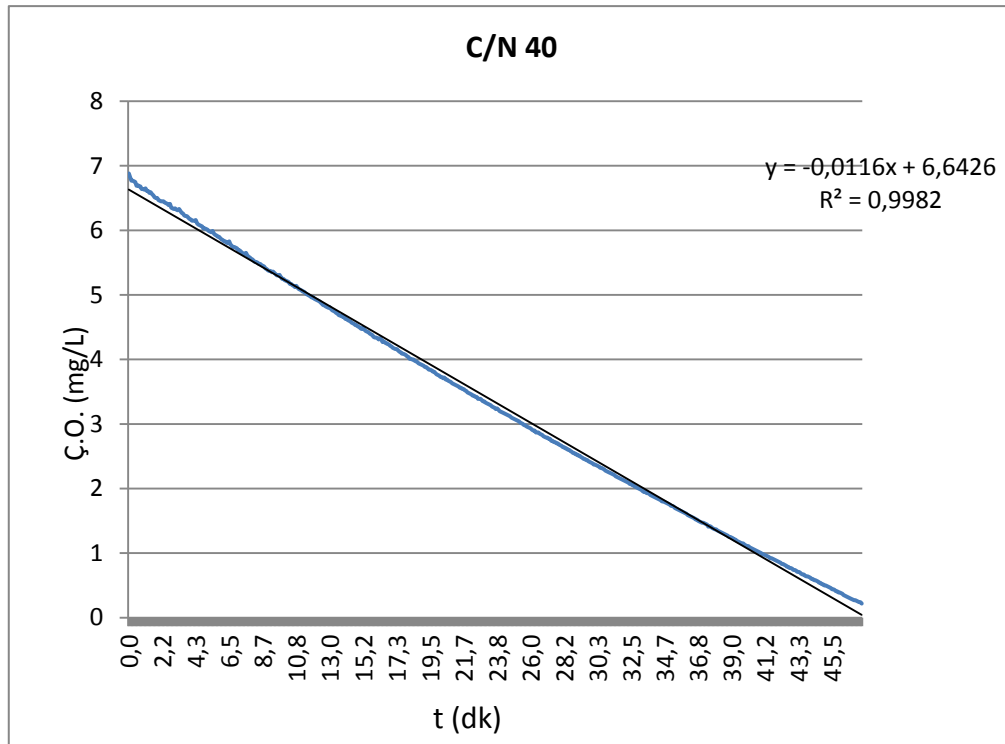
Şekil 5.12 C/N oranı 40 için r_s grafiği
