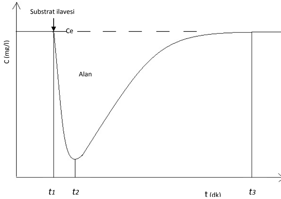
Şekil 3.11 Respirogram [4]
