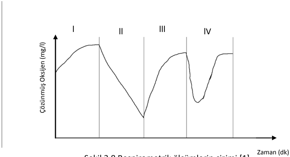
Şekil 3.8 Respirometrik ölçümlerin çizimi [1]
