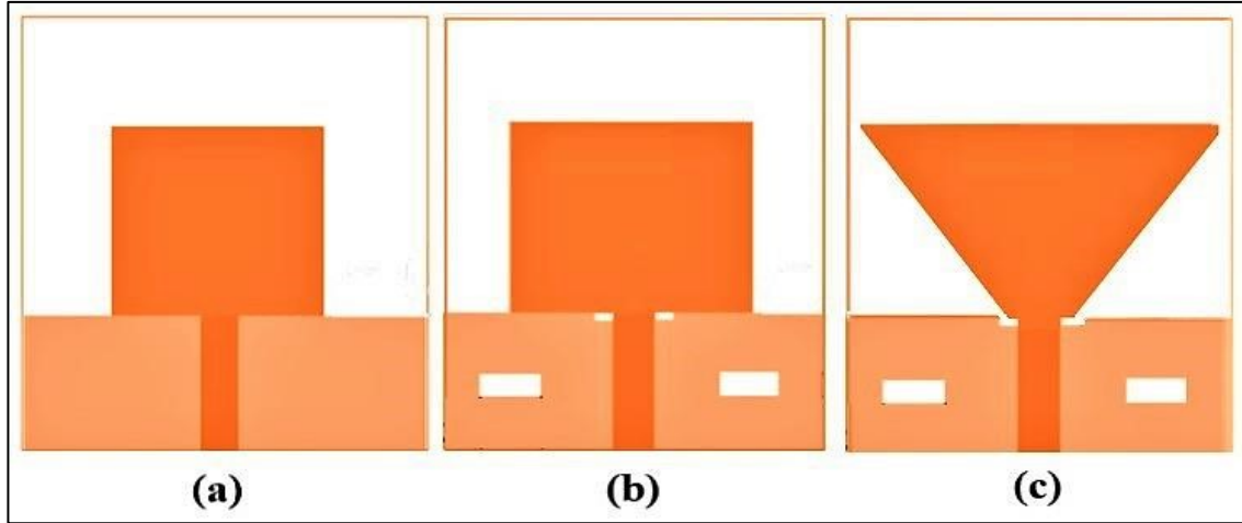
Şekil 3.13. Önerilen dörtgen yamalı DMA'nın tasarım ve gelişim süreci (a: Kare yamalı klasik DMA; b: Çentiğe ve oyuklara sahip toprak yüzeyli DMA; c: Çentikli ve oyuklu toprak yüzeye sahip ve ısıma yaması düzenlenmiş DMA)
