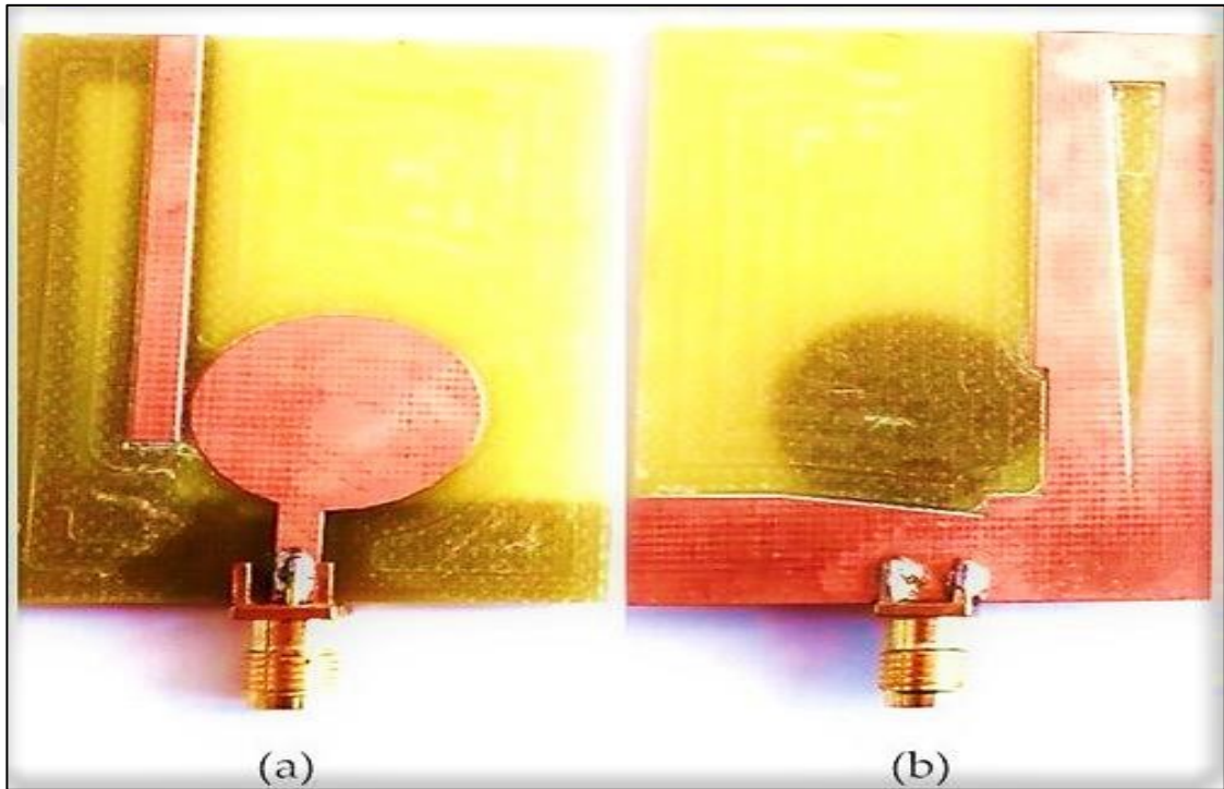
Şekil 3.9. Üretimi yapılan daireşel yamalı DMA'nın görüntüsü (a: Ön yüzü; b: Arka yüzü)
