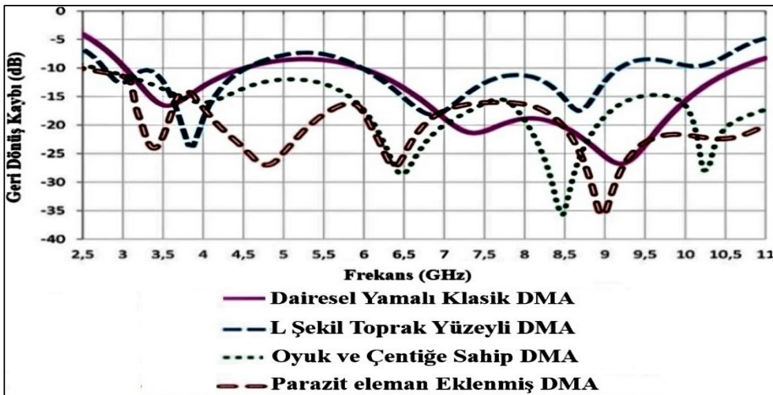
Şekil 3.6. Önerilen dairesel yamalı DMA'nın gelişimi boyunca benzetim ortamında elde edilen geri dönüş kayıpları
