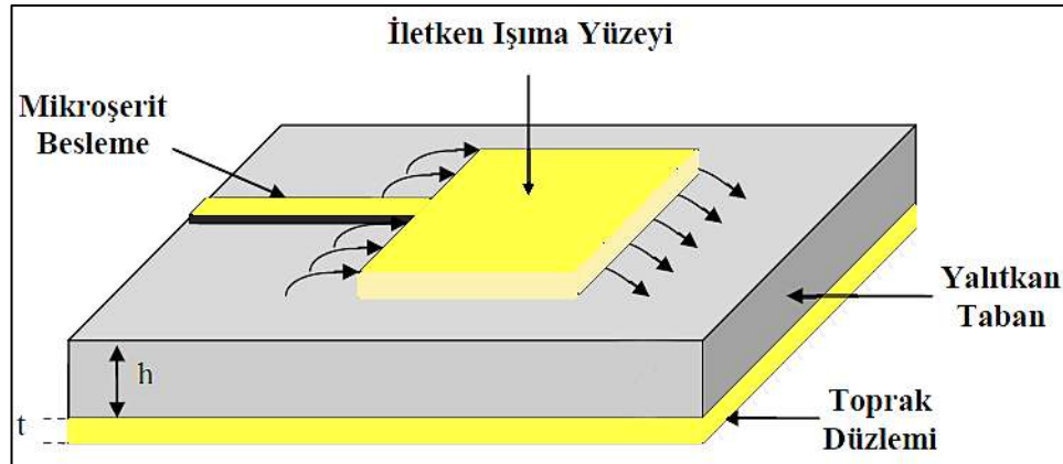
Şekil 3.2. Mikroşerit hat beslemeli bir MYA ve ısıma oluşumu
