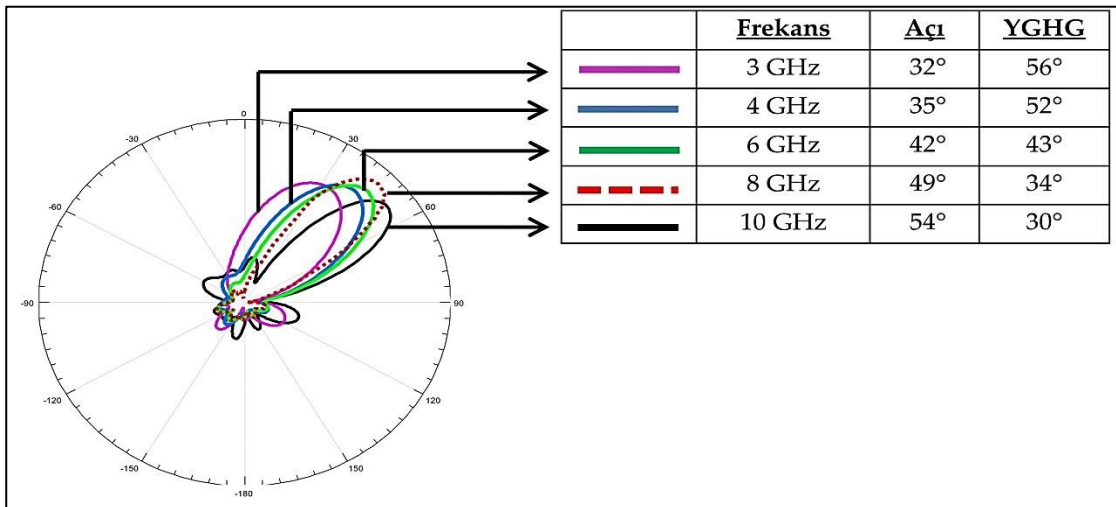
Şekil 3.11. Önerilen dairesel yamalı DMA'ya ait farklı frekanslardaki ışıma örüntüleri
