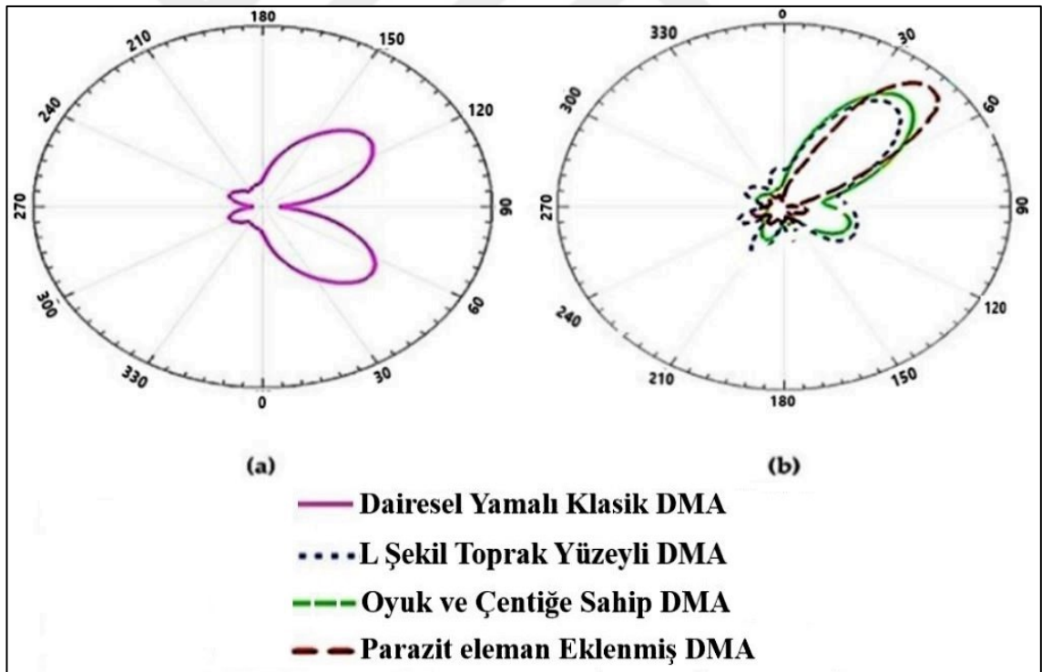
Şekil 3.7. Önerilen DMA’nın gelişimi boyunca benzetim ortamında 8 GHz frekansı için elde edilen ışıma örüntüleri (a: Dairesel yamalı klasik DMA için; b: Tasarım aşamalarıyla elde edilen DMA’lar için)
