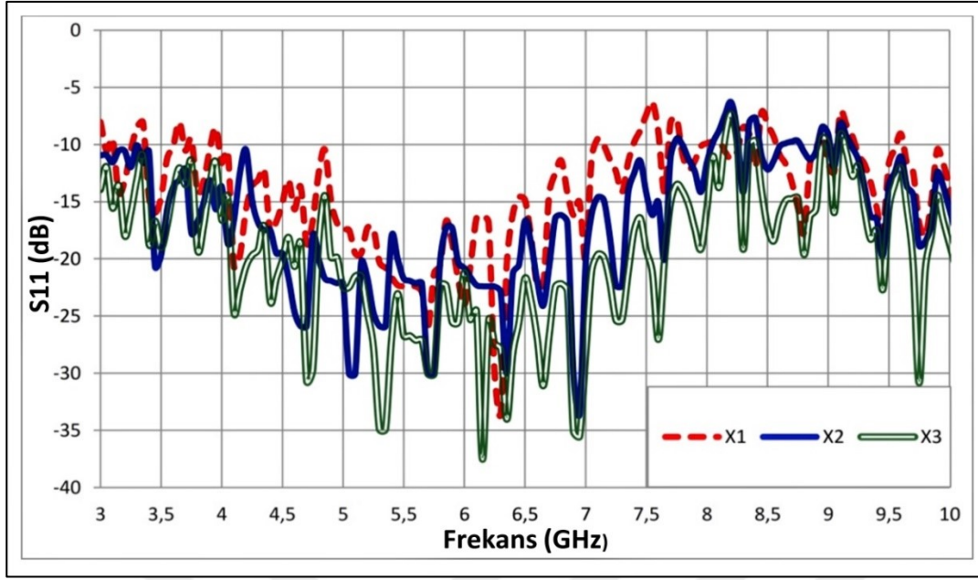
Şekil 4.4. Tümör merkezdeyken antenin farklı konumlardan elde ettiği S_{11} sonuçları
