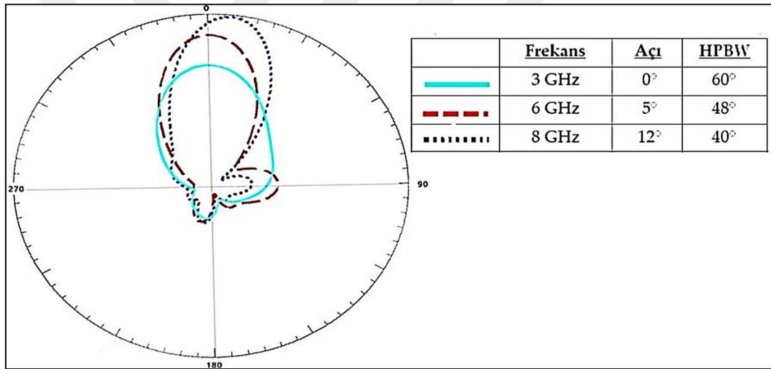
Şekil 3.19. Önerilen dörtgen yamalı DMA’ya ait farklı frekanslardaki ışıma örüntüleri
