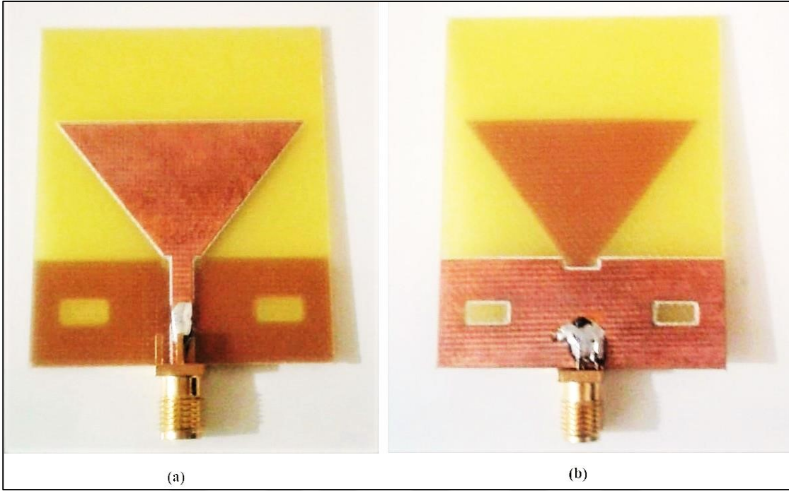
Şekil 3.17. Üretimi yapılan dörtgen yamalı antenin görüntüsü (a: Ön yüzü; b: Arka yüzü)
