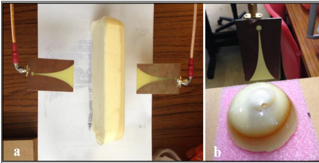
Şekil 2.5. Vivaldi antenlerle tümör tespiti için yapılan bazı ölçümler (Mohammad 2014)
