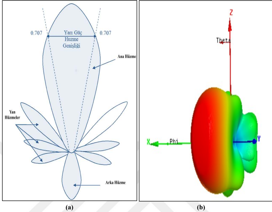
Şekil 1.13. Yönlü ışıma örüntüleri (a: İki boyutlu; b: Üç boyutlu)
