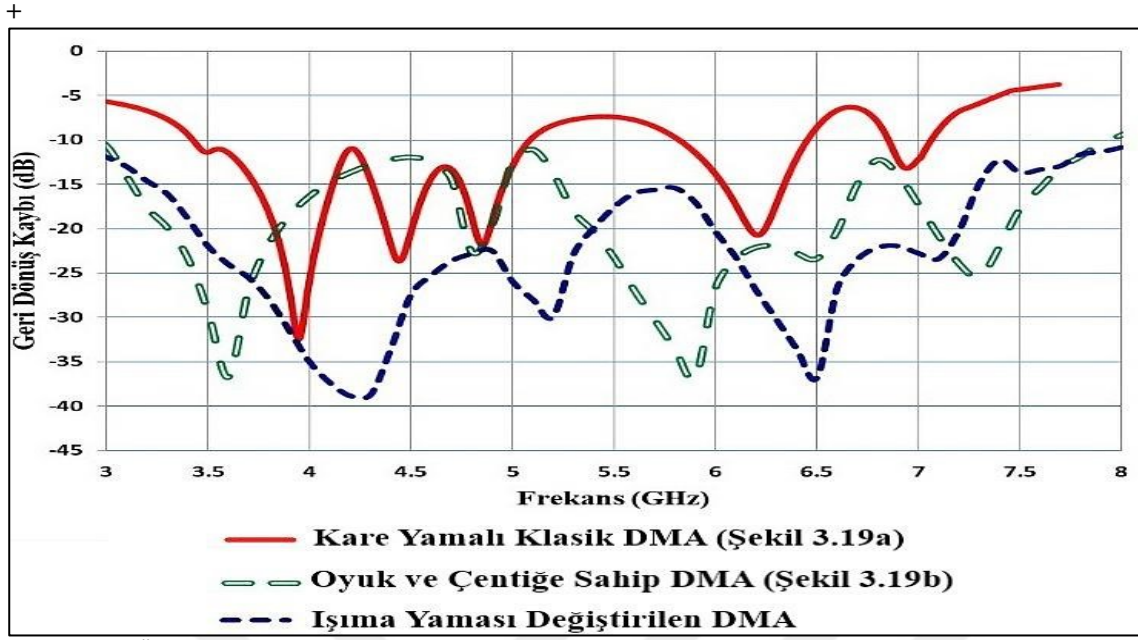
Şekil 3.14. Önerilen dörtgen yamalı DMA'nın gelişimi boyunca benzetim ortamında elde edilen geri dönüş kayıpları
