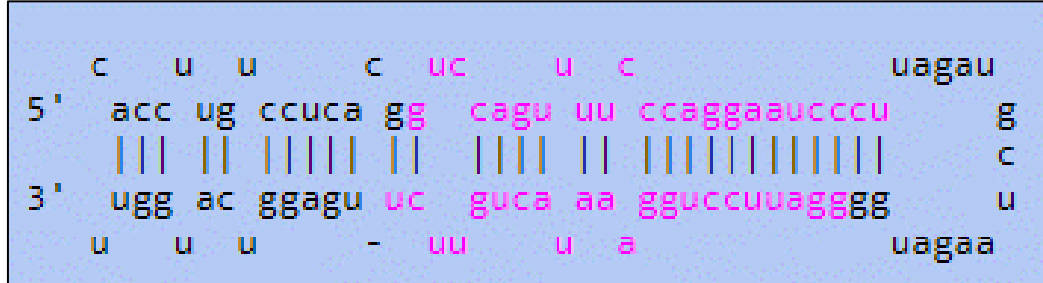
Şekil 2.12. miR-145 dizisi[161]
