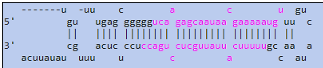
Şekil 2.15. miR-335 dizisi[171]
