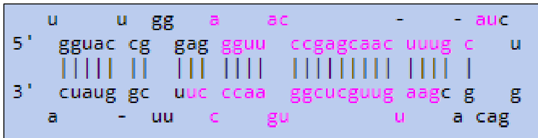
Şekil 2.19. miR-409 dizisi[180]
