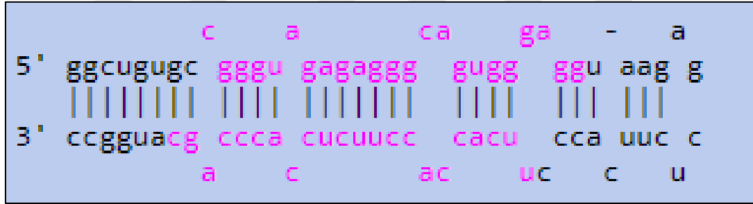
Şekil 2.20. miR-197 dizisi[182]
