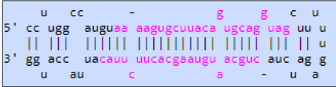
Şekil 2.16. miR-106a dizisi[174]
