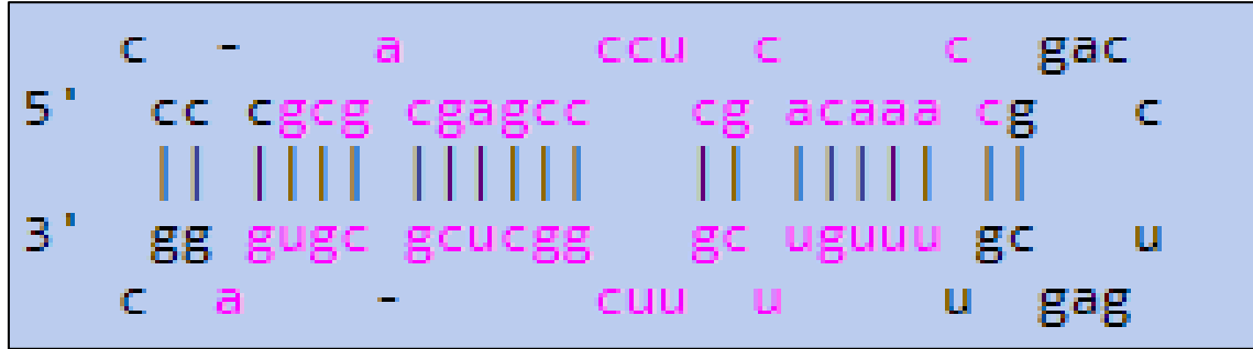
Şekil 2.18. miR-375 dizisi[179]
