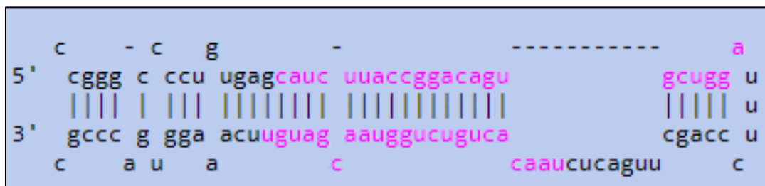
Şekil 2.14. miR-200a dizisi[168]
