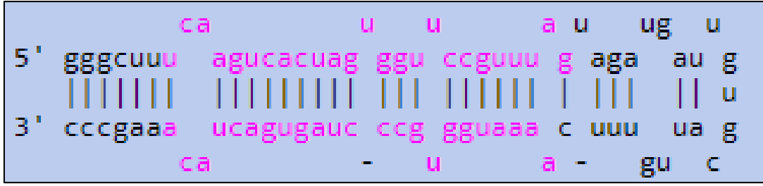
Şekil 2.21. miR-224 dizisi[184]
