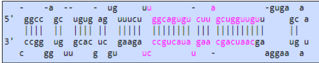
Şekil 2.13. miR-34a dizisi[166]
