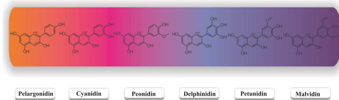
Şekil 2.4. Bazı antosiyanidinlerin kimyasal yapıları ve renkleri
