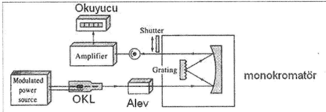
Şekil 8. Alevli Atomik Absorpsiyon spektrofotometresi
