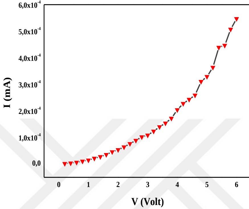
Şekil 4.17 Poli(IBMA)/ÇDKNT:%3 kompozitinin I-V grafiği
