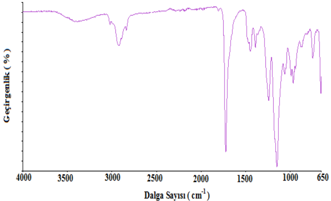
Şekil 4.2 Poli (CHMA)’nın FT-IR spektrumu
