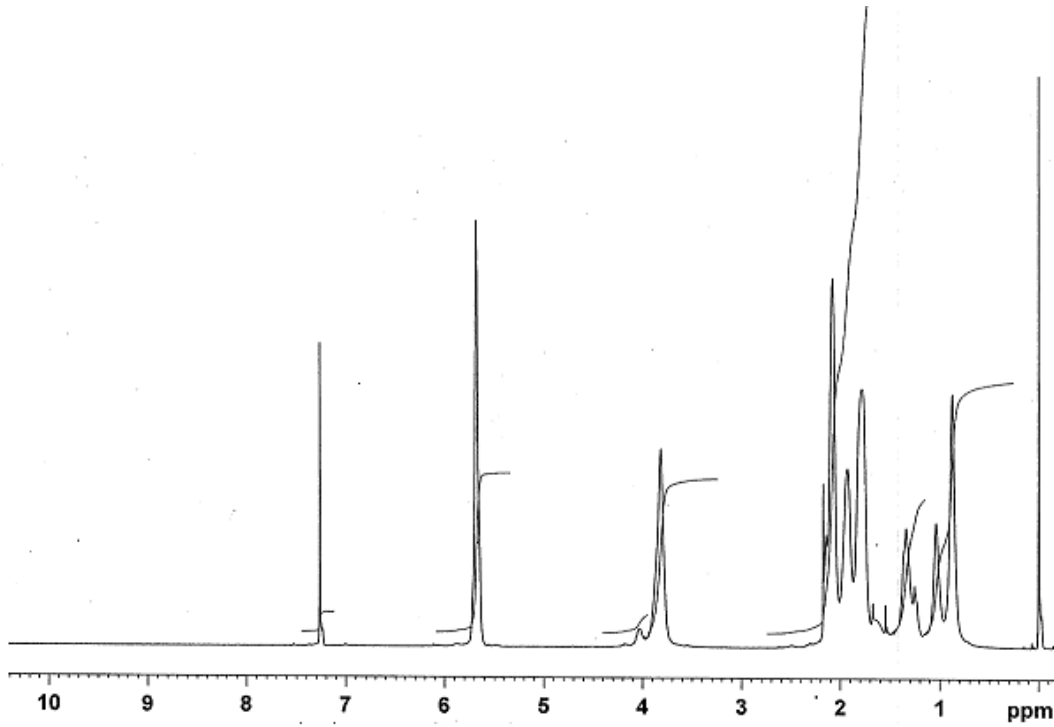
Şekil 4.3 Poli (CHMA)'nın ^1\text{H} -NMR spektrumu
