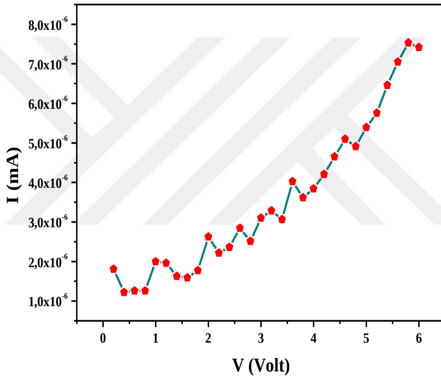
Şekil 4.14 Poli(CHMA)/ÇDKNT:%3 kompozitiinin I-V grafiği
