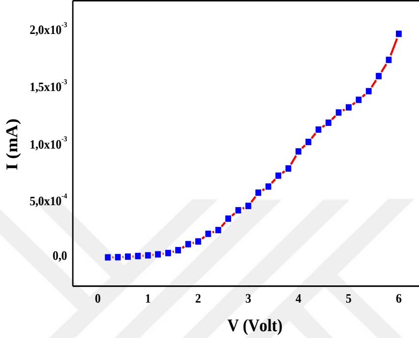
Şekil 4.15 Poli(CHMA)/ÇDKNT:%5 kompozitinin I-V grafiği
