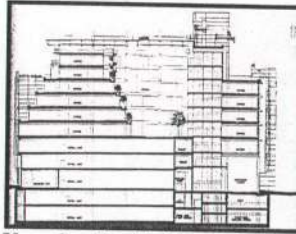
ŞEKİL 5.13 The Helicon Yapısı'nın Kesiti, (L'arç 149, p. 48).
