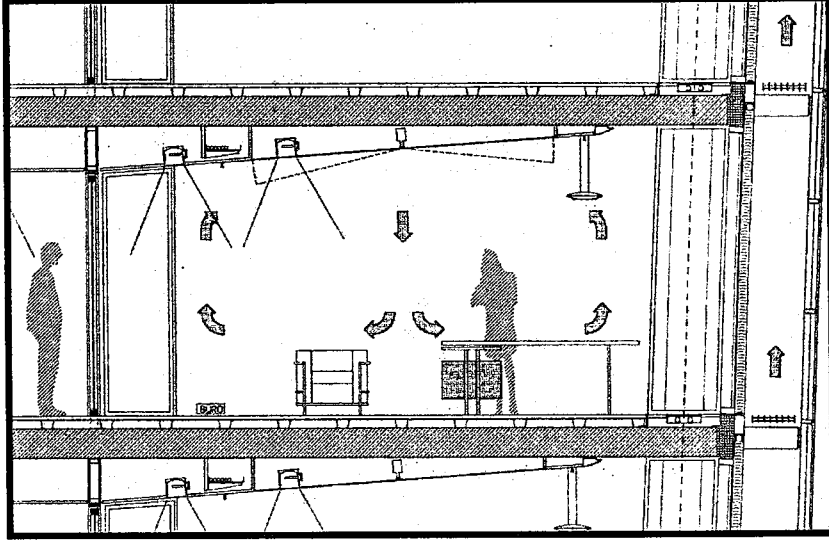
ŞEKİL 4.19 Hayat Sigorta Binası'nın Doğal Vantilasyon Şeması, (Compogno, 1999, p.123).
