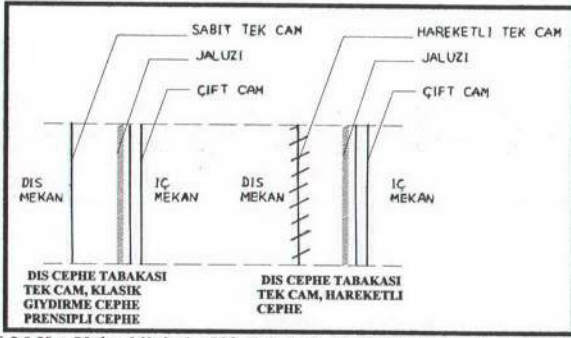
ŞEKİL 6.36 Kat Yüksekliğinde Çift Tabakalı Akıllı Giydirme Cephelerin Dış Cephe Tabakası Biçimlenmesi
