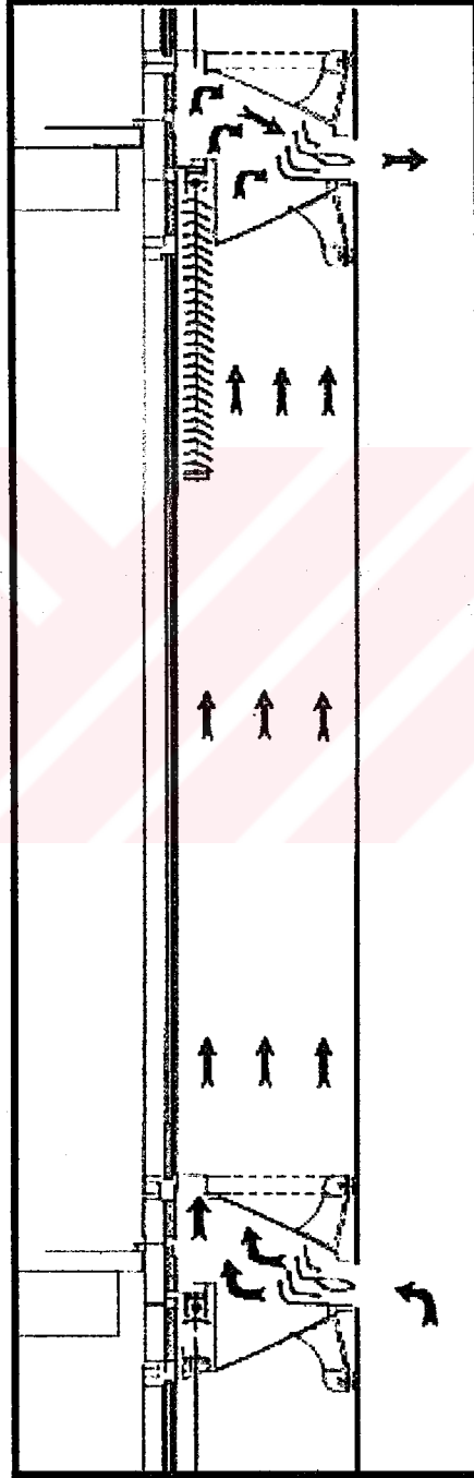
ŞEKİL 6.3 Çift Tabakalı Cephede Hava Akış Şeması, (Compagno, 1999, p.139).
