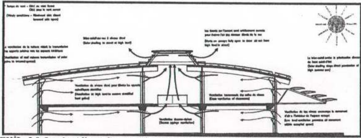
ŞEKİL 5.9 Lycée Albert Camus Binası'ndaki Doğal Ventilasyon, (Herzog, 1996, p.83).
