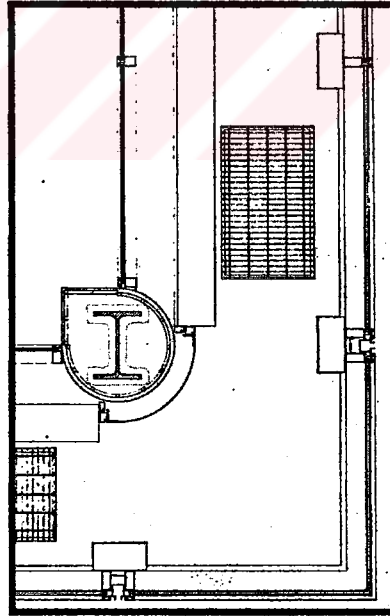
ŞEKİL 6.21 Occidental Chemical Centre Binası'nın Çift Tabakalı Giydirme Cephelerinin Planı, (Wigginton, 1996, p.161).
