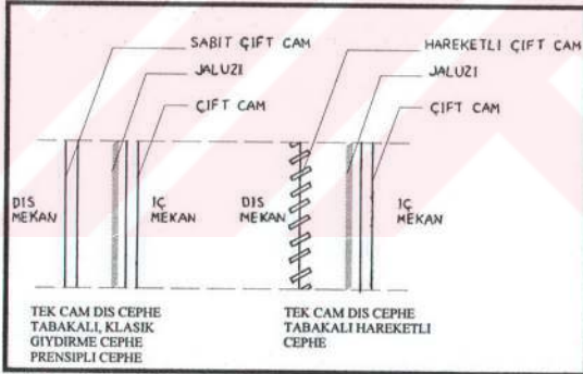
ŞEKİL 6.35 Kat Yüksekliğinde Çift Tabakalı Akıllı Giydirmce Cephelerin Dış Cephe Tabakası Biçimlenmesi
