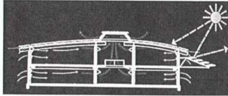
ŞEKİL 5.10 Lycée Albert Camus Binası'ndaki Doğal Ventilasyon, (Compagno, 1999, p.134).
