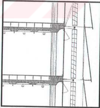
ŞEKİL 5.22 Deutsche Post Binası'nın Çift Tabakalı Giydirme Cephesi, (Compagno, 1999, p.153).
