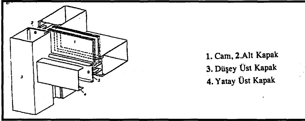
ŞEKİL 3.13 Monte Edilmiş Halde Giydirme Cephe Elemanları, (Schdmit, 1985).
