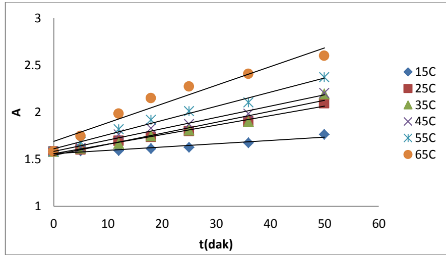
Şekil 3.20. Tetrafenilporfinatodemir(II) katalizölüğünde DMBA'nın sıcaklığa'a bağlı dönüşüm grafiği (8 mM VA, 0,8 M t- butilhidroperoksit, 10 mg polimer, t = 50 dak)
