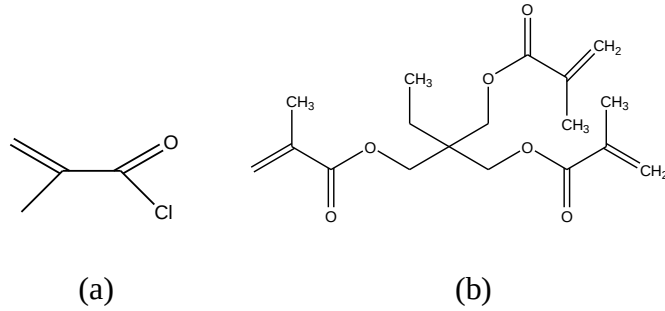
Şekil 3.1. a) Monomer metakrilil klorür (MA-Cl) b) Çapraz bağlayıcı trimetilolpropantrimetakrilatın (TMPTMA) yapısı
