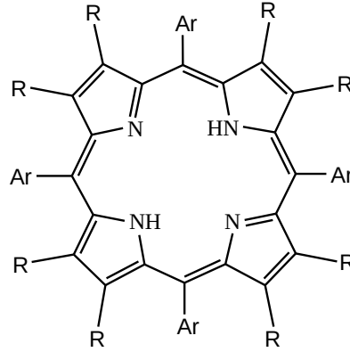
Şekil 1.4. Üçüncü kuşak porfirin ligantı örnekleri: H_2(TDCPBr_8P) : Ar= 2,6-diklorofenil, R= Br; H_2(TDCPCl_8P) : Ar= 2,6-diklorofenil, R= Cl; H_2(TDCPN_xP) : Ar= 2,6-diklorofenil, R= xNO_2 + (8-x)H ; H_2(TMPBr_8P) : Ar= 2, 4, 6- trimetilfenil, R= Br; H_2(TF_5PF_8P) : Ar= pentaflorofenil, R= F; H_2(TF_5PS_4P) : Ar= pentaflorofenil, R= 4SO_3H + 4H .
