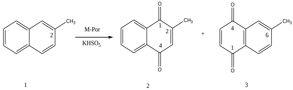
Şekil 1.11. 2-metilnaftalinin oksidasyon reaksiyonu
