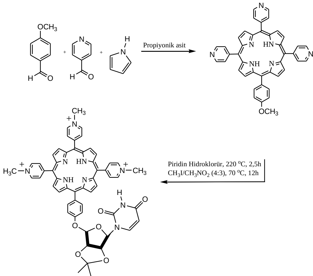
Şekil 1.7. Suda çözünebilen porfirin nükleositleri sentez reaksiyonu [28]
