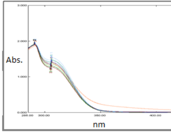
Şekil 2.1. Veratril alkolün veratril aldehite dönüşüm reaksiyonun UV-VIS spektrumu
