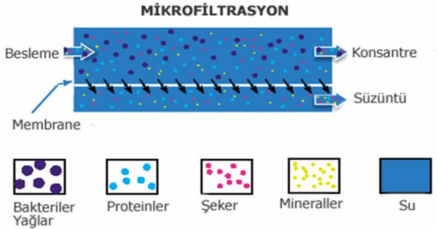
Şekil 4.5. Mikrofiltrasyon Prosesinin Şematik Gösterimi [46].
