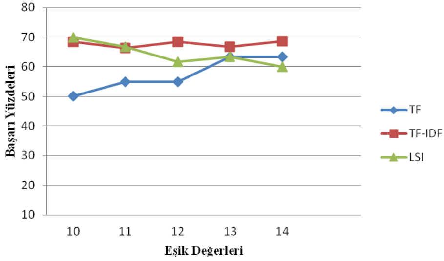
Şekil 5.7. TF, TF-IDF ve LSI vektörlerinin kıyaslanması
