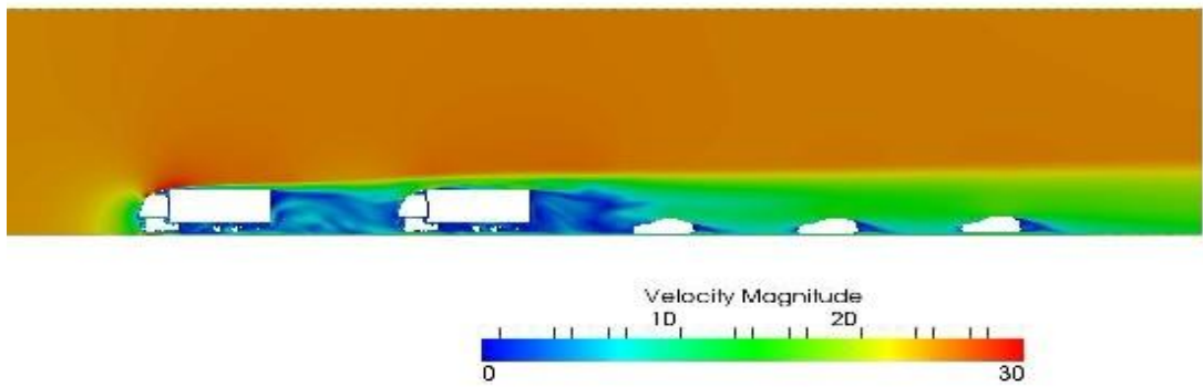
Şekil 10: 3, 6 ve 15 metrelik boşluklarda araçların Aero dinamik gösterimi [14]
