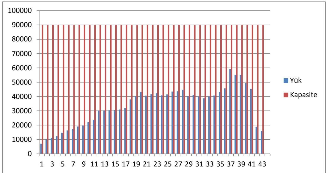
Şekil 37: Söğütluçeşme yönünden Beylikdüzü yönüne yük kapasite oranları
