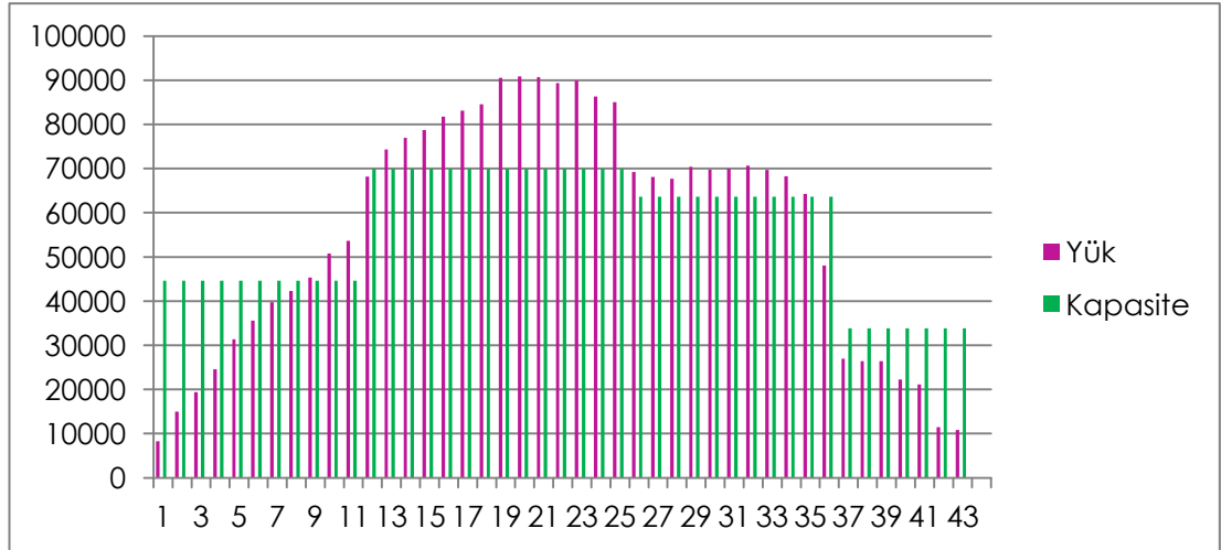
Şekil 28: Beylikdüzü yönünden Söğütluçeşme yönüne kapasite yük oranları
