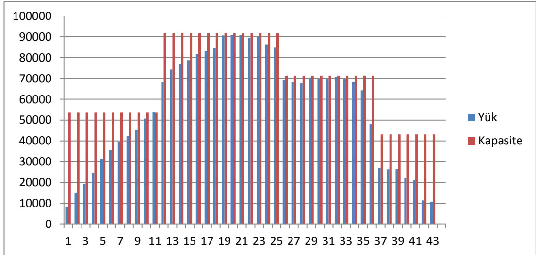
Şekil 41: Beylikdüzü yönünden Söğütluçeşme yönüne yük kapasite oranları
