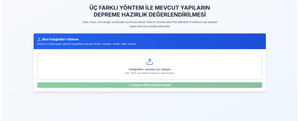
Şekil 5. Yazılımın arayüzü
