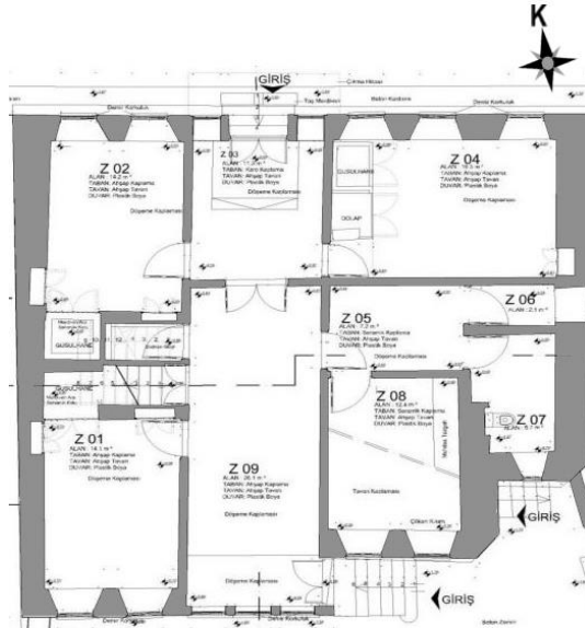
Şekil 4.19 Celal Sk. No:8 de bulunan yapının rölöve projesine ait zemin kat planı (Kudeb arşiv, 2022)
