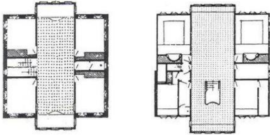
Şekil 3.12 Konya’da bulunan iç sofalı plan örnekleri (Eldem, 1984)
