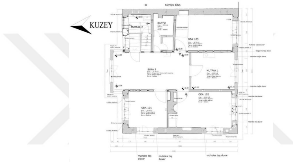
Şekil 4.26 Celal Sk. No:6 da bulunan yapının rölöve projesine ait birinci kat planı (Kudeb arşiv, 2019)
