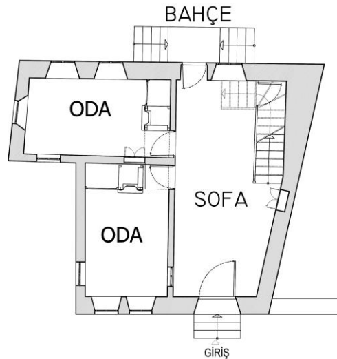
Şekil 4.73 Mahmut Dede Sk. No:20’de bulunan yapının restitüsyon projesine ait zemin kat planı (Argun Kocadağistan, 2022)
