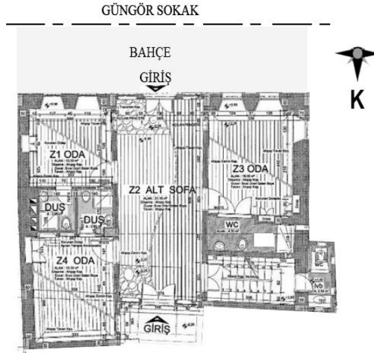
Şekil 4.50 Güngör sk. No:7’ de yer alan yapının zemin kat planı (Karatay Belediyesi arşiv, 2022)
