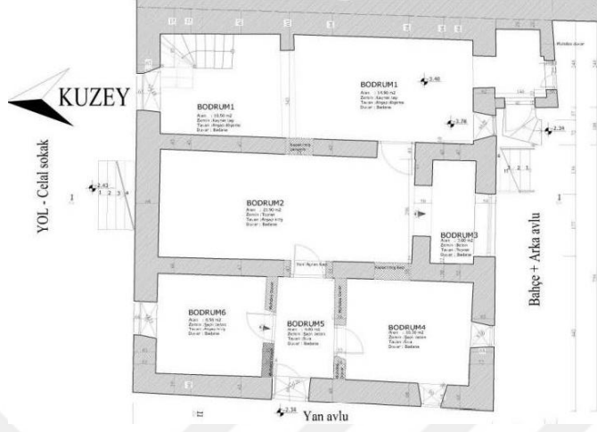
Şekil 4.27 Celal Sk. No:6 da bulunan yapının rölöve projesine ait bodrum kat planı (Kudeb arşiv, 2019)
