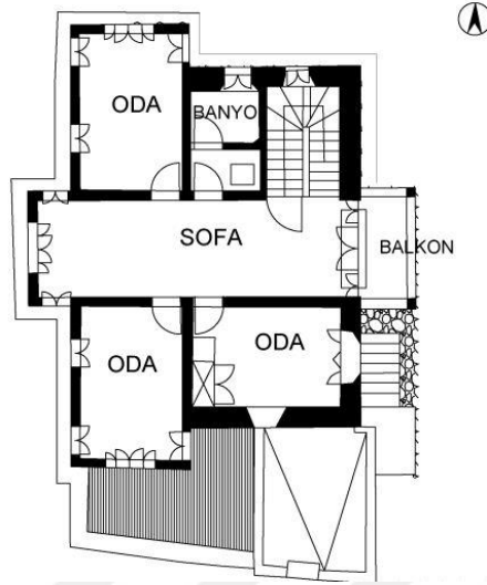
Şekil 4.56 Mahmut Dede Sk. No:25'te bulunan yapının birinci kat planı, Rölöve: Mine Ulusoy (Dönmez, 2017)
