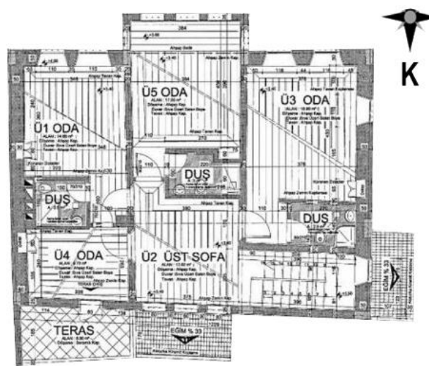
Şekil 4.51 Güngör sk. No:7’ de yer alan yapının birinci kat planı (Karatay Belediyesi arşiv, 2022)
