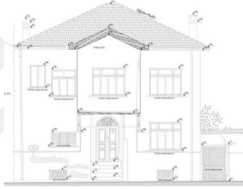
Şekil 4.30 Celal Sk. No:6 da bulunan yapının rölöve çizimlerine ait Kuzey cephesi (Kudeb arşiv, 2022)
