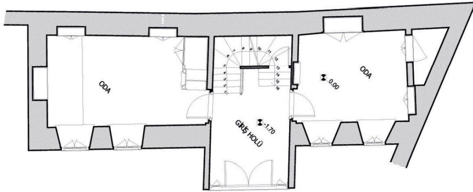
Şekil 4.40 Sokullu Mehmet Paşa Sk. No:14'te bulunan yapıya ait zemin kat planı, Rölöve: Ramazan Demir
