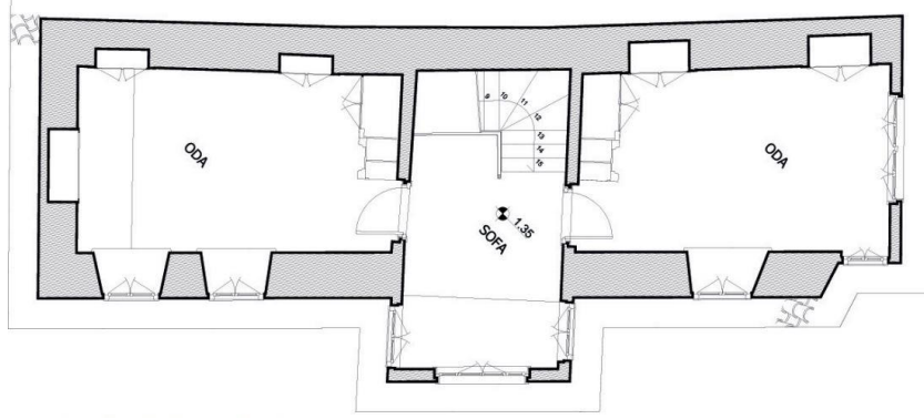
Şekil 4.41 Sokullu Mehmet Paşa Sk. No:14'te bulunan yapıya ait birinci kat planı, Rölöve: Ramazan Demir
