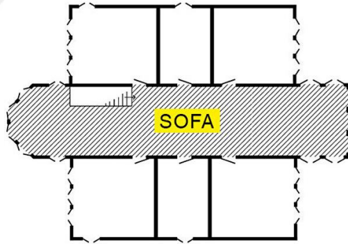
Şekil 3.11 İç sofalı plan tipini gösteren şematik plan (Url 3)
