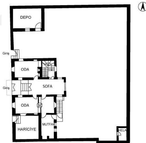
Şekil 4.55 Mahmut Dede Sk. No:25'te bulunan yapının Zemin kat planı, Rölöve: Mine Ulusoy (Dönmez, 2017)
