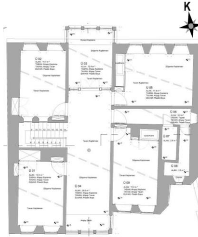
Şekil 4.20 Celal Sk. No:8 de bulunan yapının rölöve projesine ait birinci kat planı (Kudeb arşiv, 2022)
