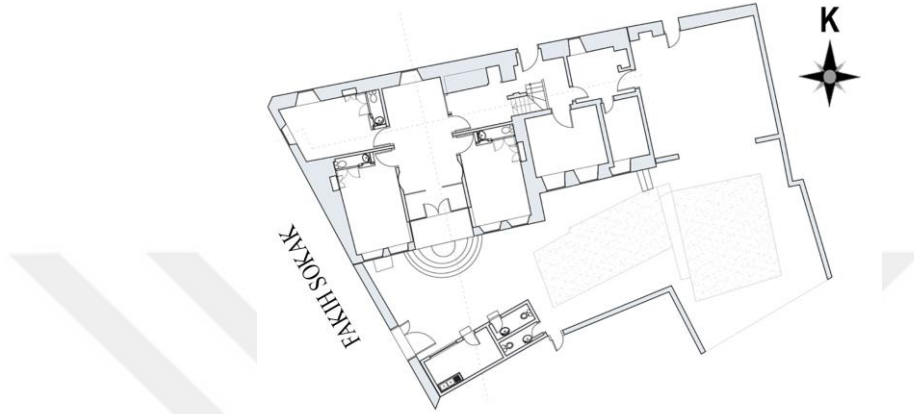
Şekil 4.5 Fakih sk. No:26'da bulunan yapının zemin kat planı (Rölöve, Argun Kocadağistan)
