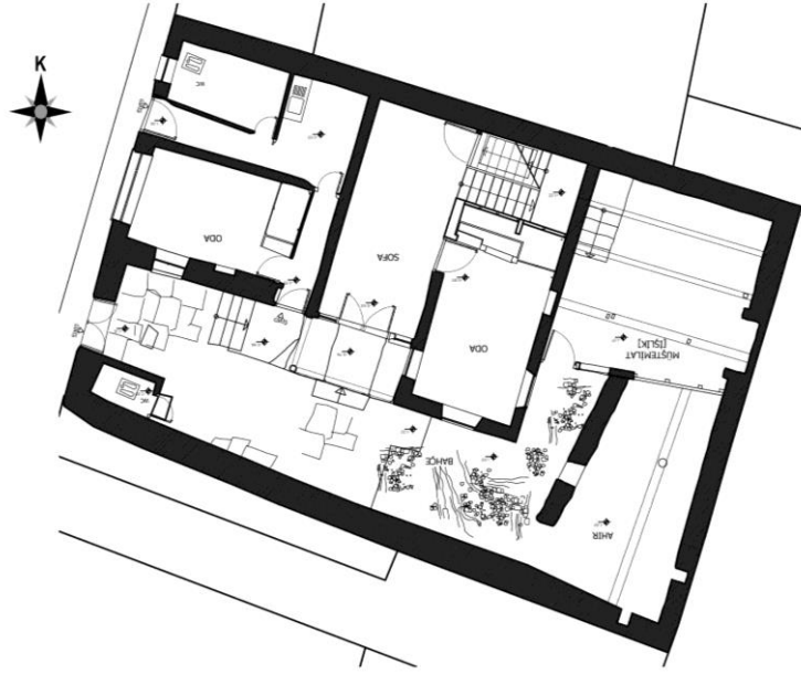
Şekil 4.65 Mahmut Dede Sk. No:21’de yer alan yapının rölöve projesine ait zemin kat planı (Rölöve: Ramazan Demir, 2008)
