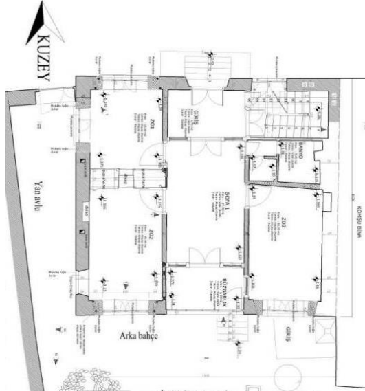
Şekil 4.25 Celal Sk. No:6 da bulunan yapının zemin kat rölöve projesine ait planı (Kudeb arşiv, 2019)
