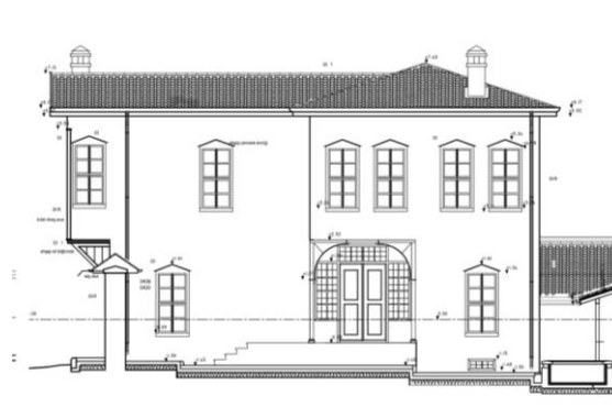
Şekil 4.69 Mahmut Dede Sk. No:21’de yer alan yapının restorasyon projesine ait, bahçe cephesi(Rölöve: Ramazan Demir, 2008)
