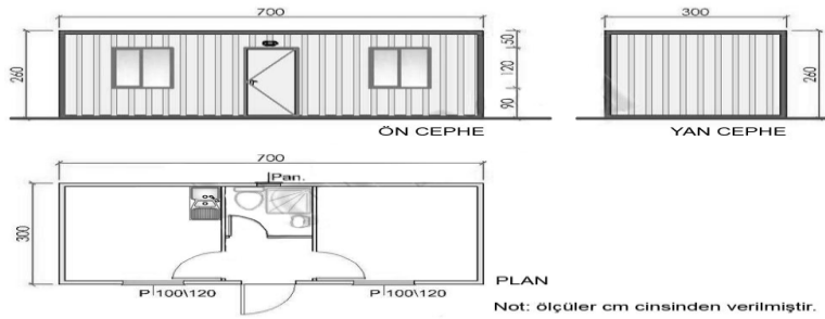
Şekil 2.9 : Geçici afet konutu planı (Ünal, 2013).
