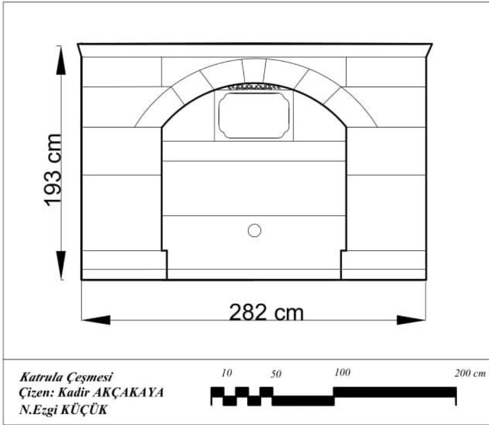
Şekil 4.63. Katrula Çeşmesi cephe çizimi
