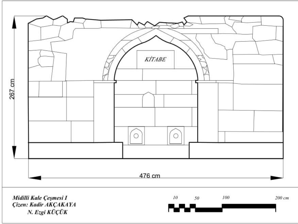
Şekil 4.79. Midilli Kale Çeşmesi 1 cephe çizimi
