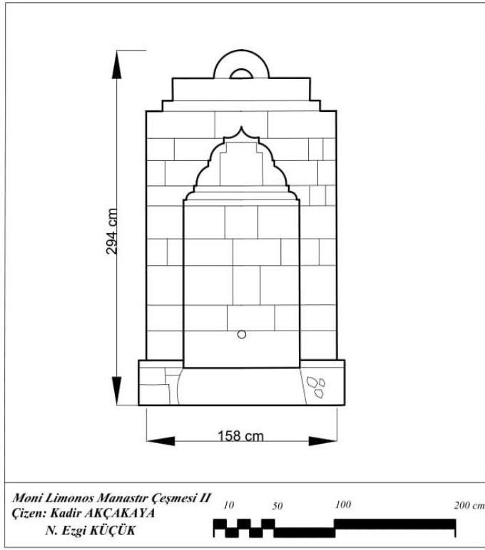
Şekil 4.133. Moni Limonos Manastır Çeşmesi 2 cephe çizimi
