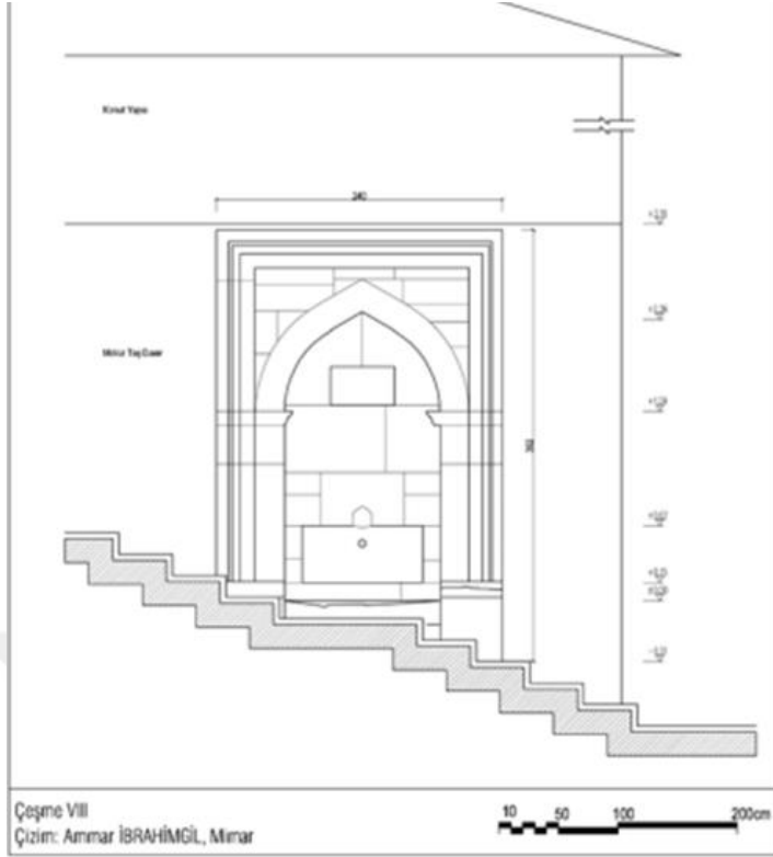
Şekil 4.112. Molivos Kasabası Çeşme 4 cephe çizimi 158
