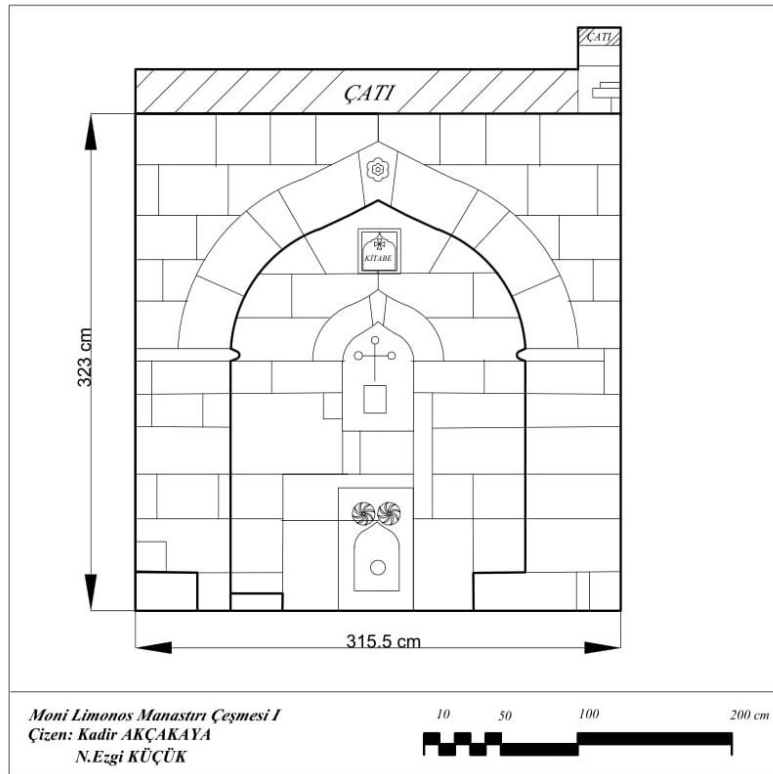
Şekil 4.127. Moni Limonos Manastırı Çeşmesi 1 cephe çizimi
