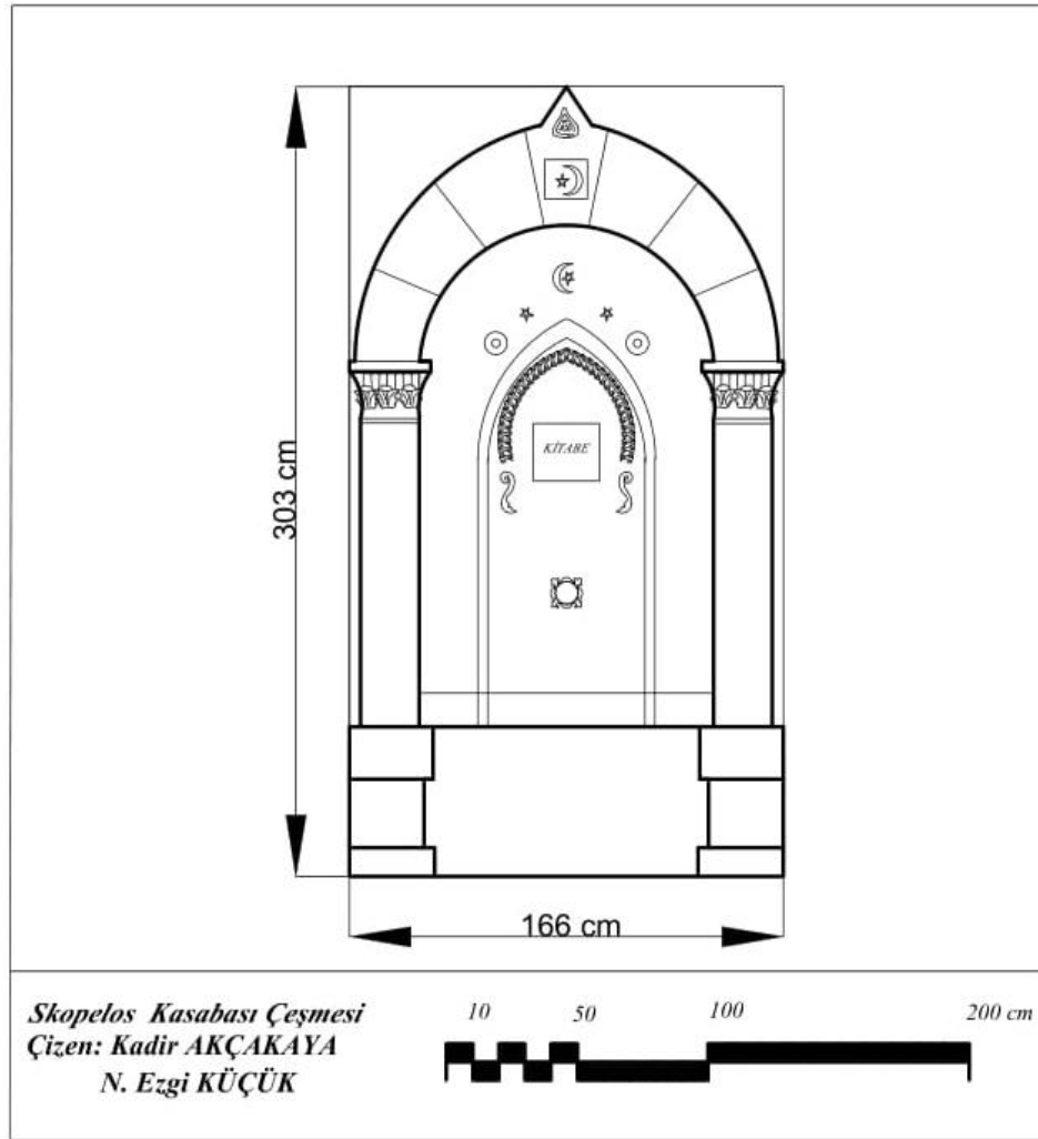
Şekil 4.173. Skopelos Kasabası Çeşmesi cephe çizimi
