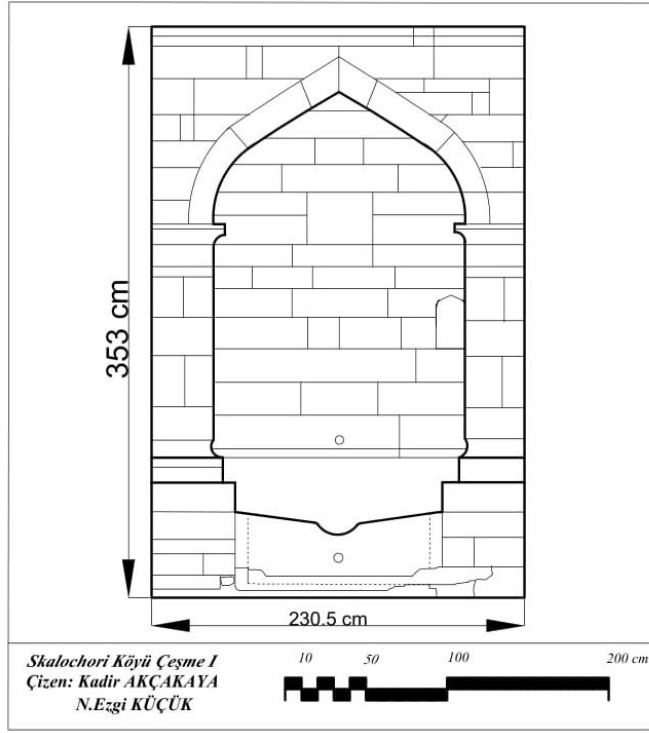
Şekil 4.161. Skalochoori Köyü Çeşme 1 cephe çizimi
