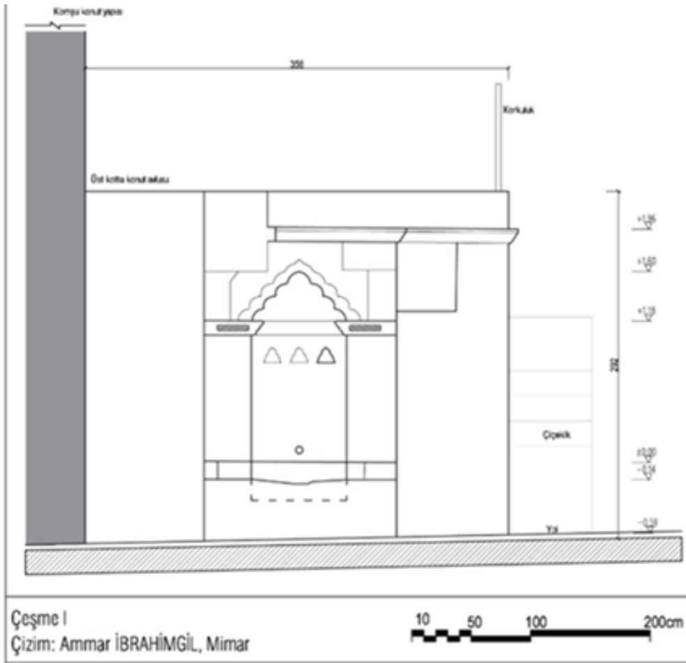
Şekil 4.97. Molivos Kasabası Çeşme 1 cephe çizimi 152
