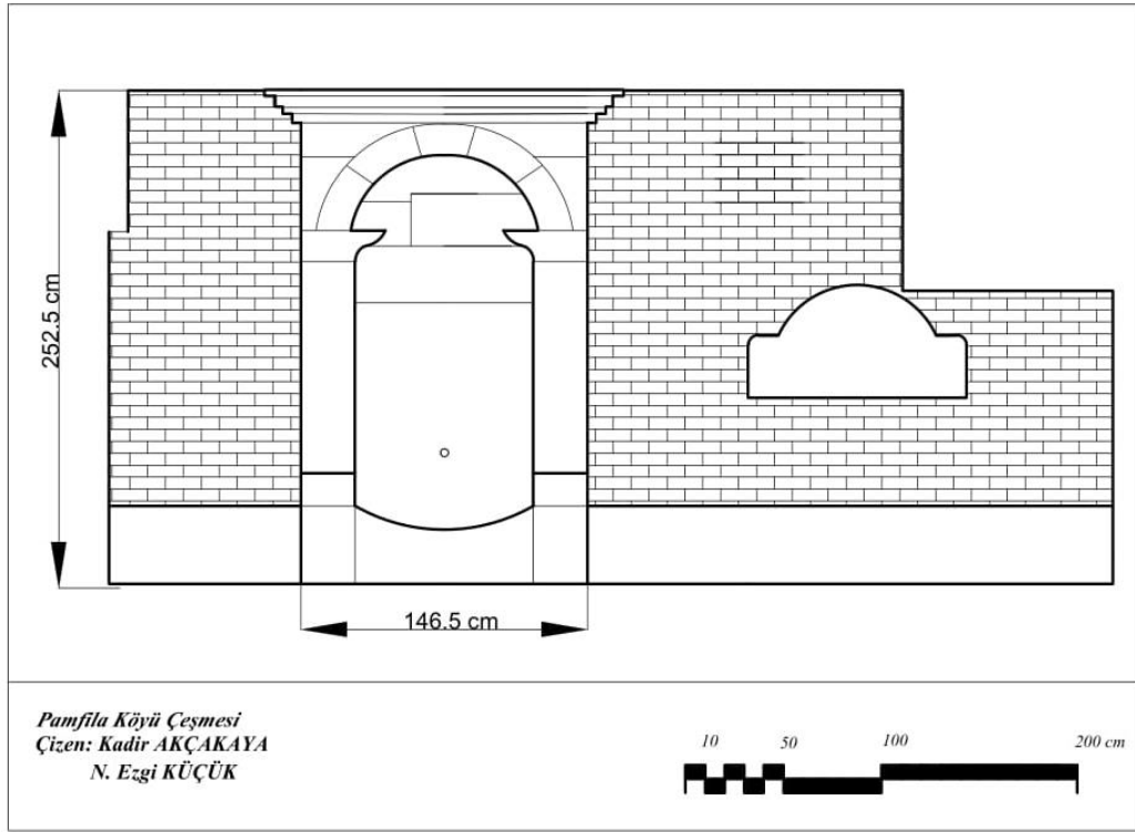
Şekil 4.140. Pamfili Köyü Çeşmesi cephe çizimi
