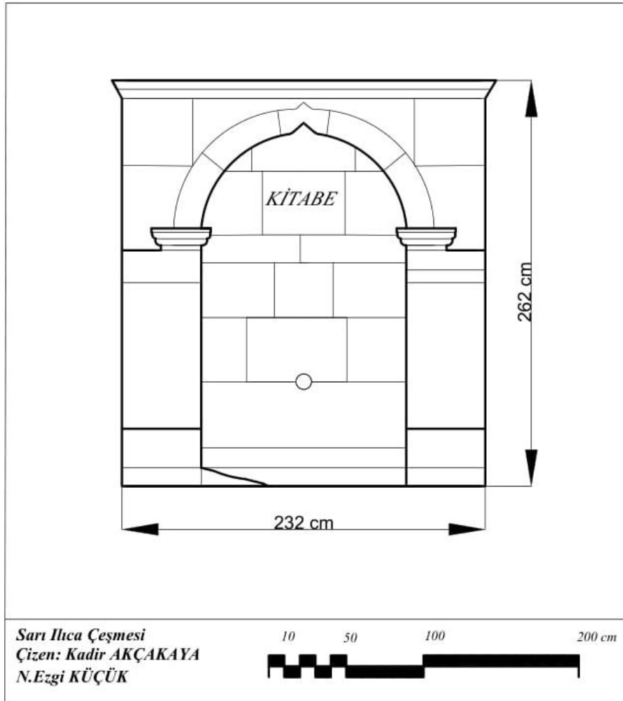
Şekil 4.153. Sarı Ilıca Çeşmesi cephe çizimi
