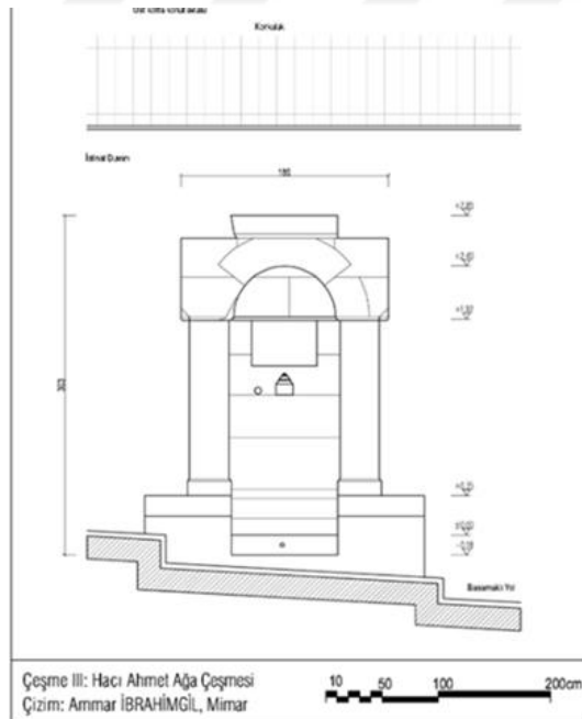
Şekil 4.39. Hacı Ahmet Ağa Çeşmesi cephe çizimi 132
