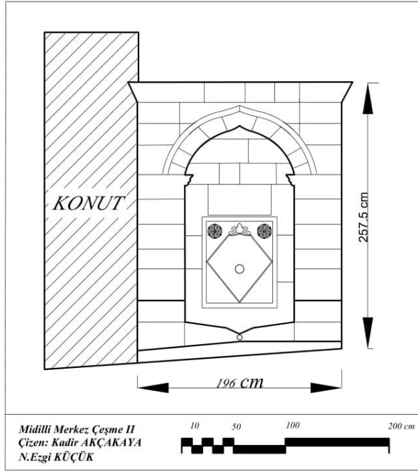
Şekil 4.92. Midilli Merkez Çeşme 2 cephe çizimi
