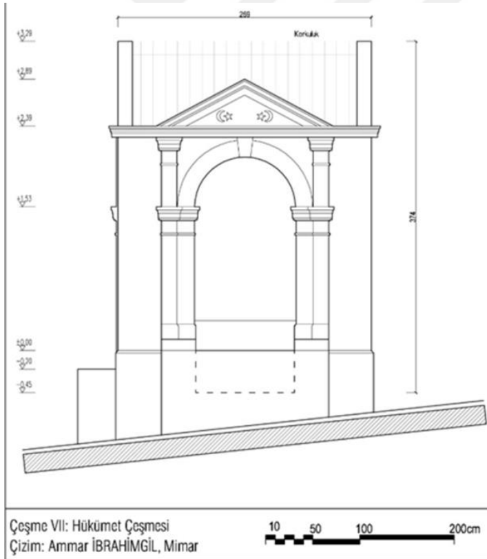
Şekil 4.57. Hükümet Çeşmesi cephe çizimi 138
