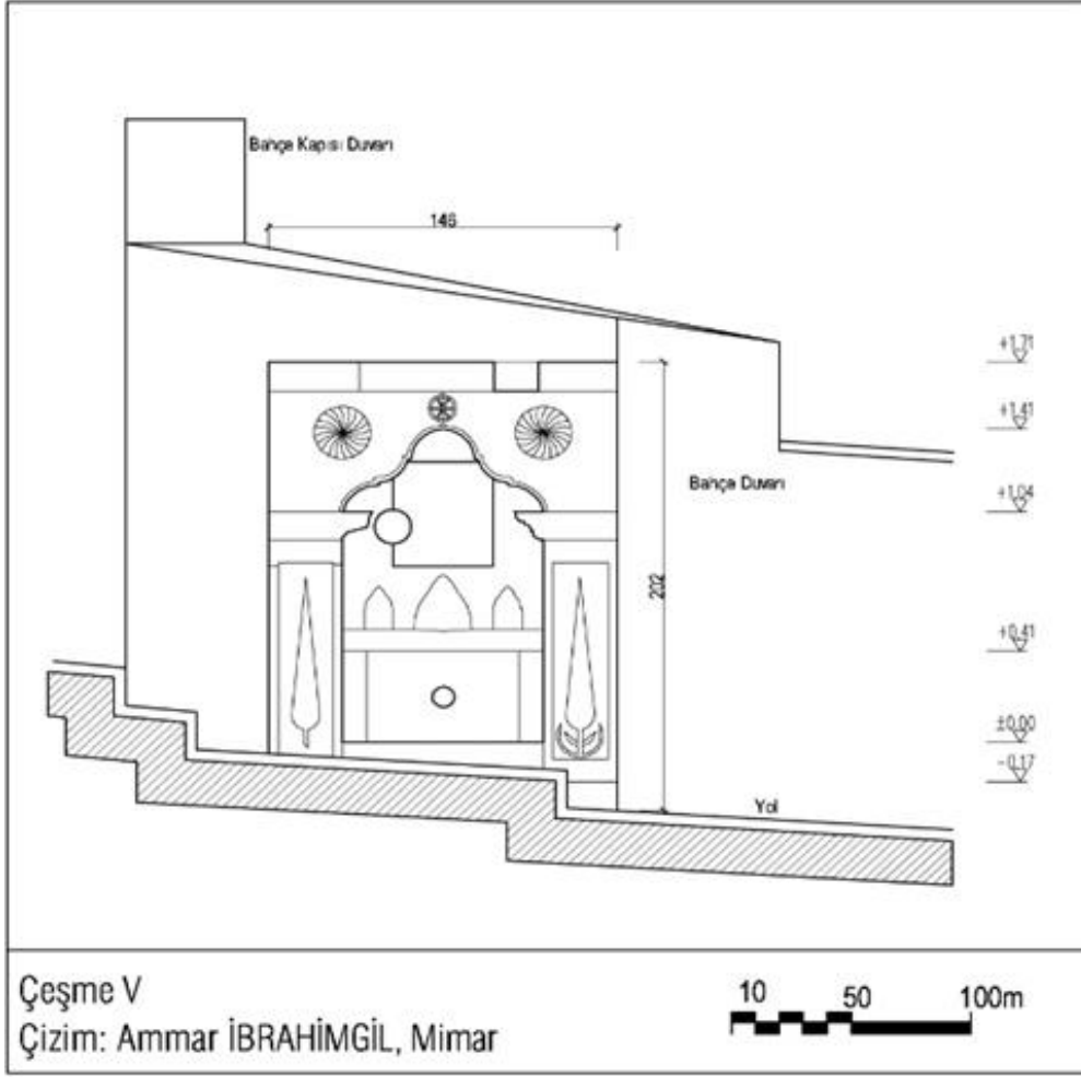
Şekil 4.104. Molivos Kasabası Çeşme 2 cephe çizimi 154
