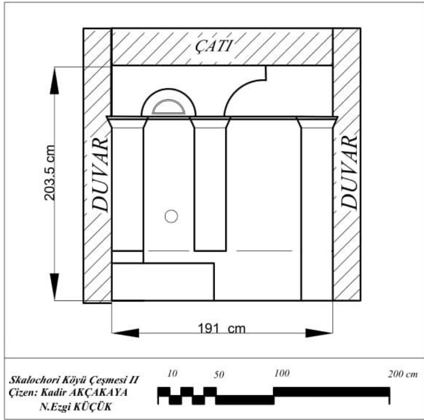
Şekil 4.165. Skalochoori Köyü Çeşme 2 cephe çizimi
