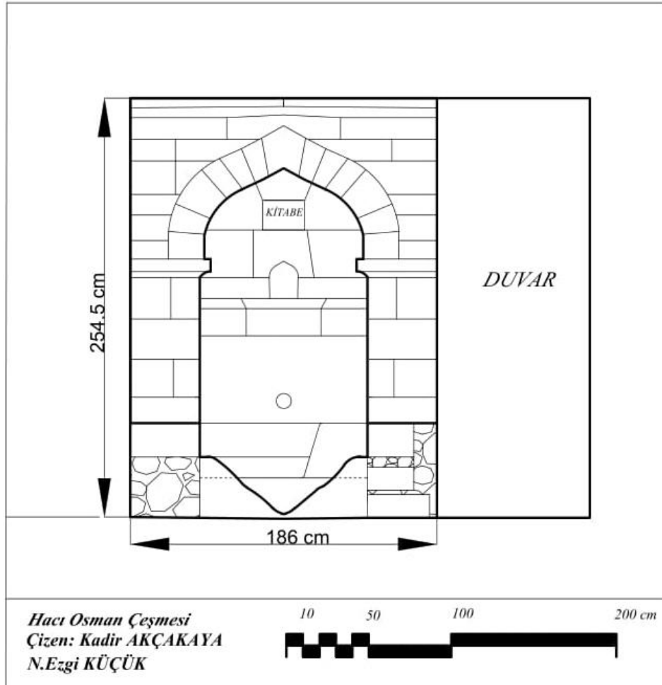
Şekil 4.53. Hacı Osman Çeşmesi cephe çizimi
