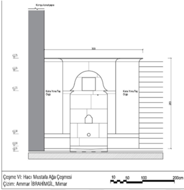
Şekil 4.49. Hacı Mustafa Ağa Çeşmesi cephe çizimi 137
