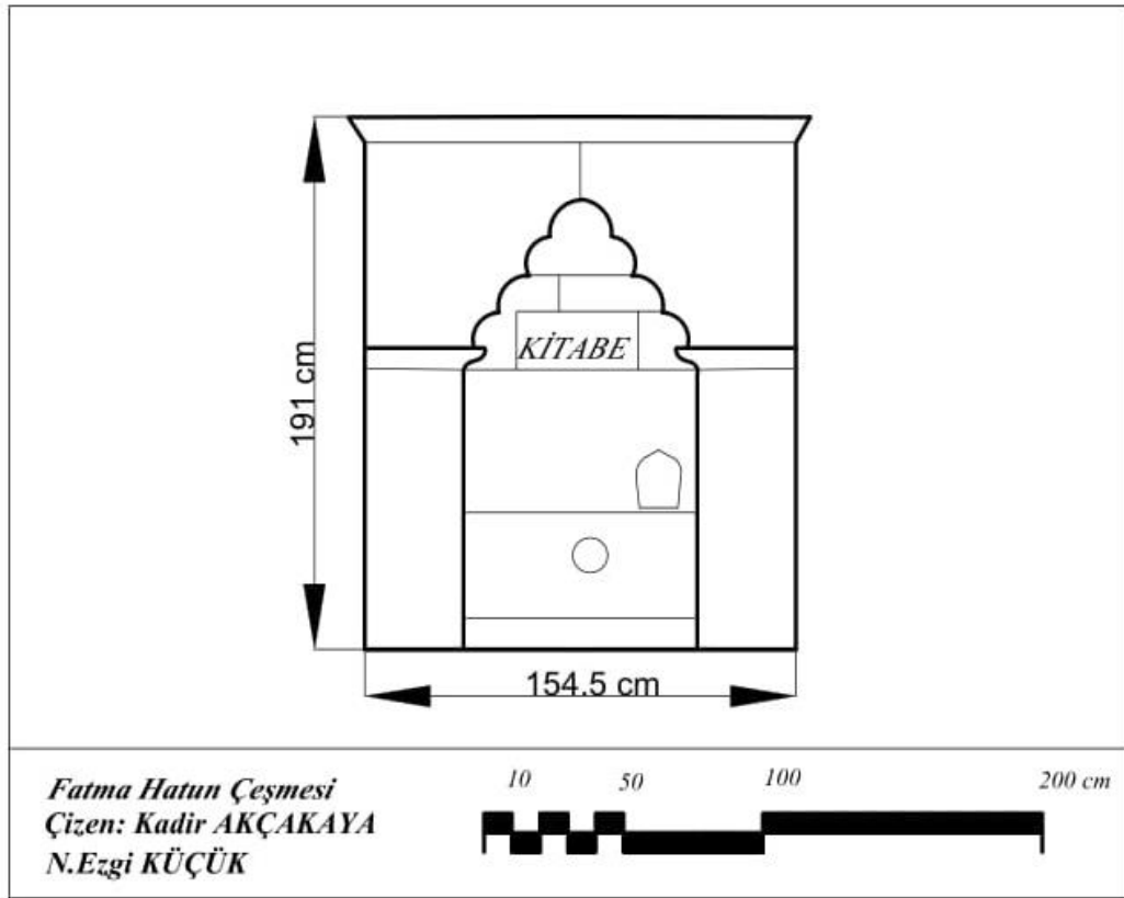
Şekil 4.35. Fatma Hatun Çeşmesi cephe çizimi
