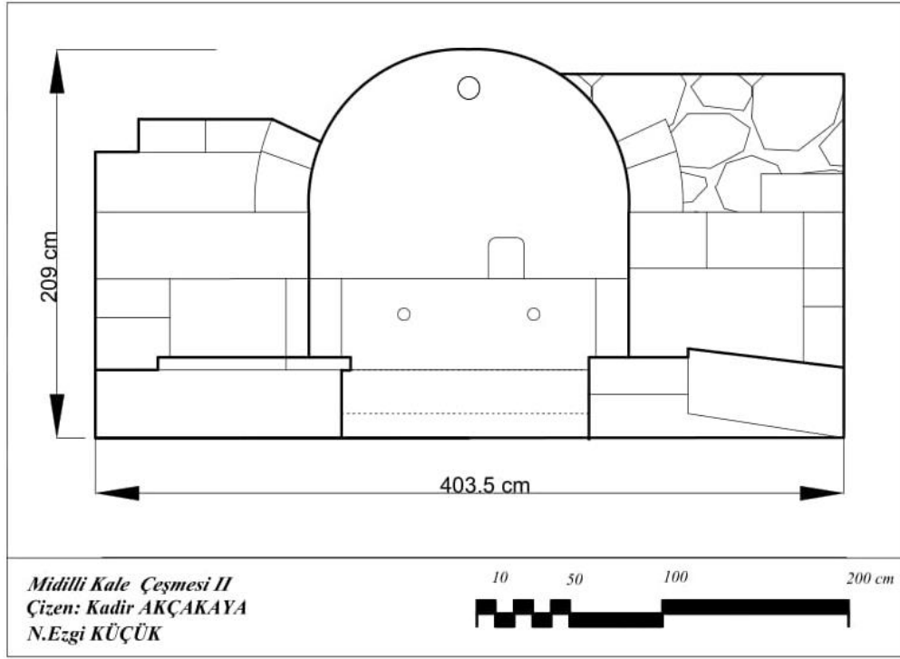
Şekil 4.86. Midilli Kale Çeşmesi 2 cephe çizimi
