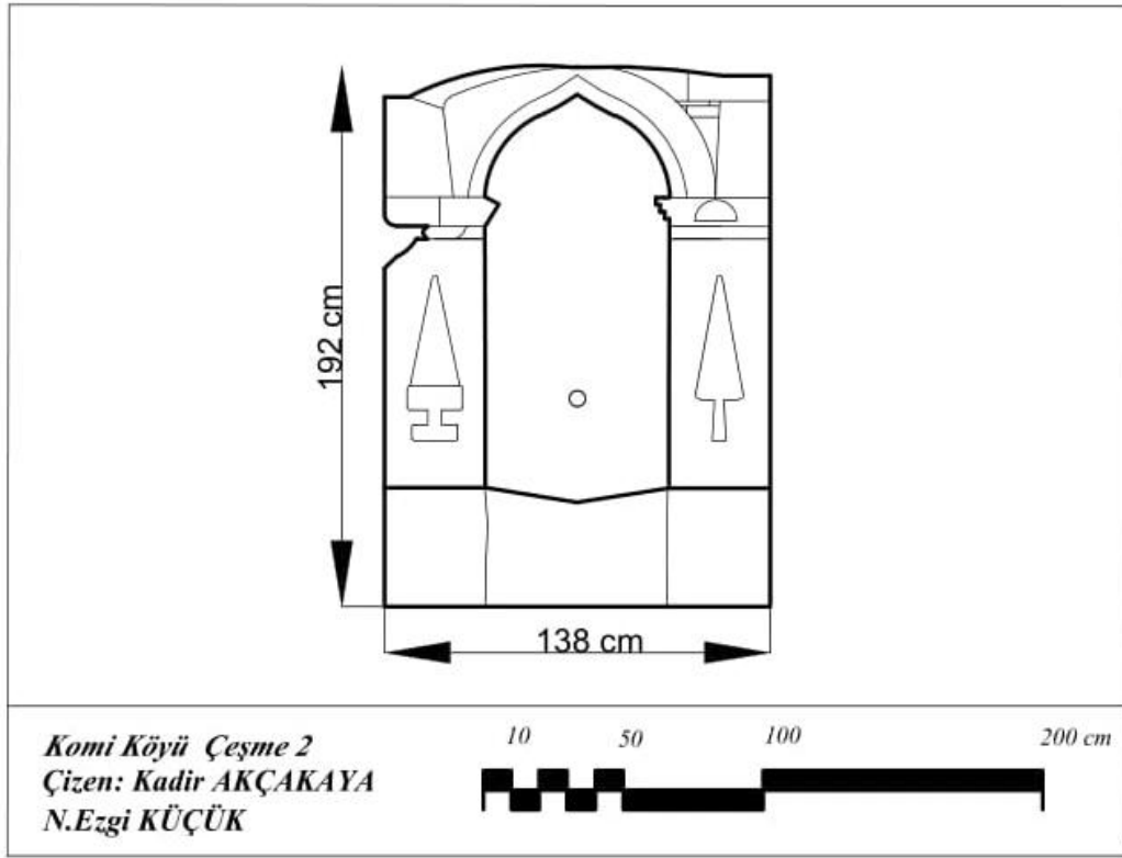
Şekil 4.70. Komi Köyü Çeşme 2 cephe çizimi
