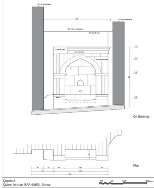
Şekil 4.115. Molivos Kasabası Çeşme 5 cephe çizimi 161
