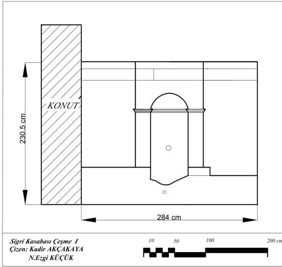
Şekil 4.158. Sıgri Kasabası Çeşme 1 cephe çizimi
