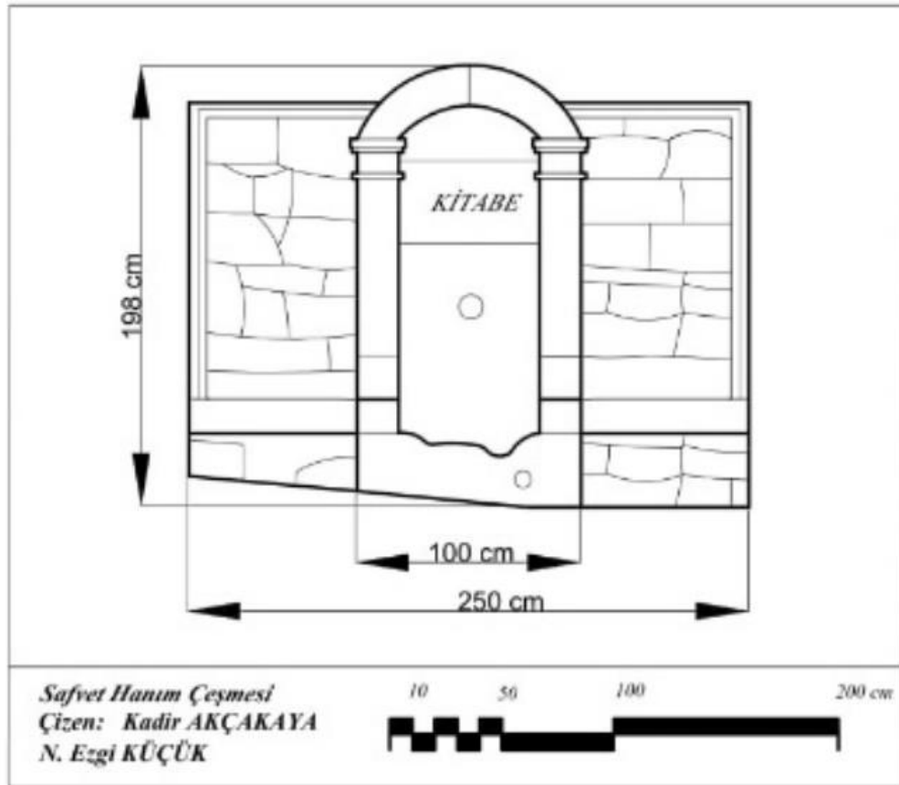
Şekil 4.149. Safvet Hanım Çeşmesi cephe çizimi
