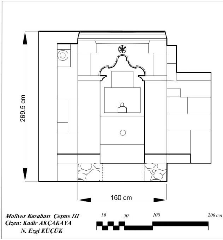
Şekil 4.108. Molivos Kasabası Çeşme 3 cephe çizimi
