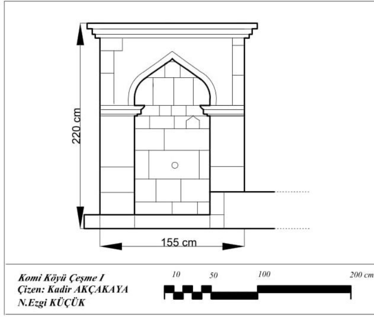
Şekil 4.66. Komi Köyü Çeşme 1 cephe çizimi
