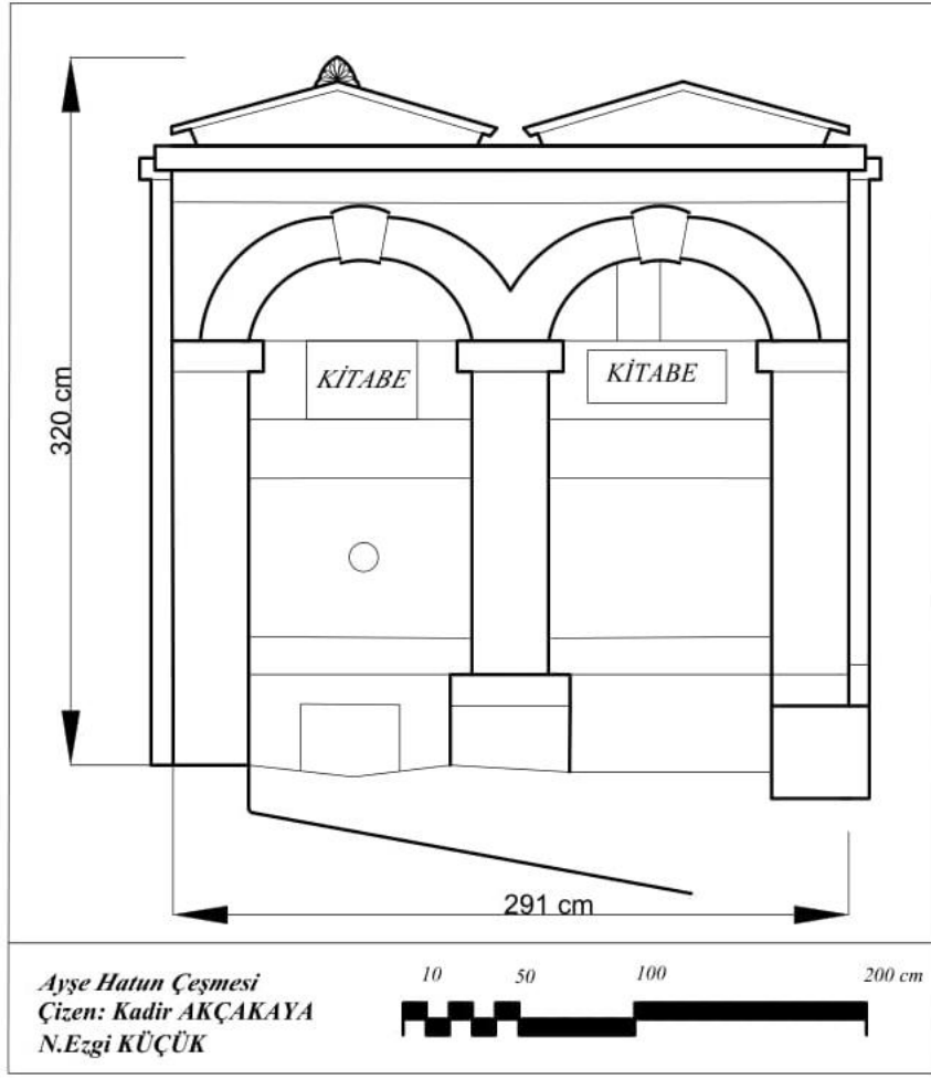
Şekil 4.13. Ayşe Hatun Çeşmesi cephe çizimi
