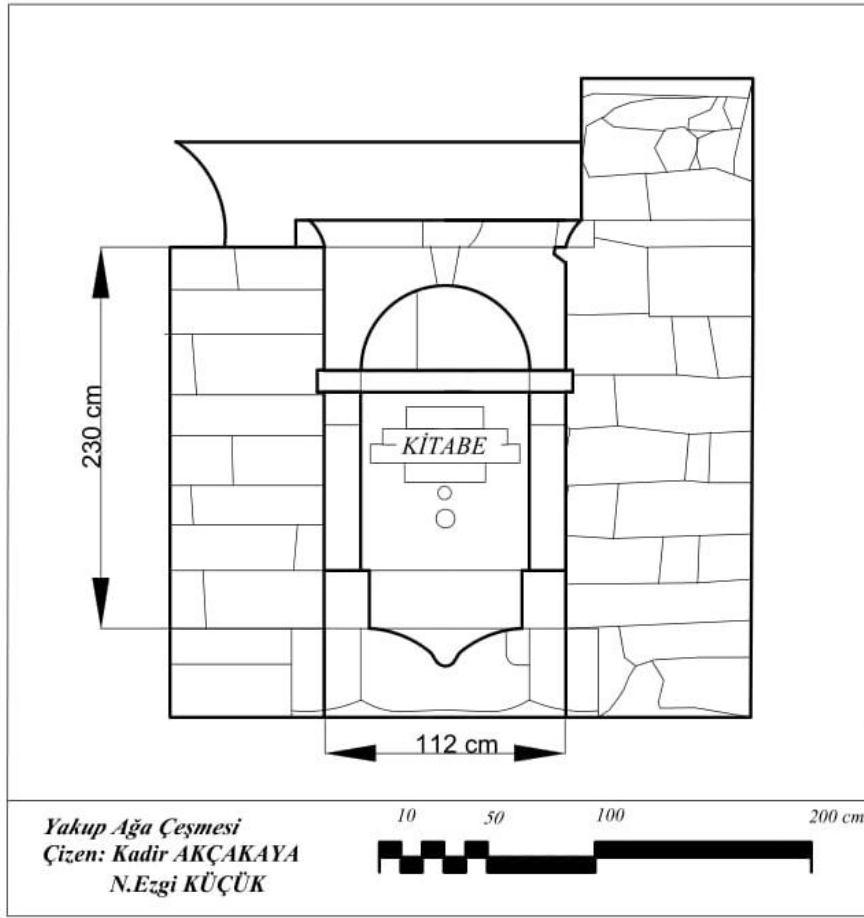
Şekil 4.187. Yakup Ağa Çeşmesi cephe çizimi
