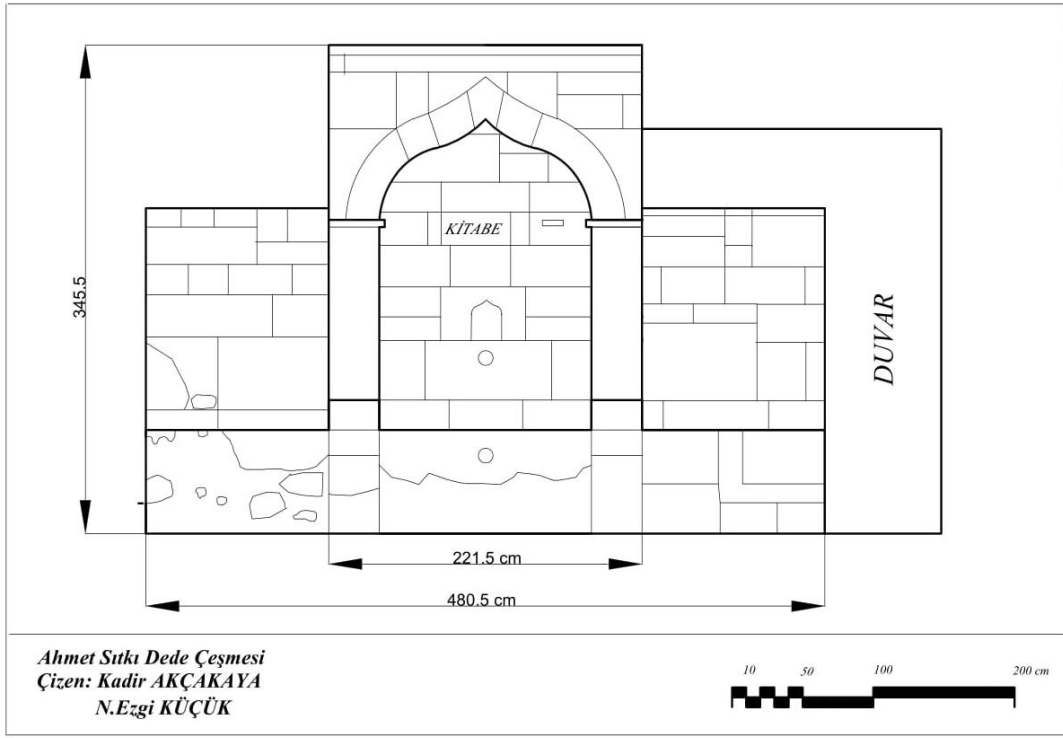
Şekil 4.3. Ahmet Sıtkı Dede Çeşmesi cephe çizimi
