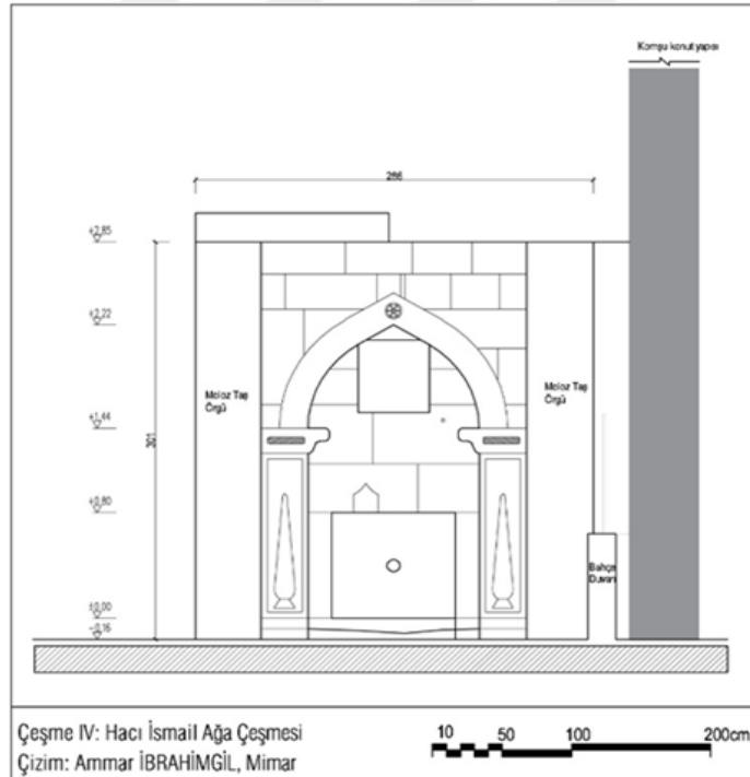
Şekil 4.44. Hacı İsmail Ağa Çeşmesi cephe çizimi 133
