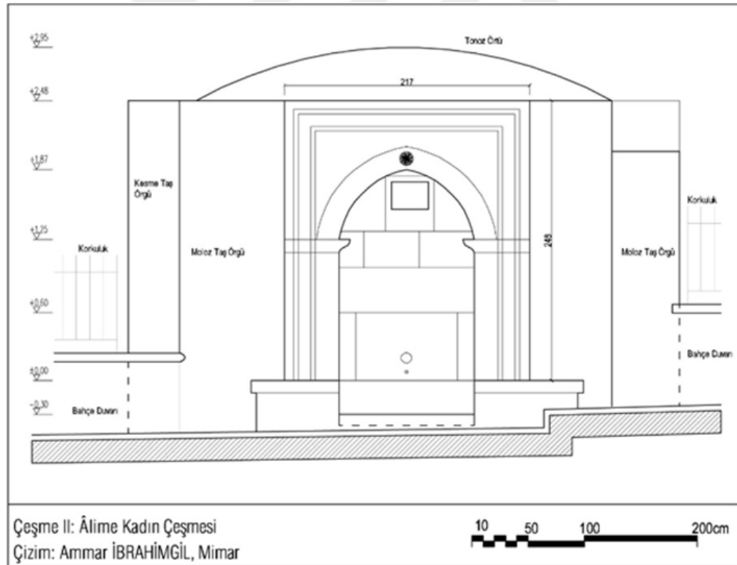
Şekil 4.8. Alime Kadın Çeşmesi cephe çizimi 120
