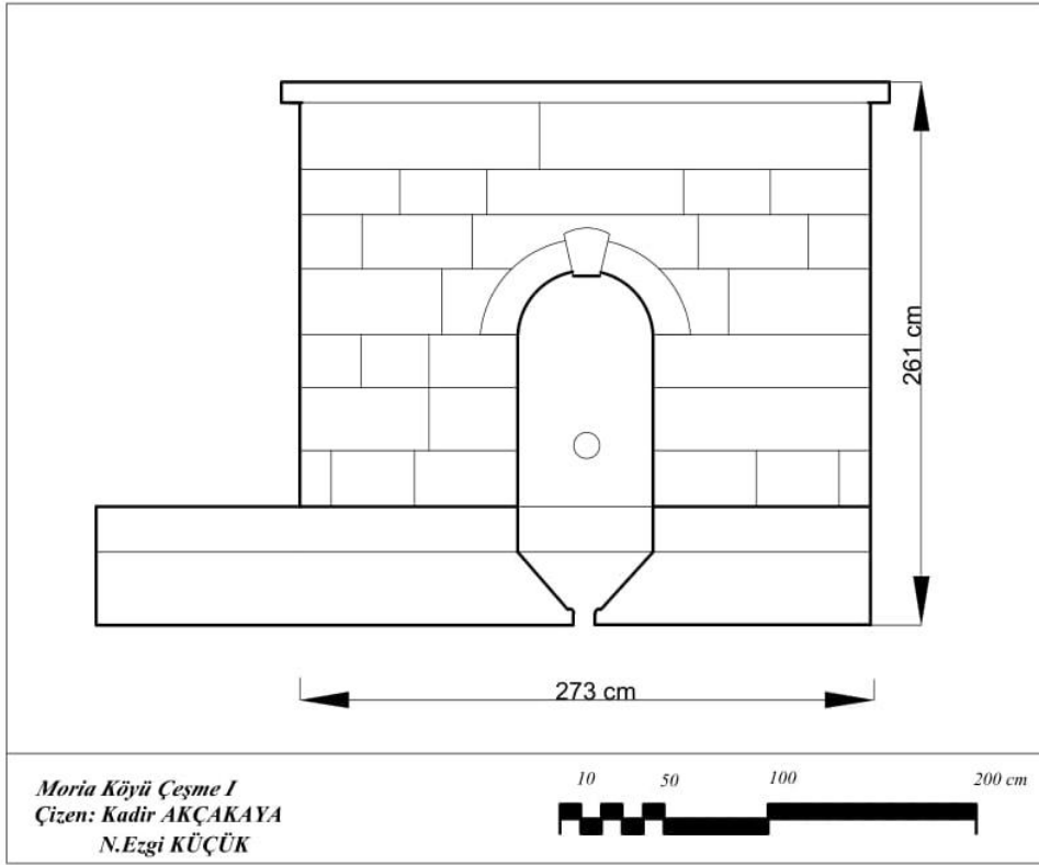
Şekil 4.137. Moria Köyü Çeşme 1 cephe çizimi
