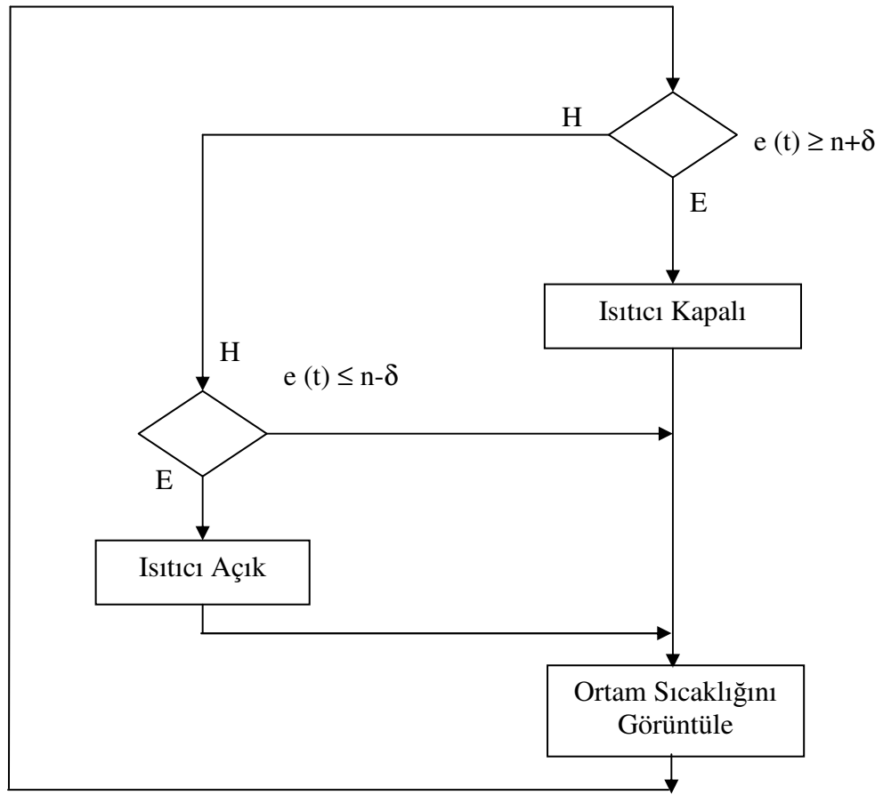
Şekil 4.6. On/Off kontrol akış şeması
