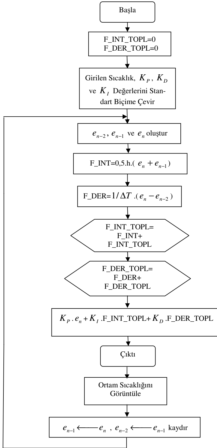
Şekil 4.17. Oransal+İntegral+Türevsel kontrol akış şeması
