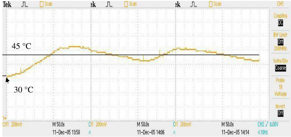
Şekil 5.4. On/Off 30-45 °C, diferansiyel aralık=3
