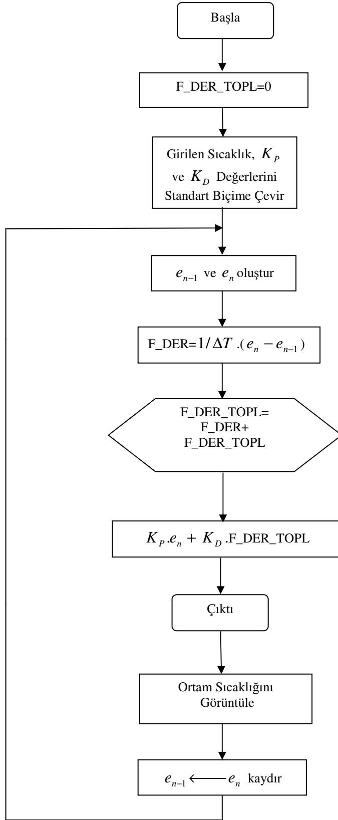
Şekil 4.15. Oransal+Türevsel kontrol akış şeması
