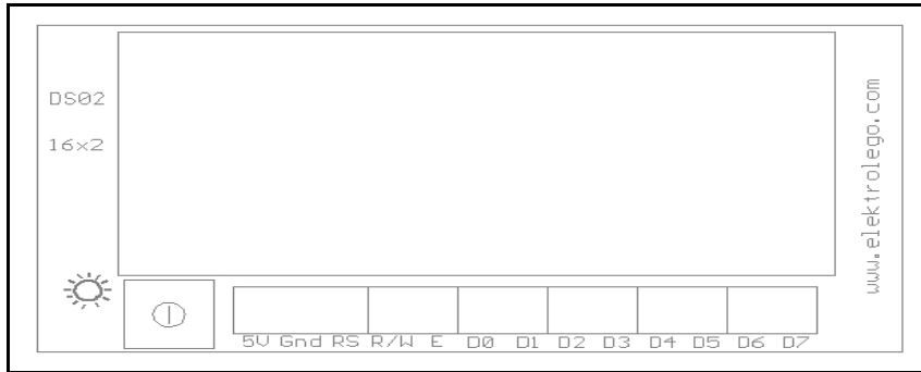
Şekil 2.12. LCD kartı yerleşim şeması
