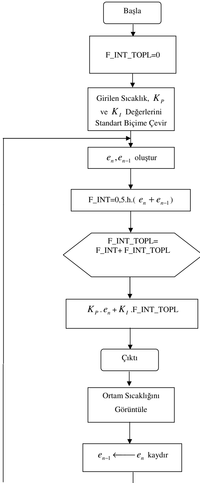
Şekil 4.12. Oransal+İntegral kontrol akış şeması
