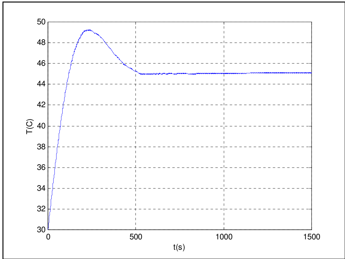
Şekil 5.20. Simulink-PID 30-45 °C, K_p=50 , K_D=7 , K_I=0,6
