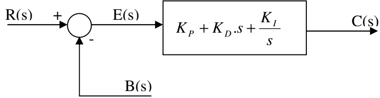
Şekil 4.16. Oransal+İntegral+Türevsel kontrol blok diyagramı
