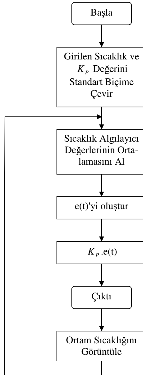
Şekil 4.9. Oransal kontrol akış şeması
