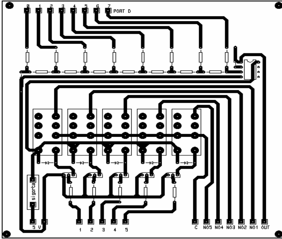
Şekil 2.7. Röle&D/A dönüştürücü kartı baskı devre şeması
