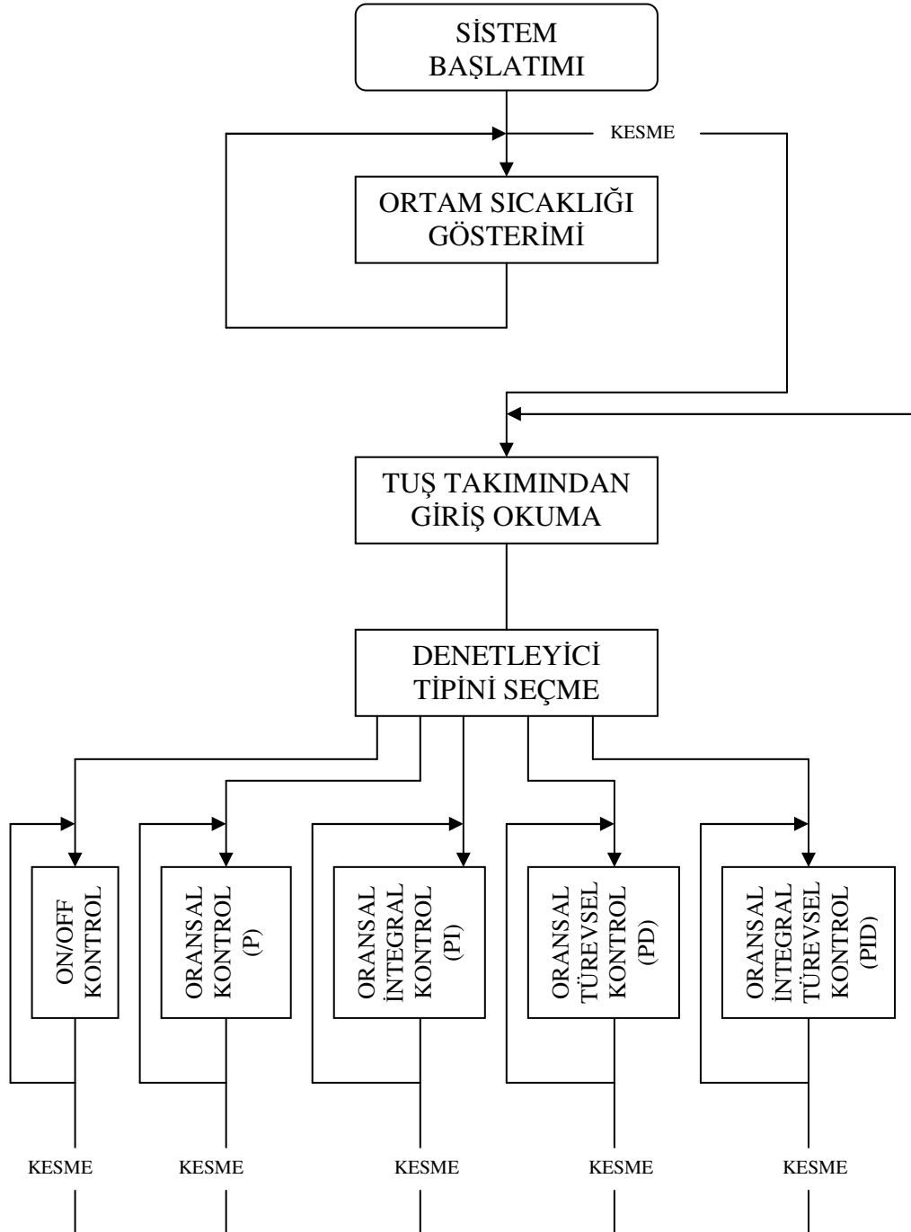
Şekil 4.1. Sistem yazılımı genel akış şeması
