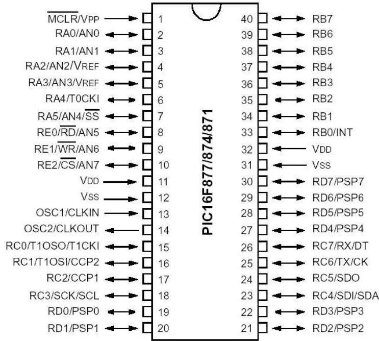
Şekil 2.2. PIC 16F877 bacak (port) bağlantıları
