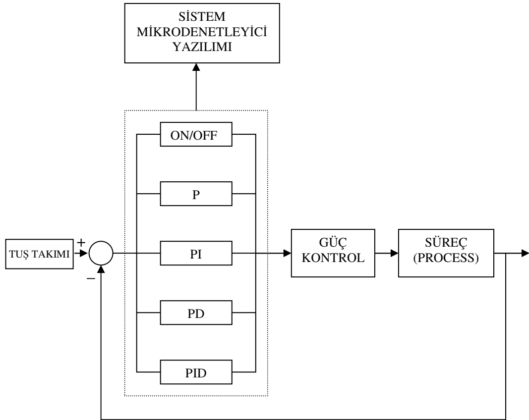
Şekil 4.2. Sistem kapalı döngü blok diyagramı
