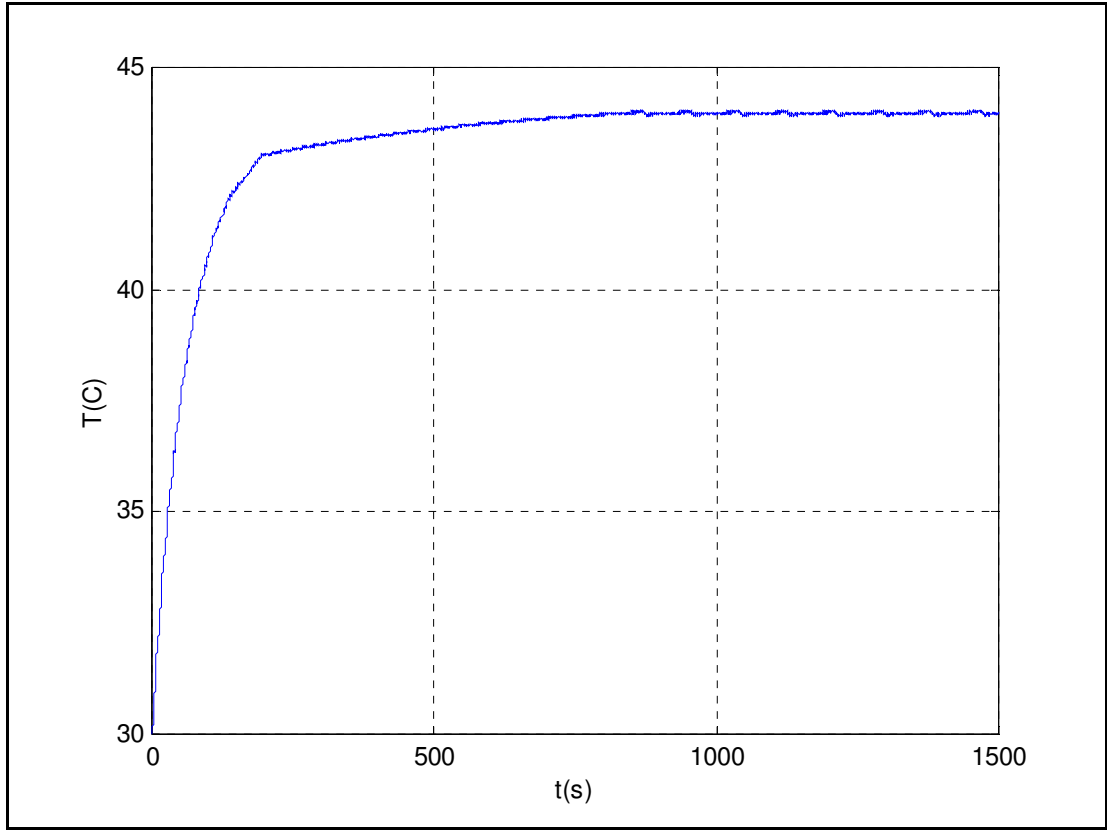
Şekil 5.14. Simulink- PD 30-45 °C, K_p=70 , K_D=6
