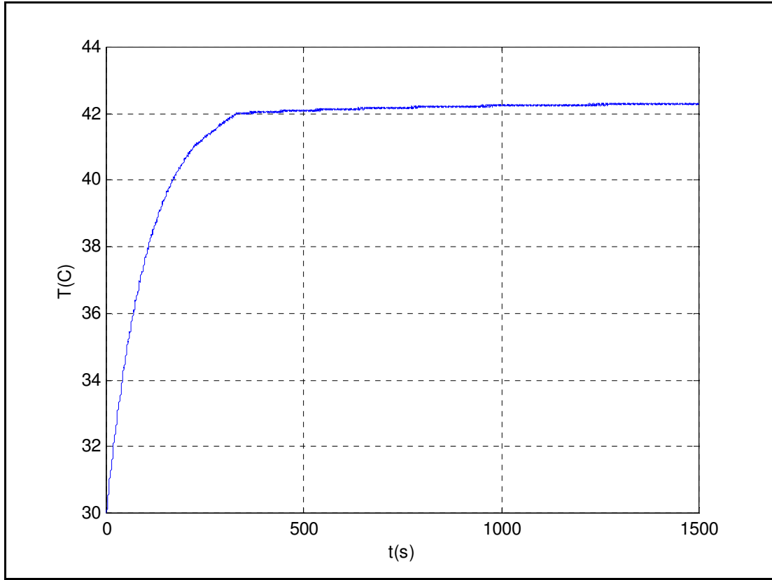
Şekil 5.8. Simulink- P 30-45 °C, K_p=40
