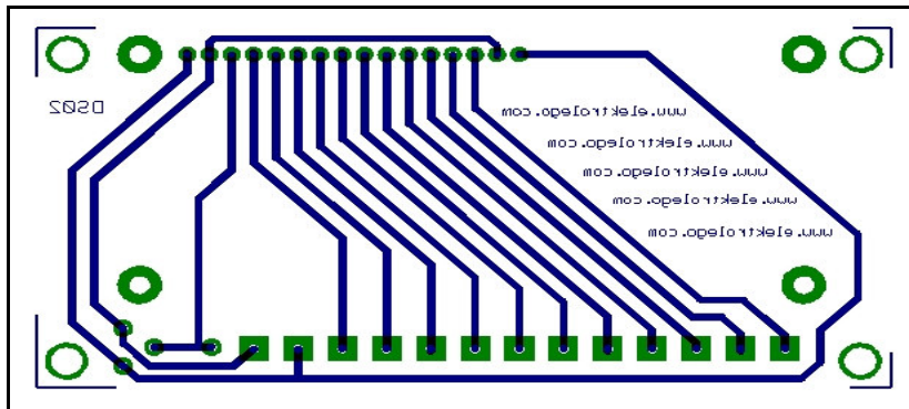
Şekil 2.13. LCD kartı baskı devre şeması
