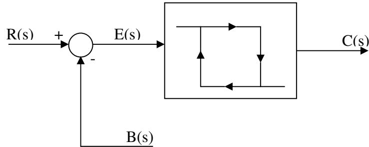
Şekil 4.4. On/Off kontrol blok diyagramı
