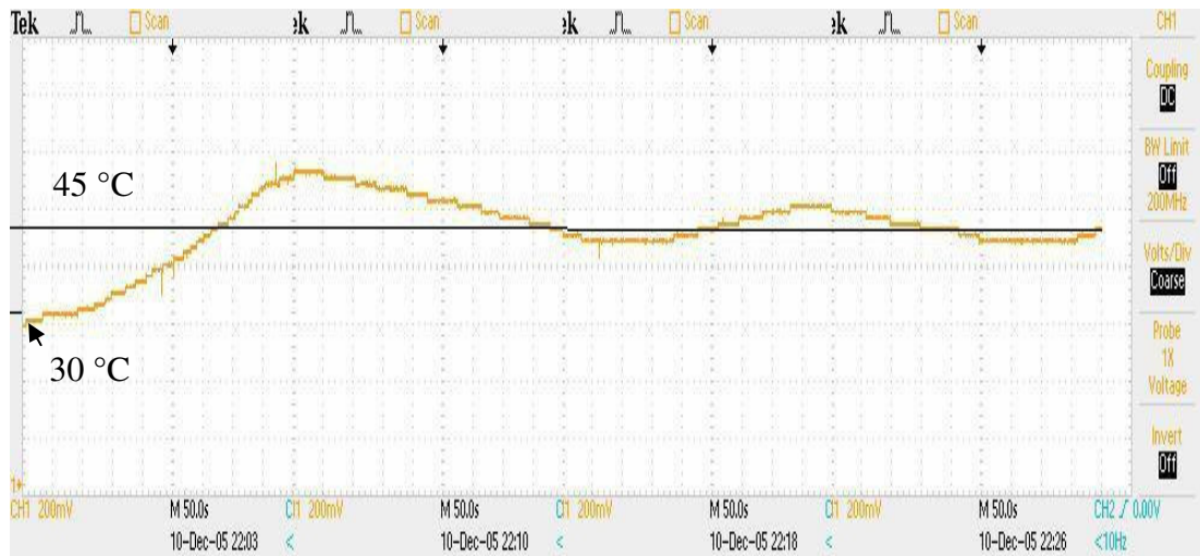
Şekil 5.9. Oransal+İntegral 30-45 °C, K_p=60 , K_I=0,6
