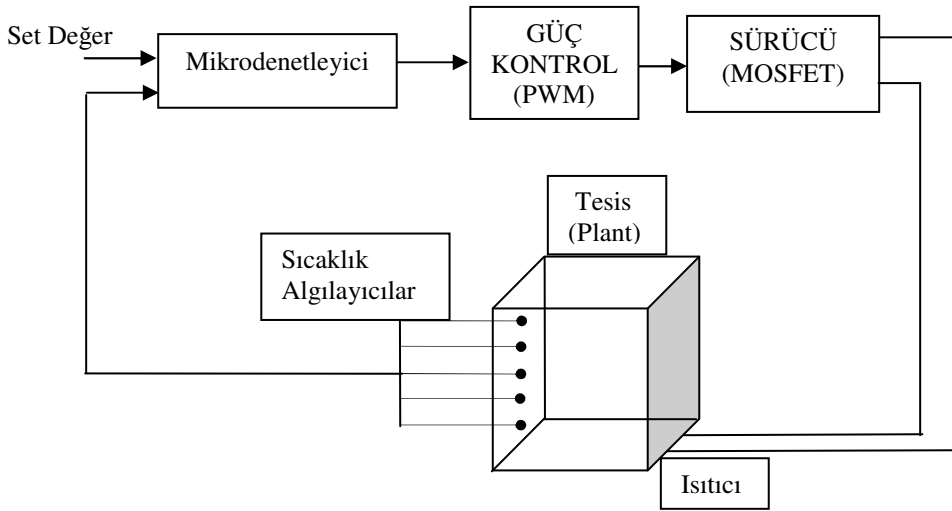
Şekil 2.1. Mikrodenetleyici kontrollü ısıl sistem genel diyagramı
