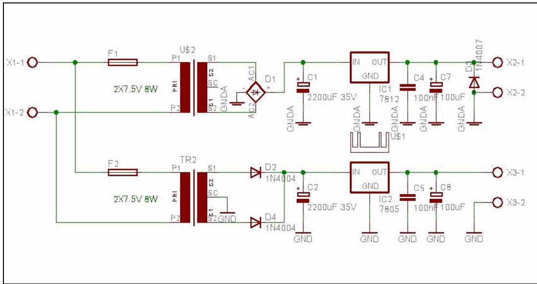
Şekil 2.10. Güç kartı devre şeması
