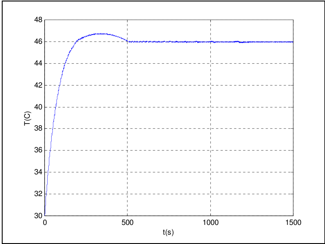
Şekil 5.18. Simulink-PID 30-45 °C, K_p=70 , K_D=5 , K_I=0,3
