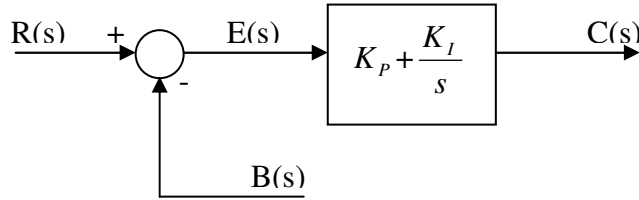
Şekil 4.10. Oransal+İntegral kontrol blok diyagramı
