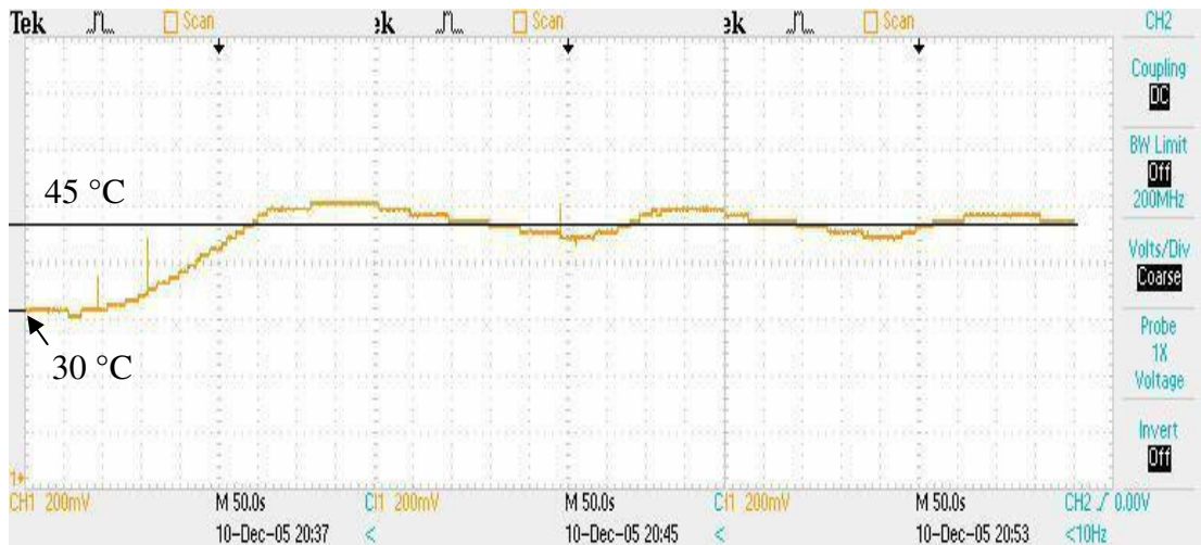
Şekil 5.3. On/Off 30-45 °C, diferansiyel aralık=1
