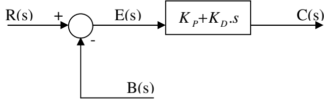
Şekil 4.13. Oransal+Türevsel kontrol blok diyagramı
