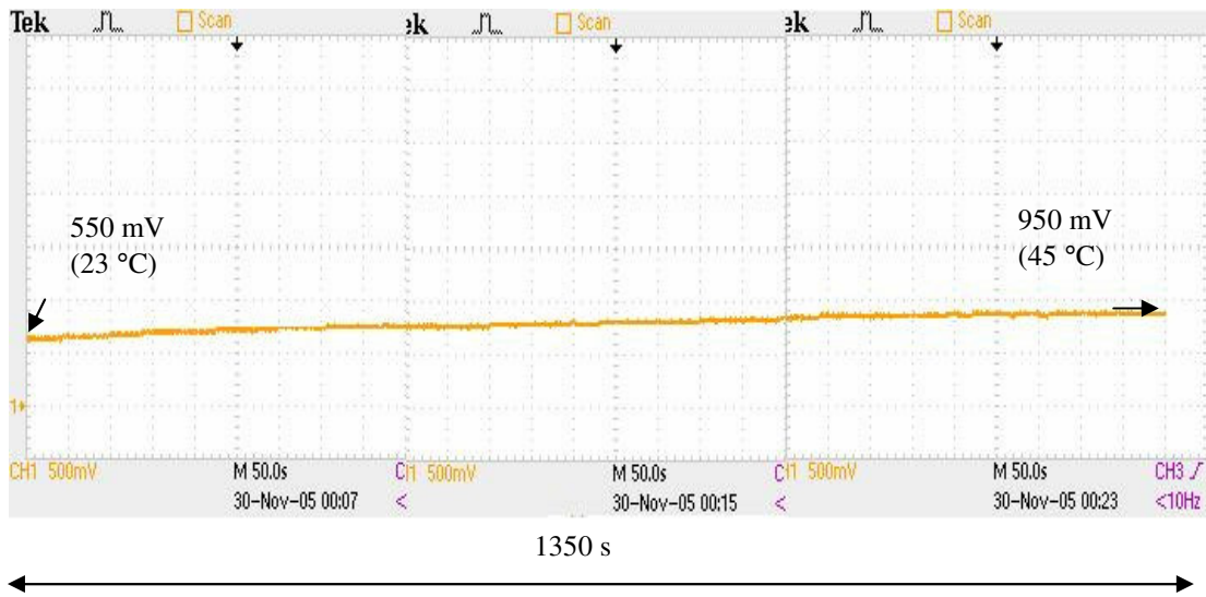
Şekil 5.2. Isıtıcıya 100 \text{ V} giriş gerilimi uygulanmasıyla elde edilen çıkış karakteristiği
