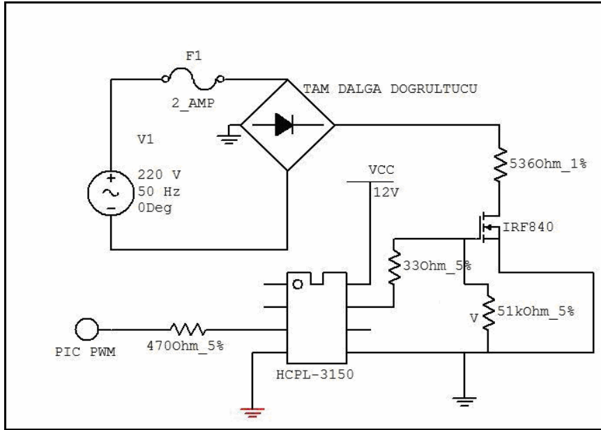
Şekil 2.8. PWM kartı devre şeması
