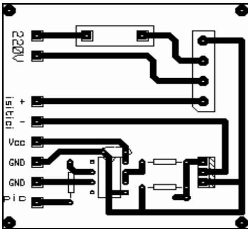
Şekil 2.9. PWM kartı baskı devre şeması
