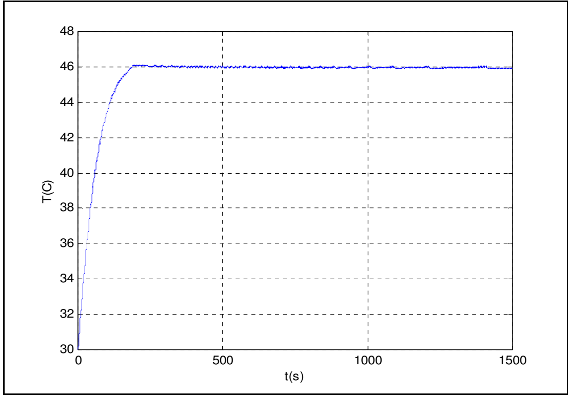
Şekil 5.12. Simulink- PI 30-45 °C, K_p=90 , K_I=0,3
