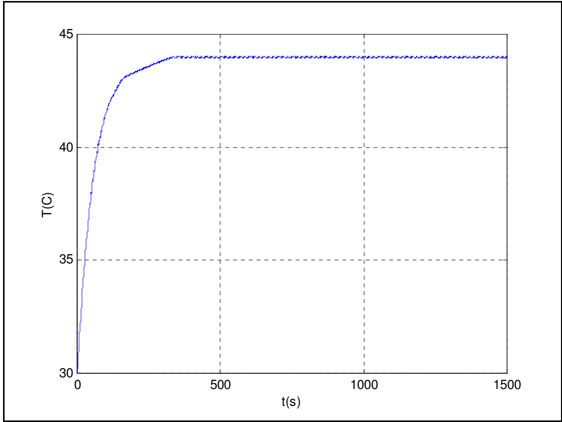
Şekil 5.6. Simulink- P 30-45 ^{\circ}\text{C} , K_p=80
