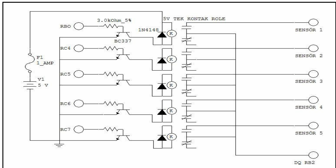
Şekil 2.5. Röle devre şeması
