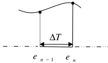
Şekil 4.14. Oransal+Türevsel kontrol örnekleme yaklaşımı
