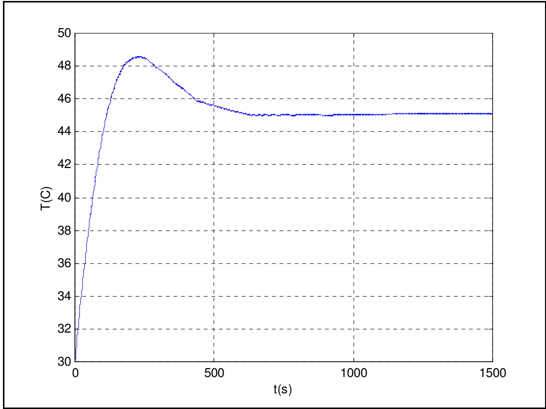
Şekil 5.10. Simulink- PI 30-45 ^{\circ}\text{C} , K_p=60 , K_I=0,6
