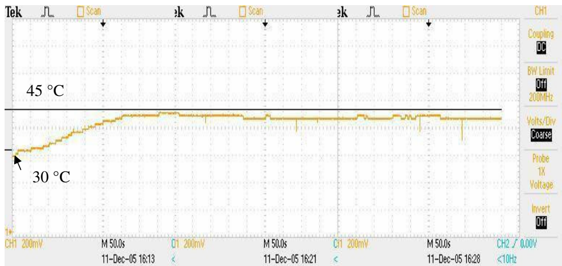
Şekil 5.13. Oransal+Türevsel 30-45 °C, K_p=70 , K_D=6
