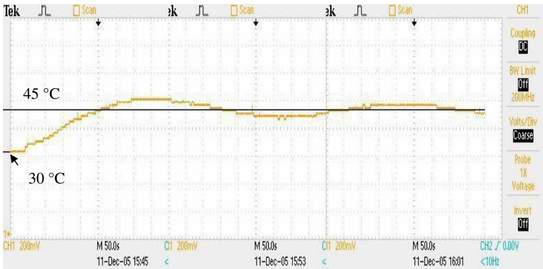
Şekil 5.11. Oransal+İntegral 30-45 ^{\circ}\text{C} , K_p=90 , K_I=0,3
