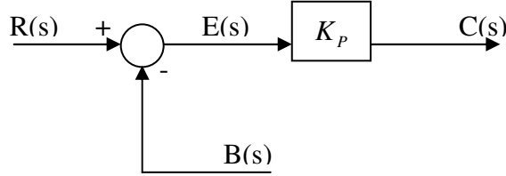
Şekil 4.7. Oransal kontrol blok diyagramı
