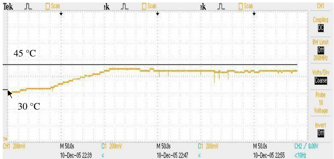
Şekil 5.15. Oransal+Türevsel 30-45 °C, K_p=50 , K_D=4
