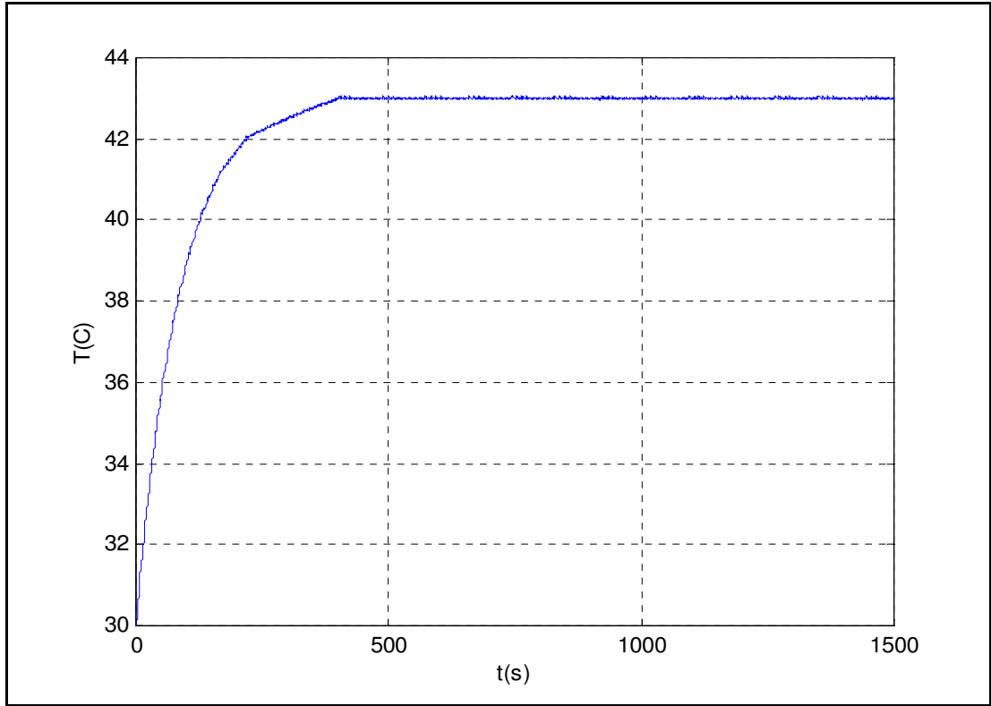
Şekil 5.16. Simulink- PD 30-45 °C, K_p=50 , K_D=4
