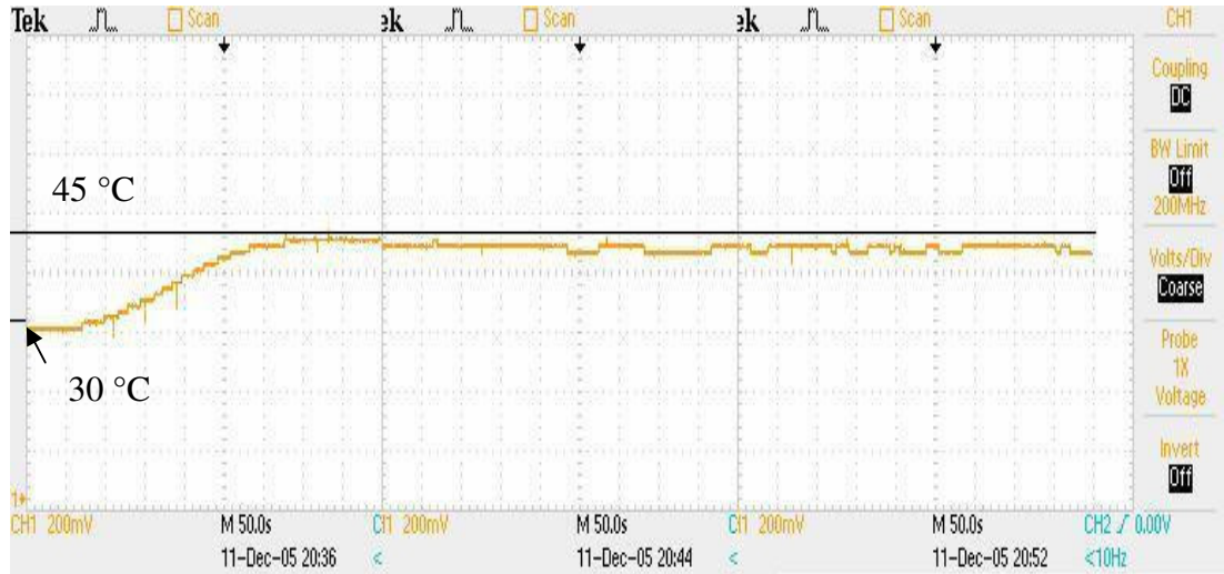
Şekil 5.5. Oransal 30-45 °C, K_p=80
