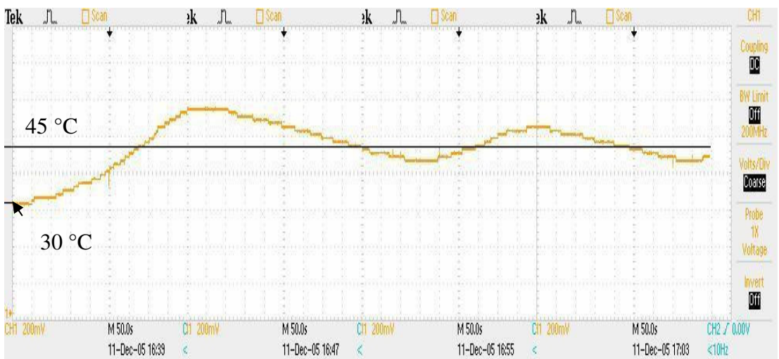
Şekil 5.19. Oransal+İntegral+Türevsel 30-45 °C, K_p=50 , K_D=7 , K_I=0,6
