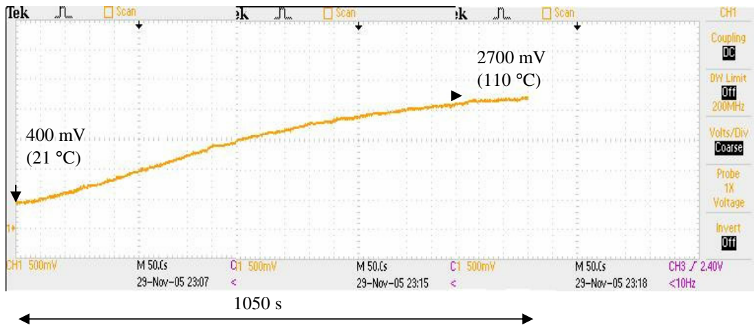
Şekil 5.1. Sistemin açık döngü birim basamak tepkisi
