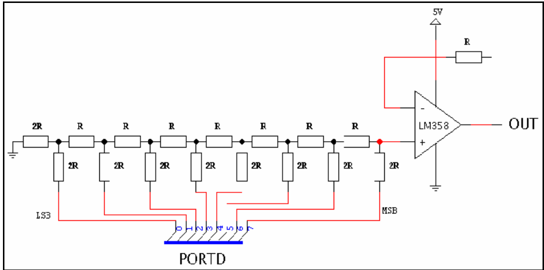
Şekil 2.6. D/A dönüştürücü devre şeması
