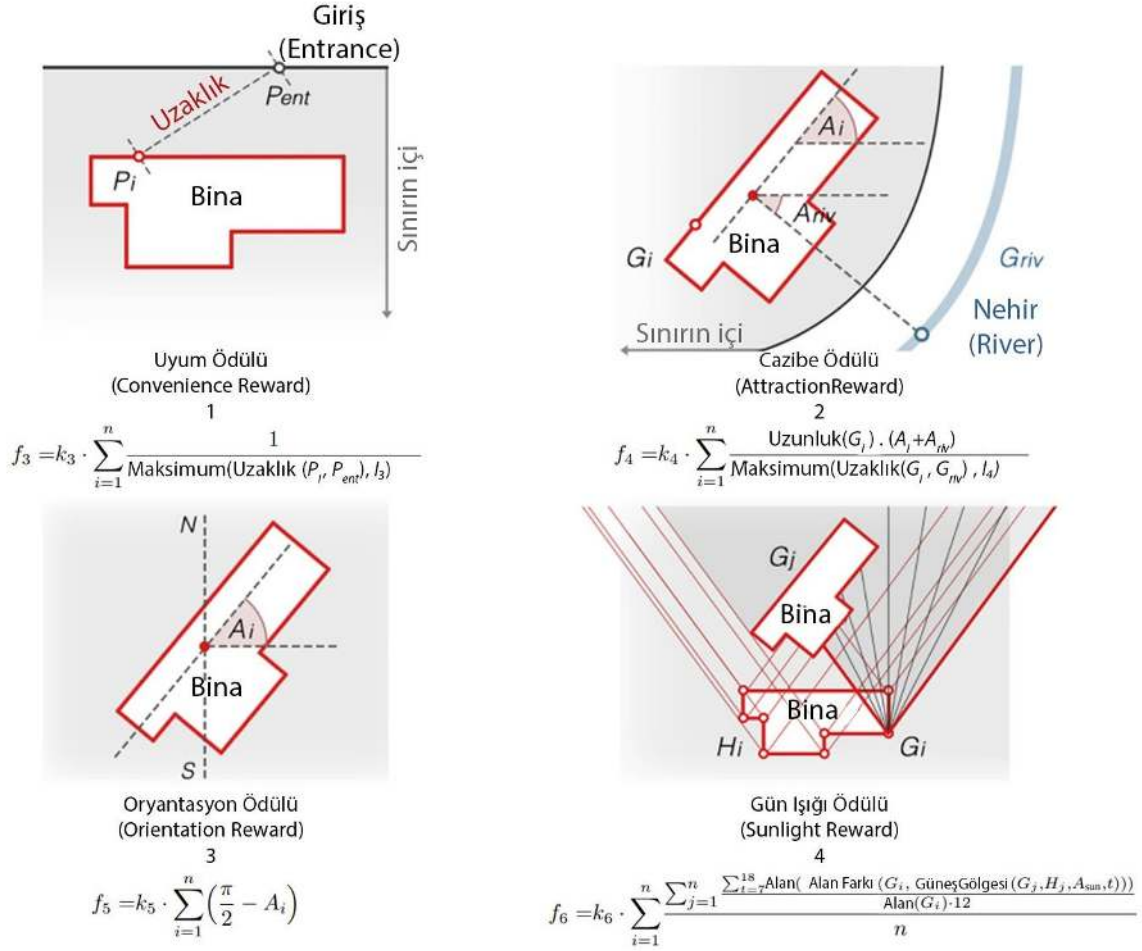
Şekil 51: Ödül Fonksiyonları [95]
