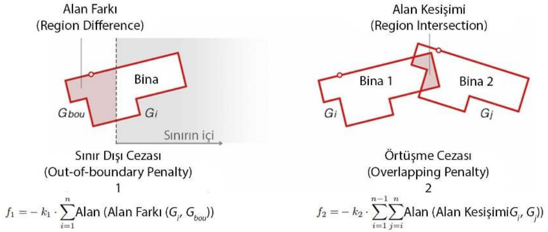
Şekil 50: Ceza Fonksiyonları [95]
