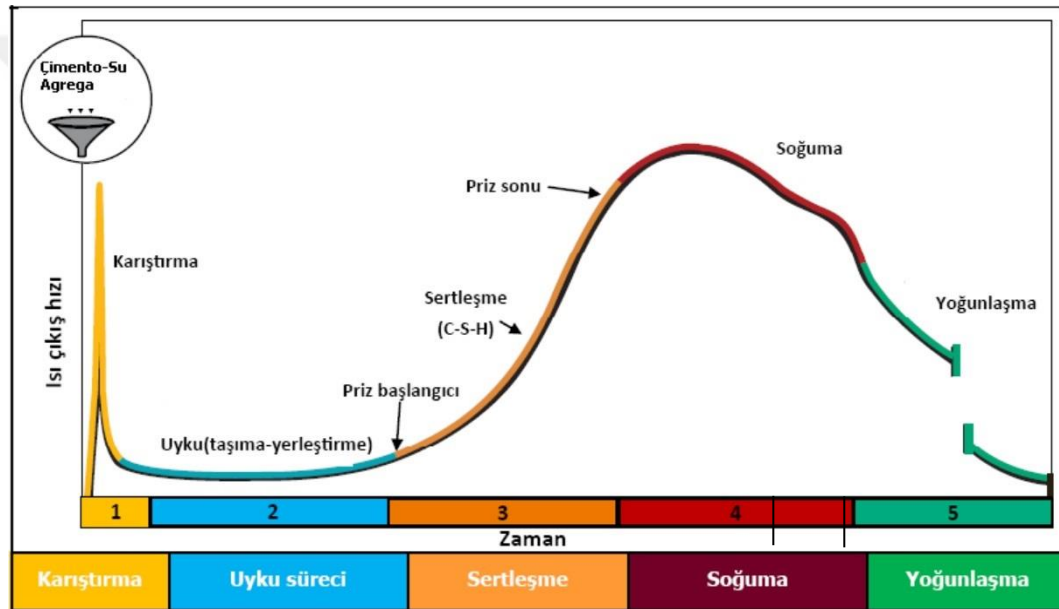
Resim 5.1 Hidratasyon Süreçleri [56]
