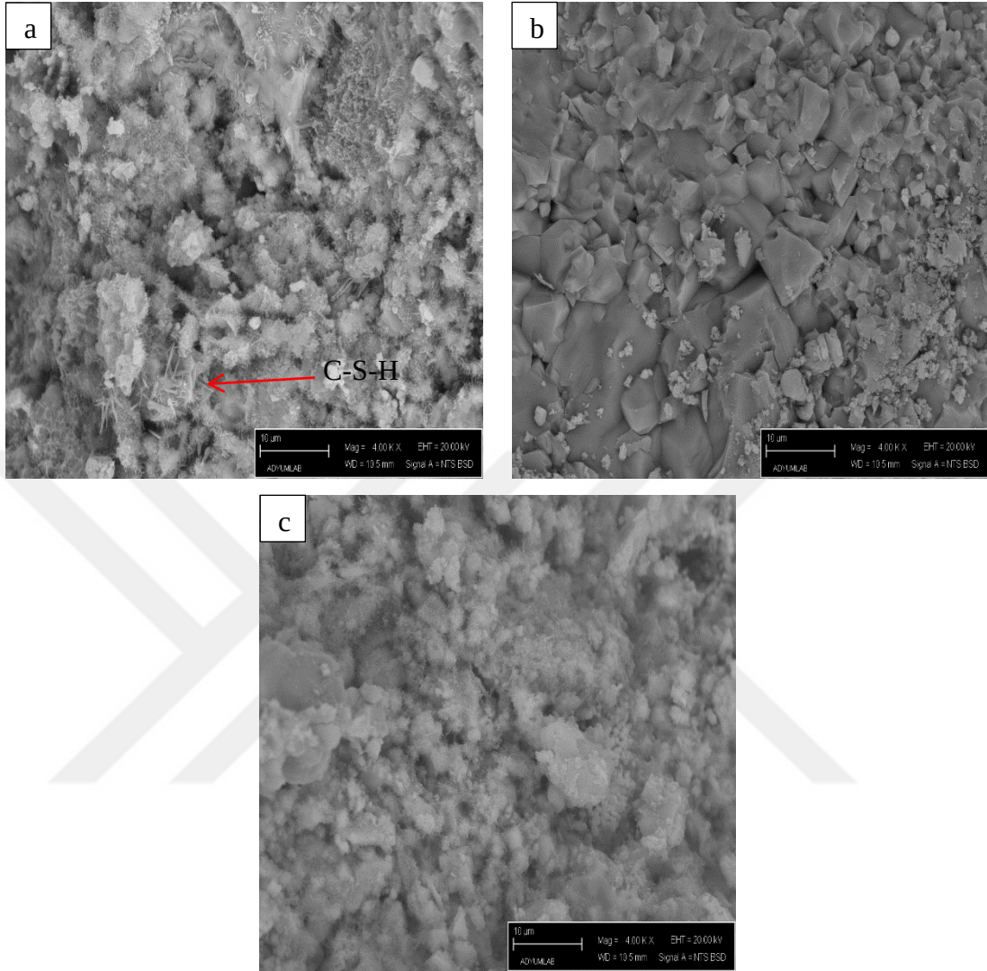
Resim 7.9 Yüksek Fırın Cürufu Katkılı 4 Bar Basıncılı Kürüne Tabi Tutulan Numunelerin Mikroyapı Görüntüleri
