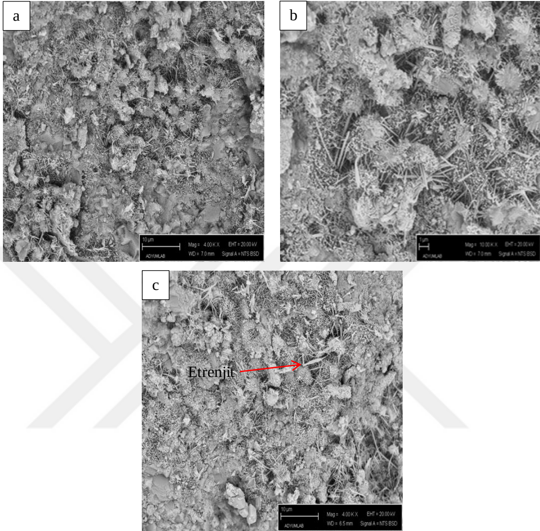
Resim 7.2 Uçucu kül katkıli standart su kürüne tabi tutulan numunelerin mikroyapı görüntüleri
