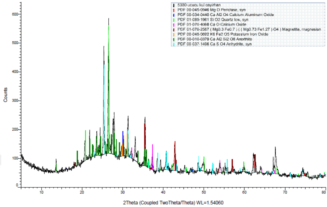
Resim 6.1 Uçucu Küle Ait XRD Analizi
