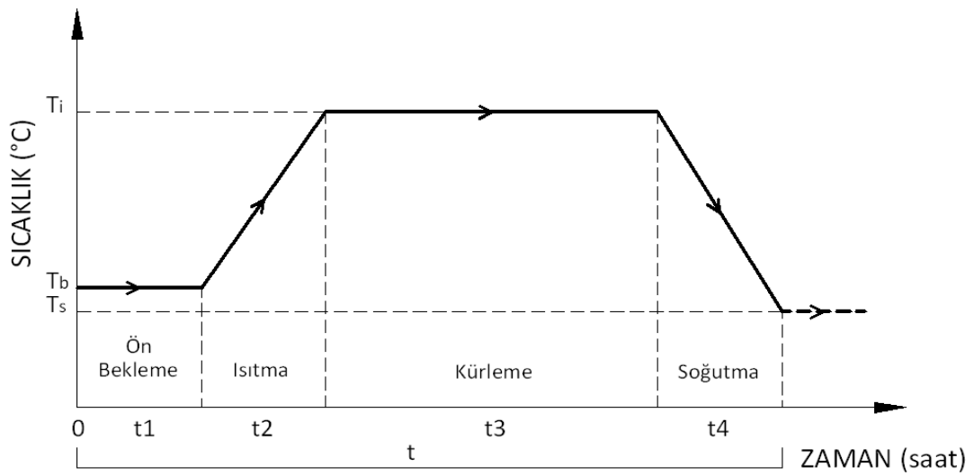
Resim 4.1 Tipik Bir Isıtım İşlem Çevriminin Aşamaları [53]
