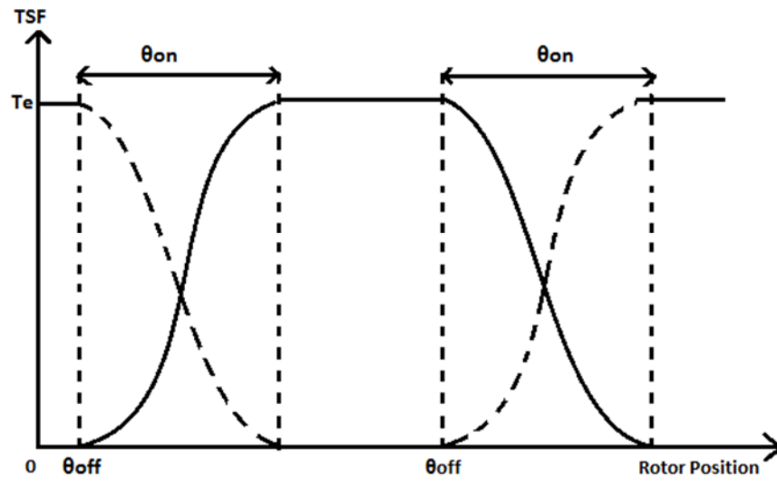
Fig. 3.6. Cubic TSF [7]
