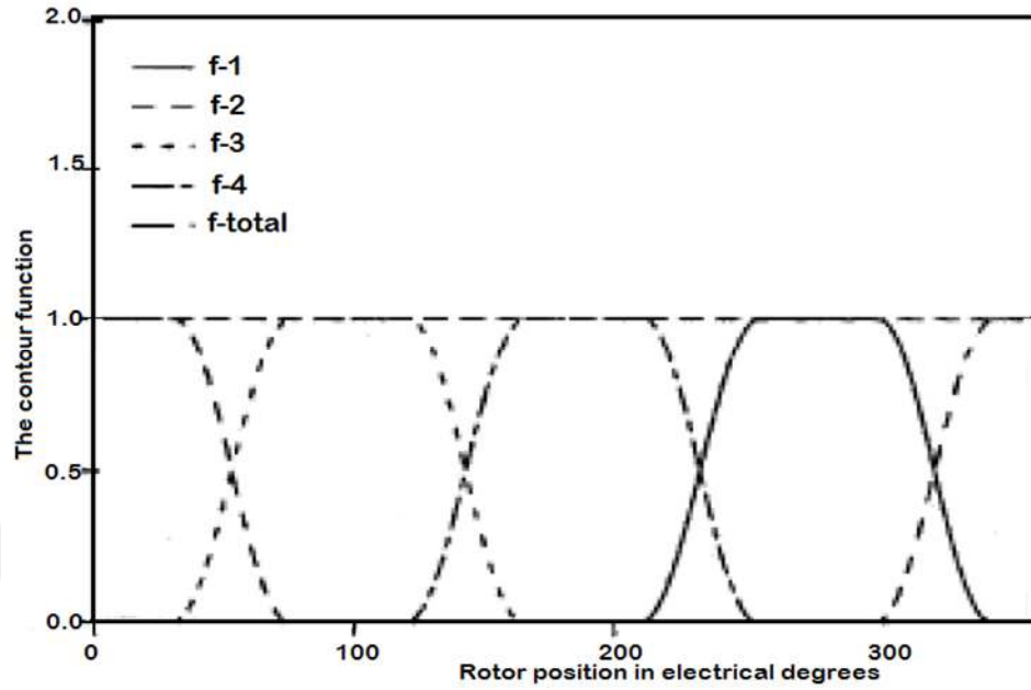
Fig. 3.5. Sinusoidal TSF [7]
