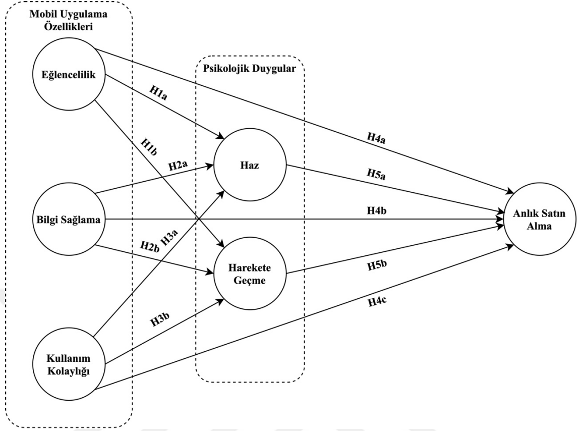
Şekil 1: Araştırma Modeli
