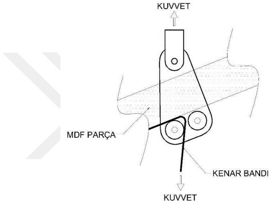
Şekil 3.1. Kenar bandı soyma deneyi için aparat [Fotoğraf: Burak Mirac Yılmaz, 2018]
