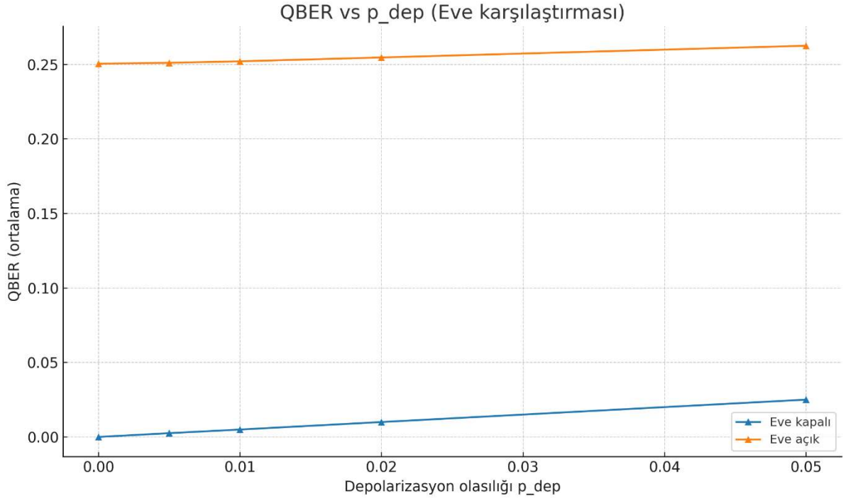
Şekil 2.7 QBER'in p_{dep} 'e bağlı karşılaştırması (Eve açık/kapalı). Dinleyici varlığında QBER artmaktadır.
