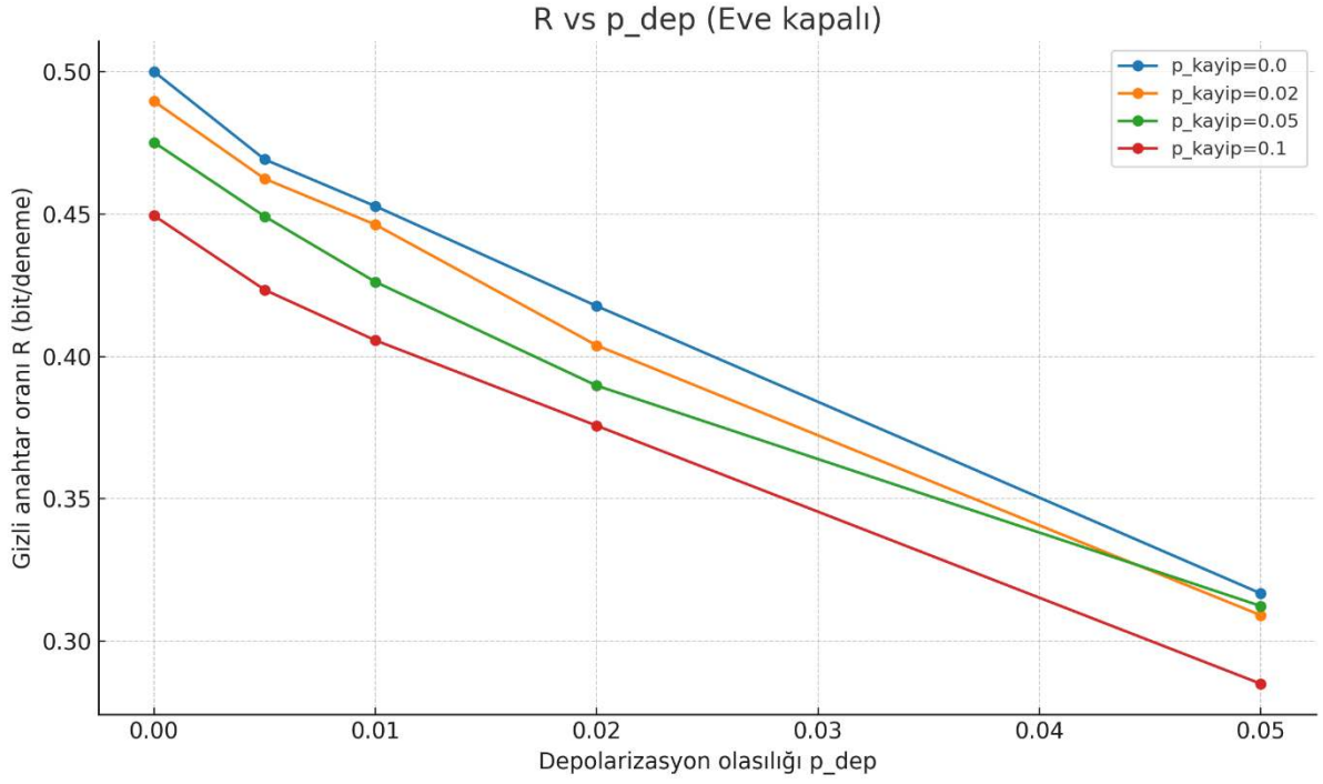
Şekil 2.5 Eve kapalıyken R 'nin p_{dep} 'e bağlı değişimi; farklı p_{kayıp} değerleri için ortalama değerler.
