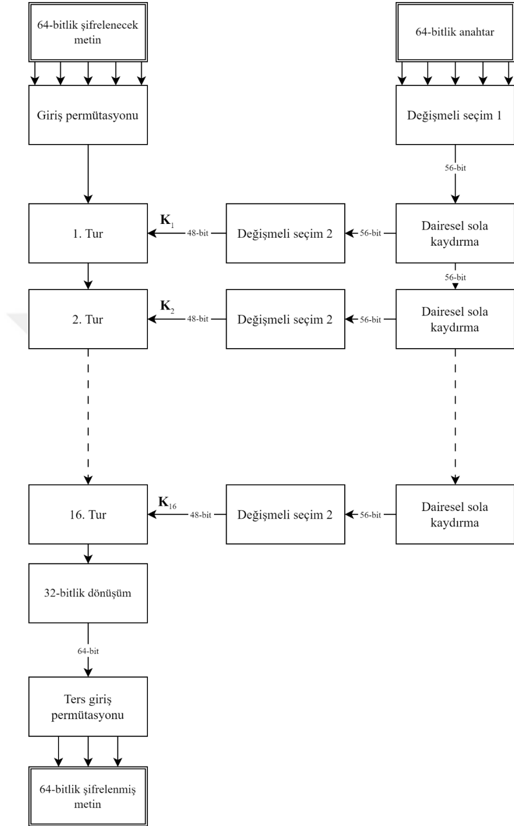
Şekil 1.3 DES'in Çalışma Prensibi
