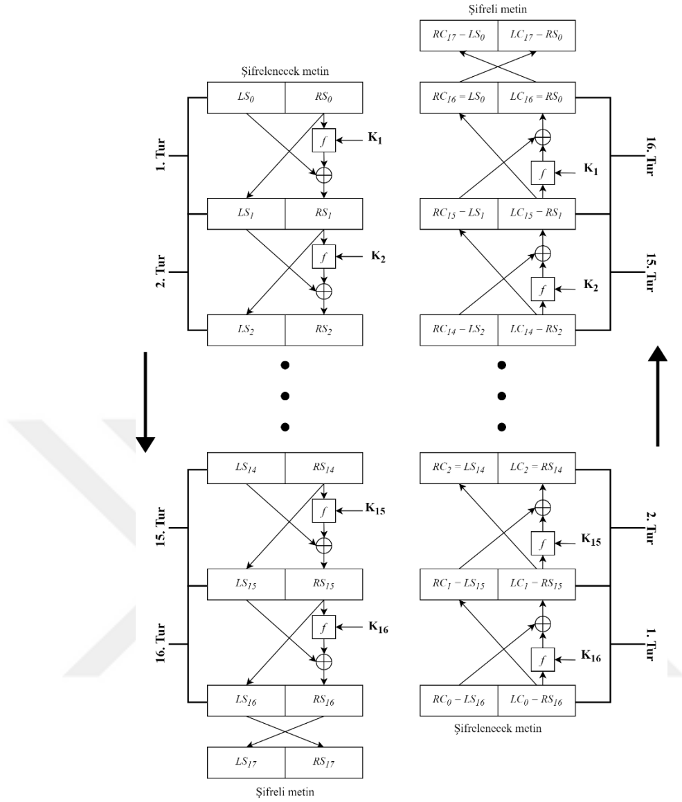
Şekil 1.1 Feistel Ağı'nın Çalışma Prensibi
