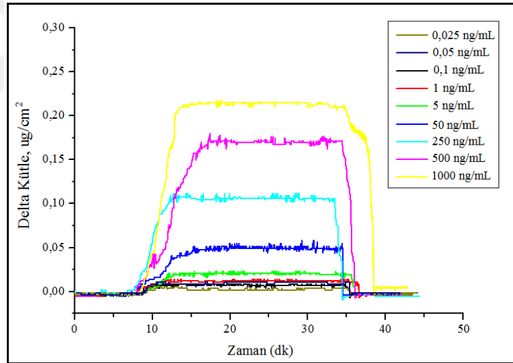
Şekil 4.10. C6-HSLBaskılanmış QCM Çiplerde C6-HSL Tayinine Derişimin Etkisi. Delta Kütle-Zaman Grafiği. pH: 7.0; akış hızı: 0.5 mL/dak.; T: 25 °C.
