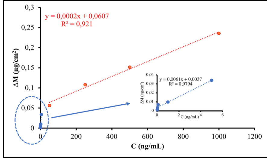
Şekil 4.13. C6-HSL baskılanmış QCM sensöre ait derişim ile Delta Kütle ( \Delta m ) arasındaki bağıntı. pH: 7.0; akış hızı: 0,5 mL/dak.; sıcaklık: 25 °C.
