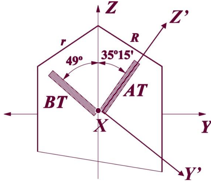
Şekil 2.24. Bir kuvars kristalinin AT ve BT kesim düzlemi [160].
