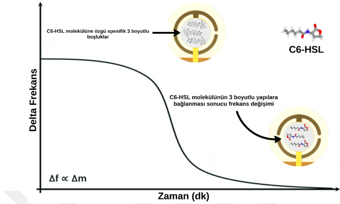
Şekil 2.26. Kuvars kristal mikrobals biyosensörünün mekanizmasının resimsel gösterimi.
