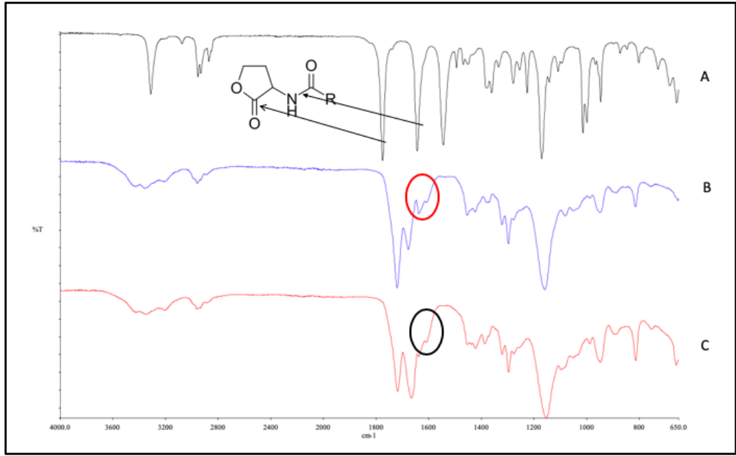
Şekil 4.2. A. C6-HSL, B. C6-HSLbaskılanmış C. baskılanmamış polimerik membranların FTIR-ATR spektrumu.
