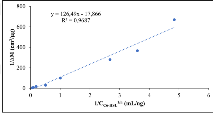
Şekil 4.20. Langmuir-Freundlich adsorpsiyon izotermi.
