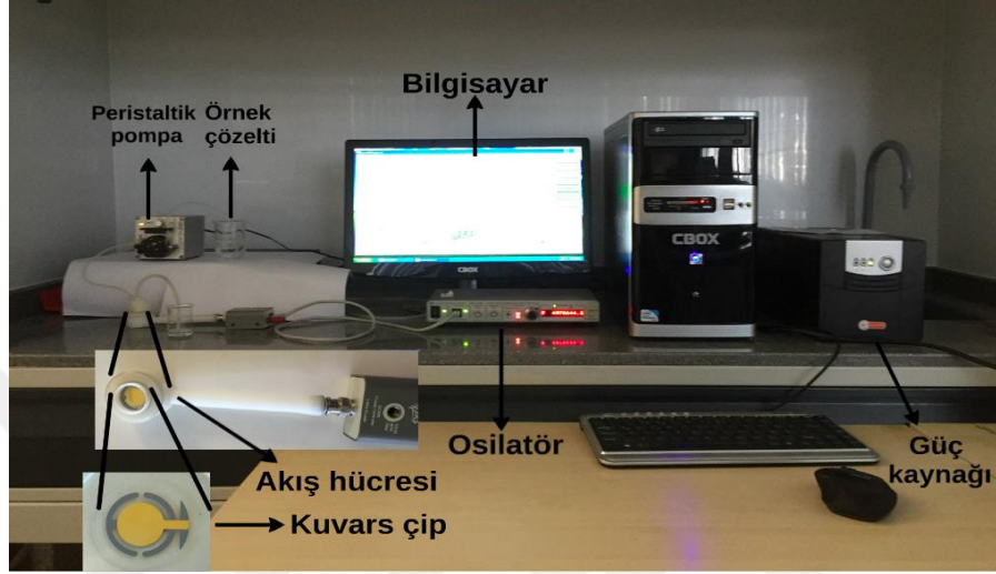
Şekil 3.6. Kullanılan QCM sistemi.
