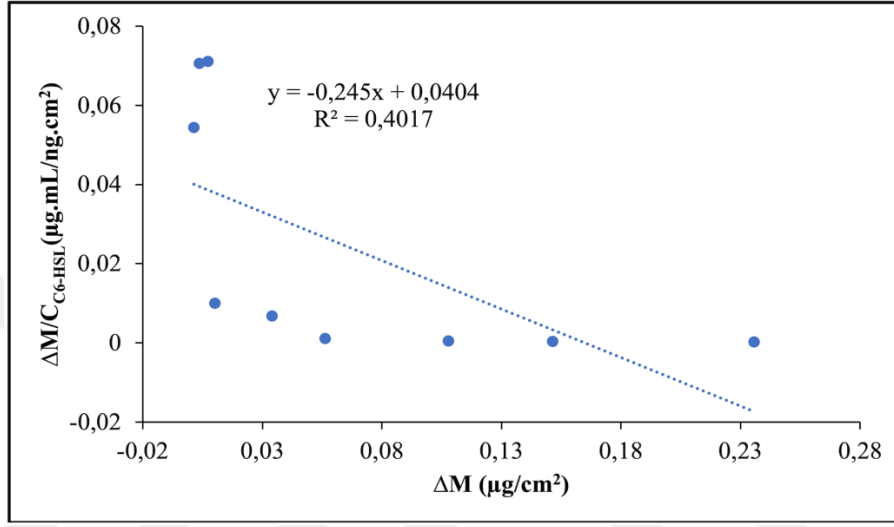
Şekil 4.15. C6-HSL baskılanmış QCM sensörün denge kinetik analiz doğrusu (Scatchard).
