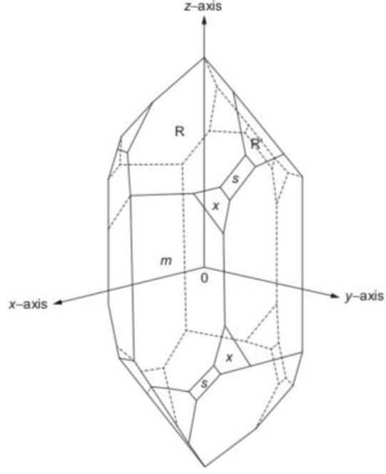
Şekil 2.20. Doğal kuvars kristalinin ekseni tipik dış formu [156].
