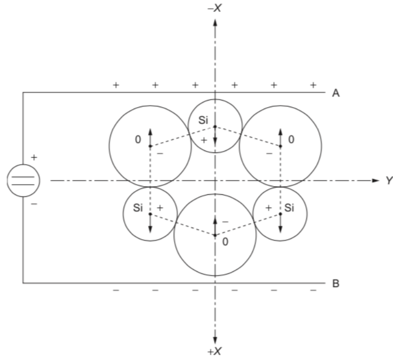
Şekil 2.23. Ters piezoelektrik [156].
