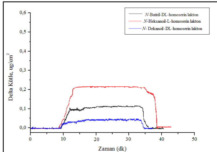
Şekil 4.21. C4-HSL, C6-HSL ve C10-HSL moleküllerinin C6-HSL baskılanmış (MIP) QCM sensöre verdiği kütle-zaman grafiği; Çözelti derişimleri: 1000 ng/mL.
