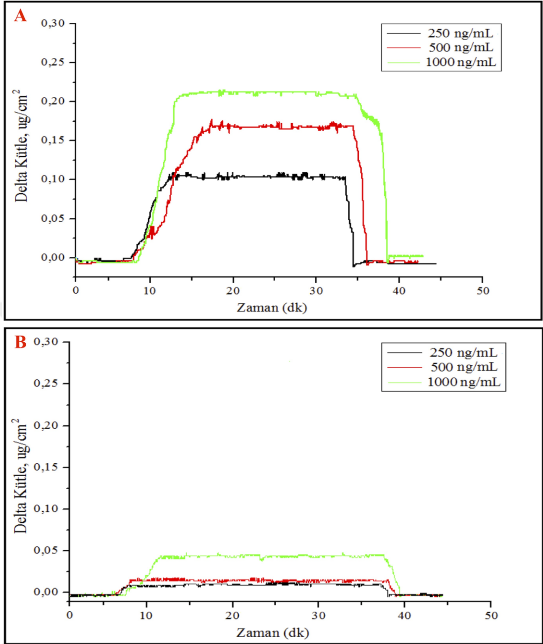
Şekil 4.14. C6-HSL baskılanmış (A) ve baskılanmamış (B) QCM sensörün derişim grafikleri.
