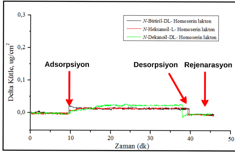
Şekil 4.24. C4-HSL, C6-HSL ve C10-HSL moleküllerinin C6-HSL baskılanmamış (NIP) QCM sensöre karşı verdiği toplu haldeki kütle-zaman grafiği; Çözelti derişimleri: 1000 ng/mL.
