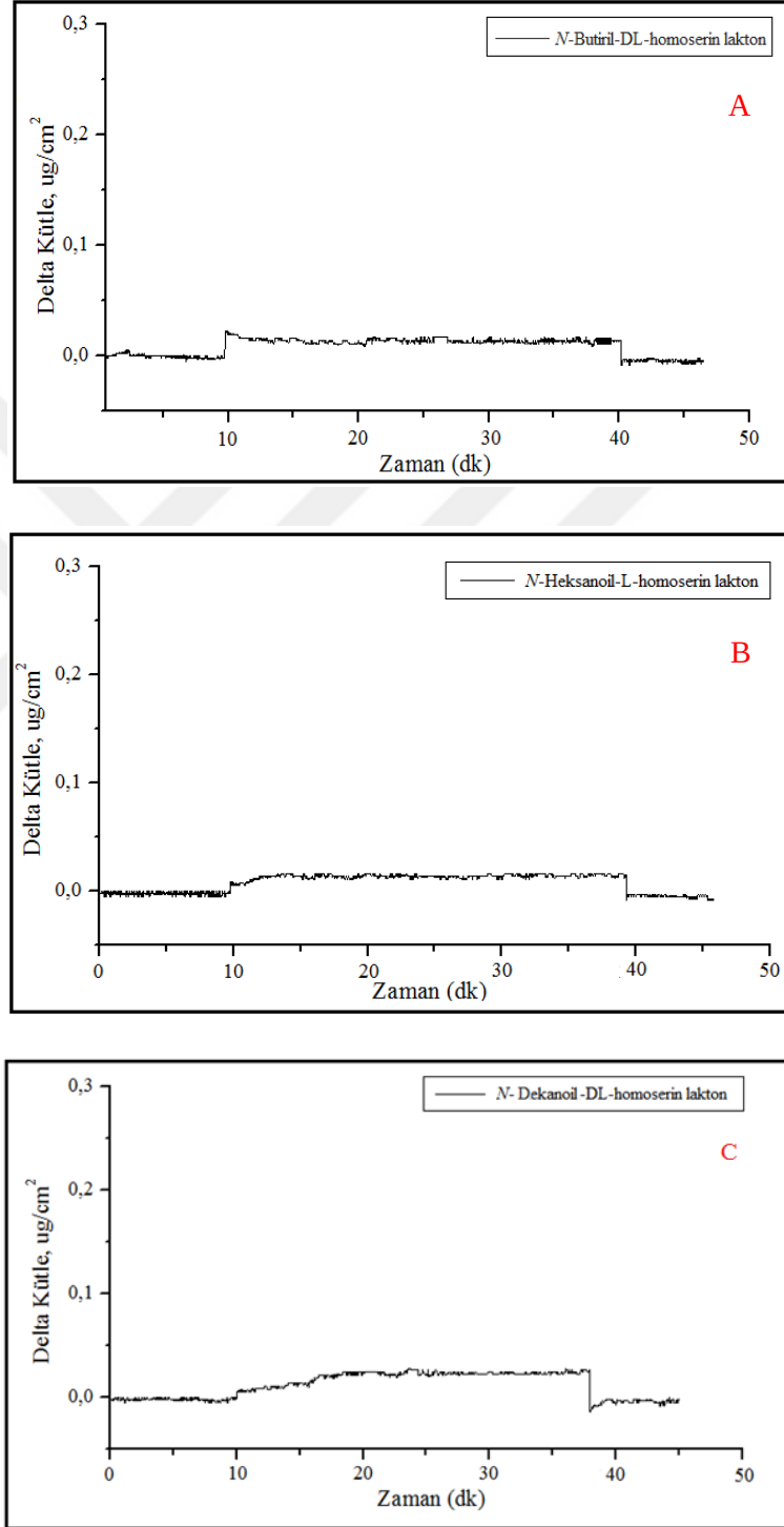
Şekil 4.23. C4-HSL, C6-HSL ve C10-HSL moleküllerinin baskılanmamış (NIP) QCM sensöre karşı verdiği kütle-zaman grafiğı; Çözelti derişimleri: 1000 ng/mL.
