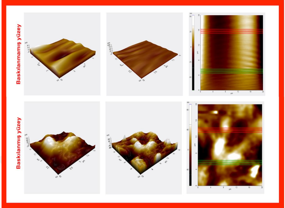
Şekil 4.4. Baskılanmış ve baskılanmamış membranların atomik kuvvet mikroskobu görüntüleri.
