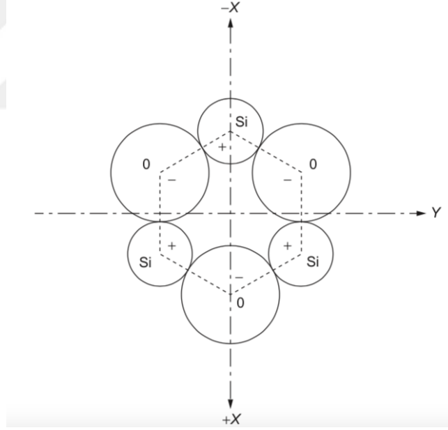
Şekil 2.21. z ekseninden bakıldığında kuvars z içindeki Si ve O atomu [156].
