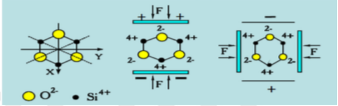
Şekil 2.17. Bir kuvars kristalindeki piezoelektrik etkisinin açıklaması [155].
