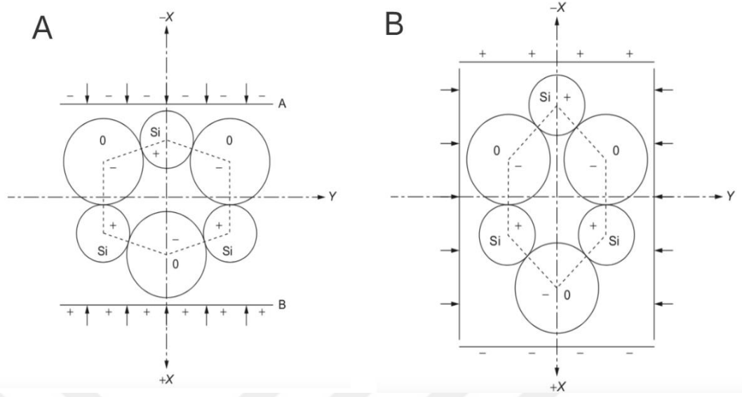
Şekil 2.22. A: Doğru boyunca piezoelektrik B: Dik piezoelektrik [156].
