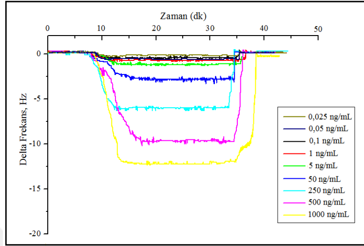
Şekil 4.9. C6-HSLBaskılanmış QCM ÇiplerdeC6-HSL Tayinine Derişimin Etkisi. Delta Frekans-Zaman Grafiği. pH: 7.0; akış hızı: 0.5 mL/dak.;T: 25 °C.
