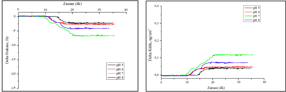
Şekil 4.6. Eş-zamanlı QCM sonuçlarına pH'nın Etkisi (1/3 C6-HSL: AAm). Delta Frekans ve Delta Kütle Zaman Eğrileri. C6-HSL derişimi: 1000 ng/mL; akış hızı: 0,5 mL/dk; T: 25 °C.
