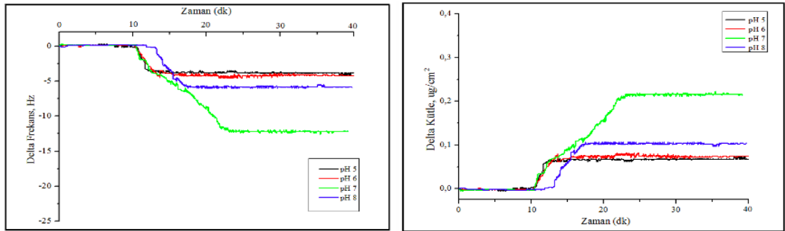
Şekil 4.7. Eş-zamanlı QCM sonuçlarına pH'nın Etkisi (1/3 C6-HSL: AAm). Delta Frekans ve Delta Kütle Zaman Eğrileri. C6-HSL derişimi: 1000 ng/mL; akış hızı: 0,5 mL/dk; T: 25 °C.
