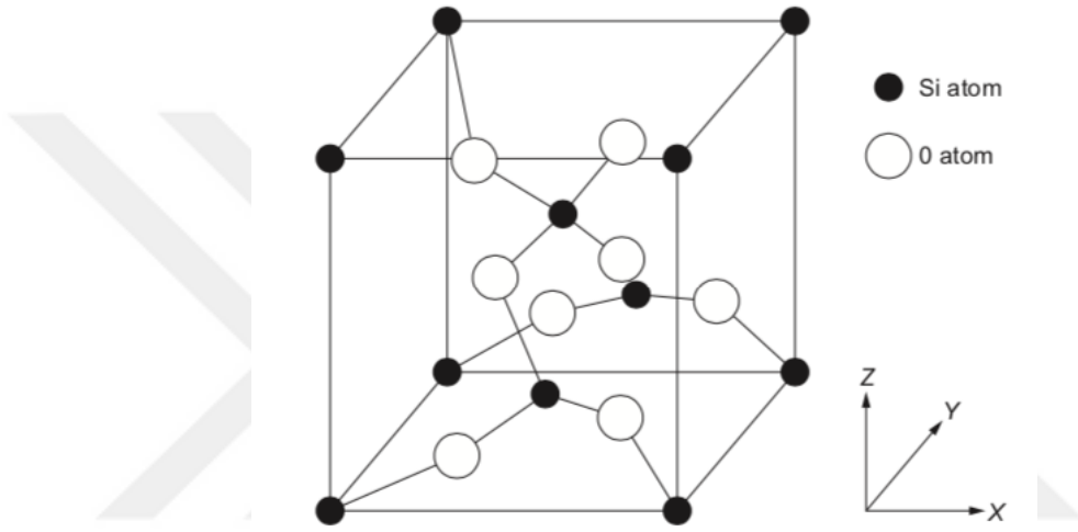
Şekil 2.19. \alpha -kuvarsın birim hücresi [156].
