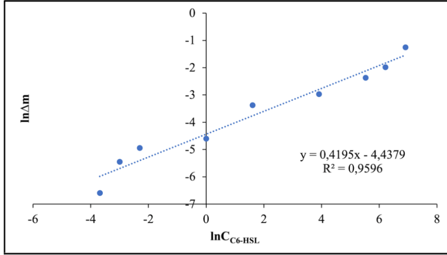
Şekil 4.19. Freundlich adsorpsiyon izotermi.
