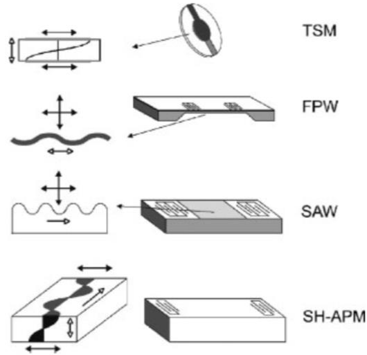
Şekil 2.16. Dalga yayılım tarzları ile karakterize edilen dört yaygın akustik dalga cihazı türü.
