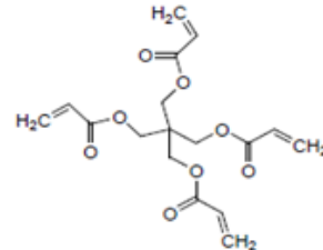
Pentaeritrol Tetraakrilat
