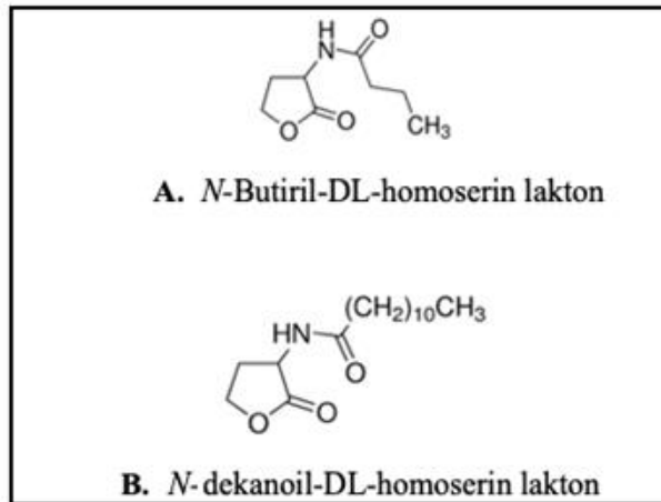
Şekil 3.7. Yarışmacı ajanlar.
