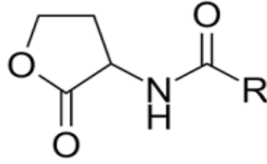
Şekil 2.3. Lakton moleküllerinin genel kimyasal yapıları.
