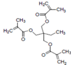
Trimetilolpropan Trimetakrilat
