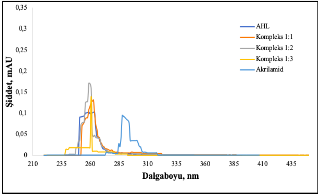
Şekil 4.1. C6-HSL/Akrilamid komplekslerine ait spektrofotometrik grafikler pH 7.0, T:25 °C.
