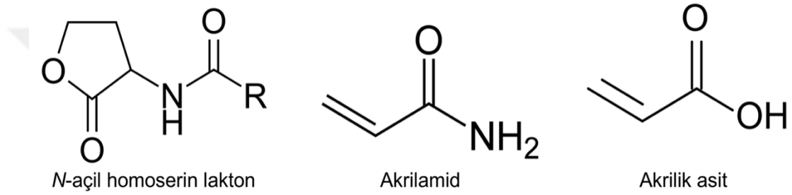
Şekil 3.1. N-açıl-homoserin lakton, akrilamid ve akrilik asit moleküllerinin kimyasal yapıları.
