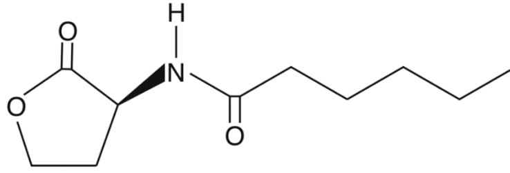
Şekil 2.5. C6-HSL yapısı.
