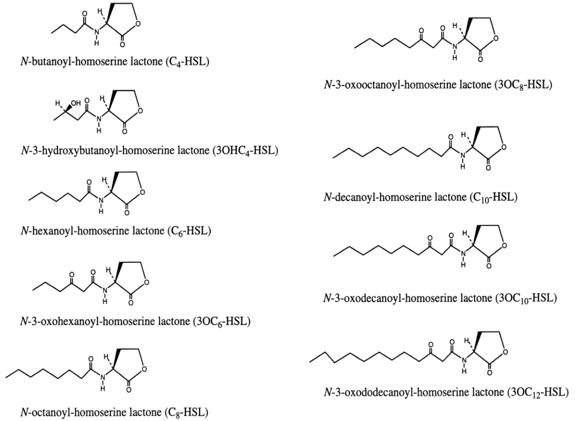
Şekil 2.2. Bazı N-açıl homoserinlerin laktonların kimyasal yapıları.
