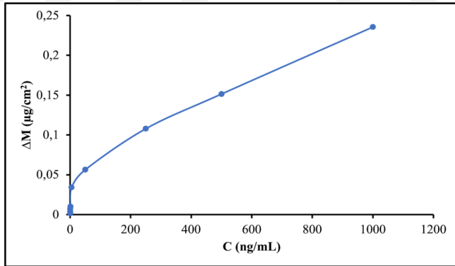
Şekil 4.12. Derişime karşı Δm değışiminin grafiđi. pH: 7.0; akış hızı: 0,5 mL/dak.; T: 25 °C.
