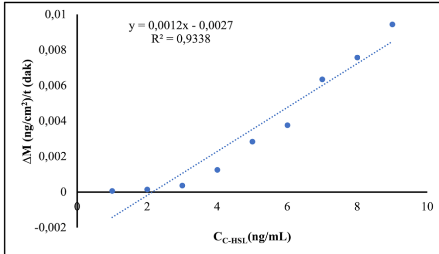
Şekil 4.16. C6-HSL baskılanmış QCM sensörün denge kinetik analiz doğrusu.
