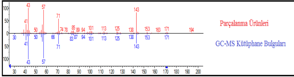
C6-HSL Parçalanma Ürünleri ve Kütüphane Bulguları ile Eşleştirilmesi
