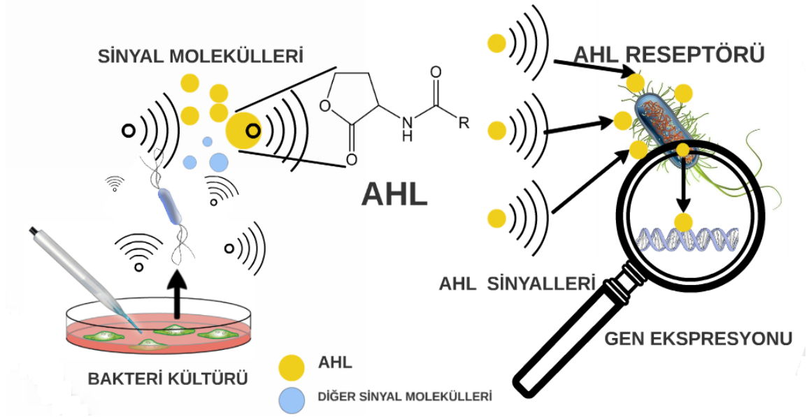
Şekil 2.4. Bakterilerin AHL üretimi, sinyal moleküllerinin bakteri reseptörü ile alınışının ve gen ekspresyonunun şematize edilmiş şekli.
