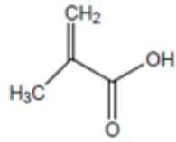
Metakrilik Asit
