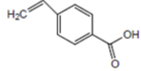
p-vinil Benzoik Asit
