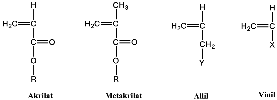
Şekil 2. 18 Bazı monomerlerin polimerleşme hızlarına göre sıralanışı
