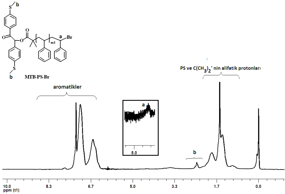
Şekil 4. 47 MTB sonlu fonksiyonel PS(MTB-PS)' nin ^1\text{H} NMR spektrumu
