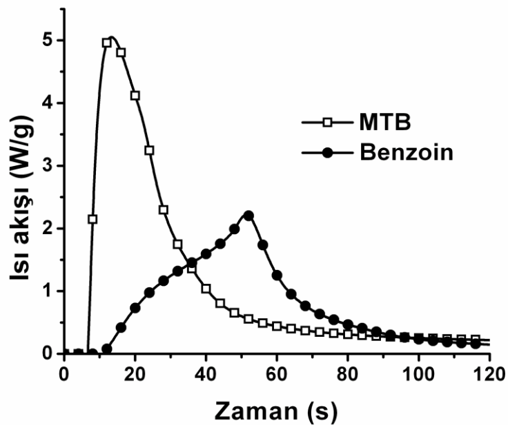
Şekil 4. 8 MTB (% 0,1, w/w ), Benzoin (% 0,1, w/w ) fotobaşlatıcıları varlığında epoksi diakrilatın (% 80 EA + % 20 TPGDA) Foto-DSC ile elde edilen polimerizasyonunun ısı akışı grafiği (Işık yoğunluğu= 15 \text{ mW cm}^{-2} )
