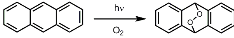
řekil 2. 26 Antrasen molekülünün UV ışık ve oksijen varlığında endoperoksit oluřturması
