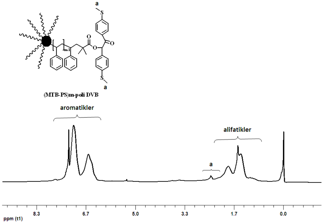
Şekil 4. 49 Çok kollu (MTB-PS) m -poli DVB yıldız polimerik başlatıcısının 1 H NMR spektrumu
