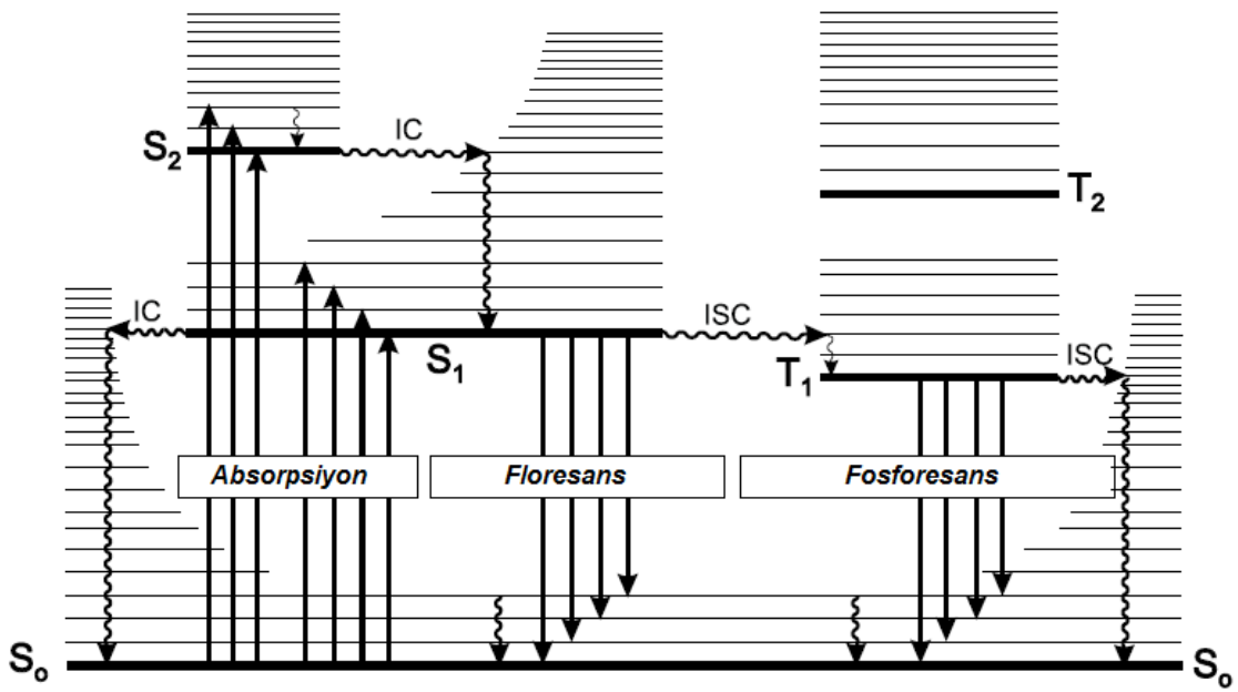
Şekil 2. 6 Jablonski Diyagramı
