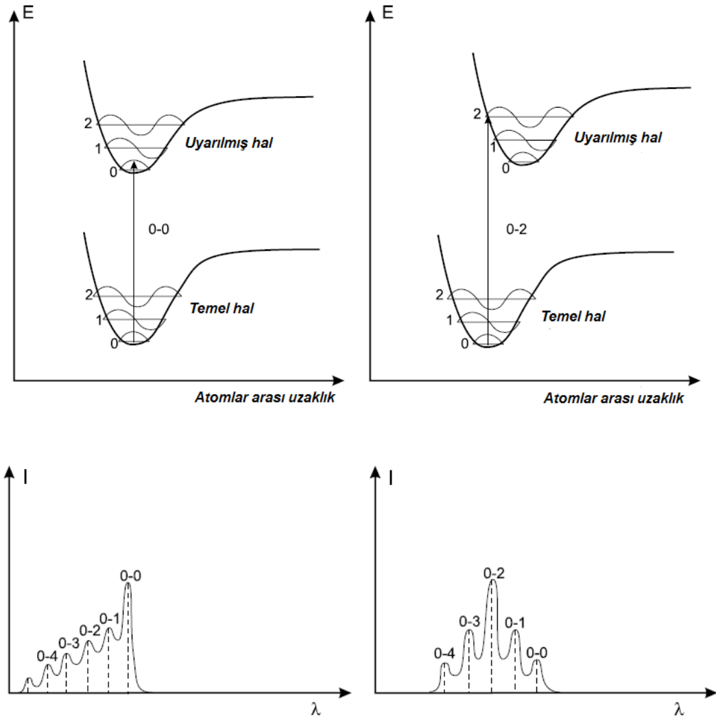
Şekil 2. 10 Franck-Condon Geçişi (Dikey geçişlerin potansiyel enerji diyagramları)
