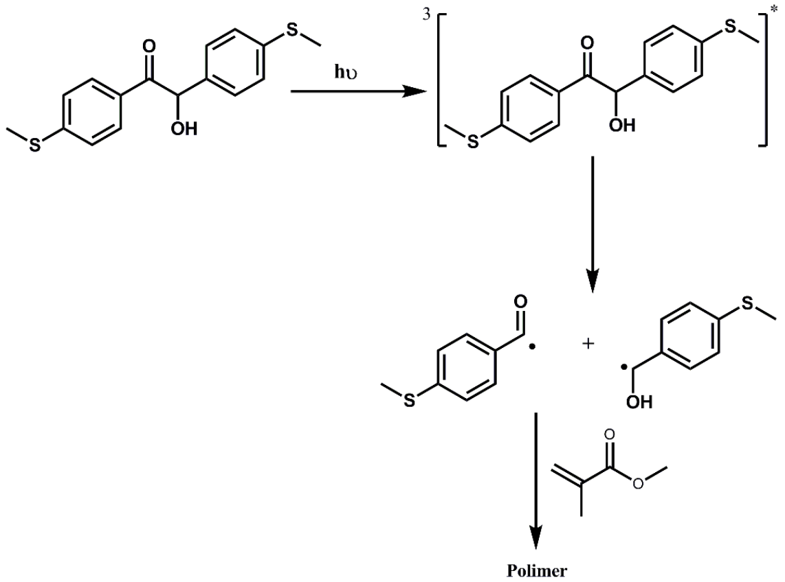
Şekil 5. 1 4,4'-MTB için önerilen fotobaşlatma mekanizması
