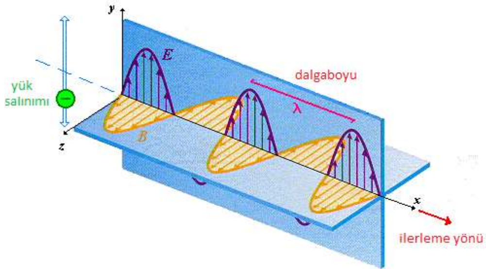
Şekil 2. 1 Elektromanyetik dalga
