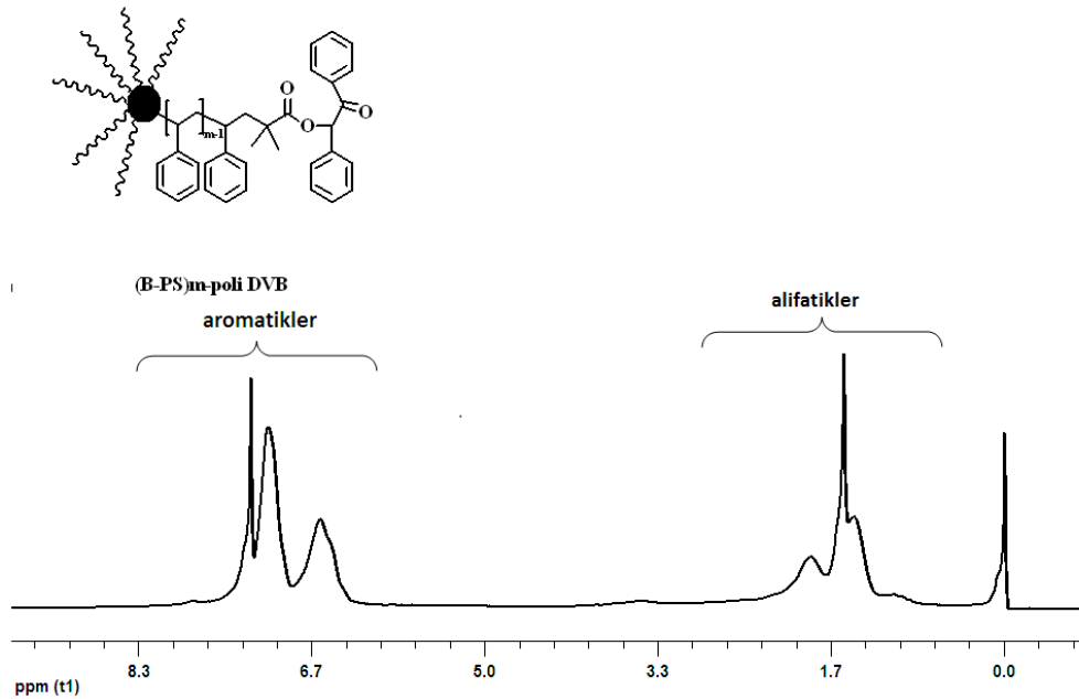
Şekil 4. 65 Çok kollu (Benzoin-PS)m-poli DVB yıldız polimerinin 1 H NMR spektrumu
