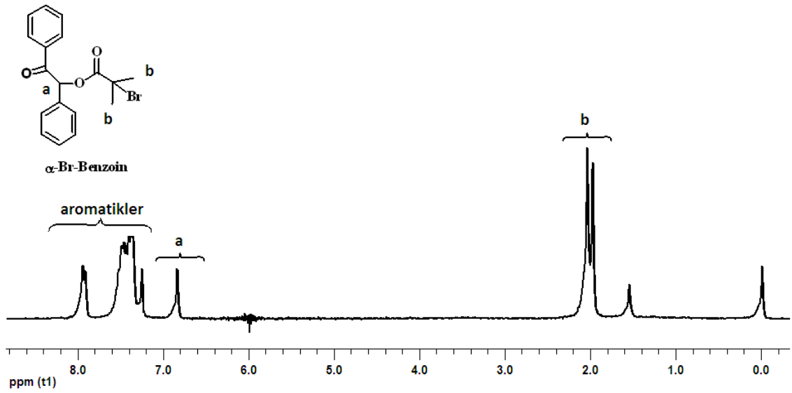
Şekil 4. 61 α- bromofonksiyonel benzoinin 1 H NMR spektrumu
