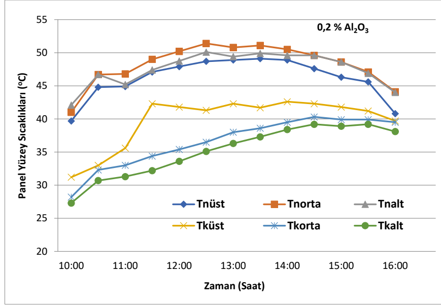
Şekil 7.19. Kanatçıksız ve %0,2 oranında levha kanatçıklı \text{Al}_2\text{O}_3 -su soğutmalı panellerin ön yüz sıcaklıklarının gün boyunca değişimi
