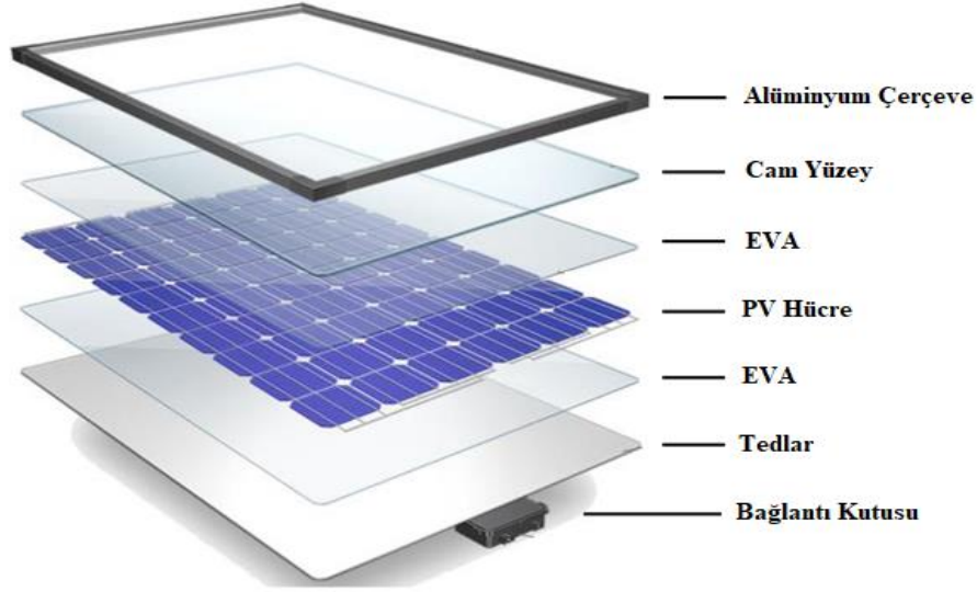
Şekil 3.8. Fotovoltaik hücre yapısını meydana getiren materyaller
