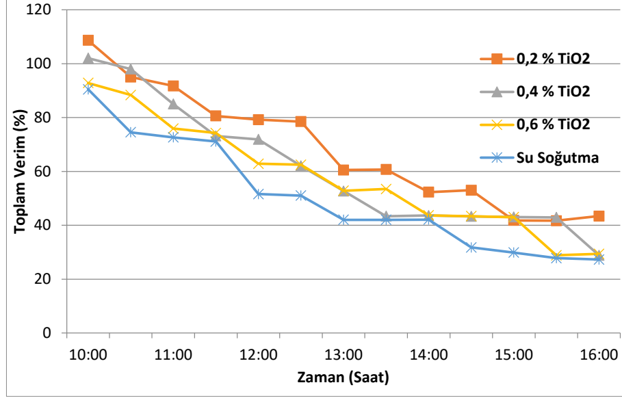
Şekil 7.82. Levha kanatçıklı bir panelde su soğutmalı ve farklı oranlardaki \text{TiO}_2 -su soğutmalı panellerin toplam verimlerinin gün boyunca değişimi
