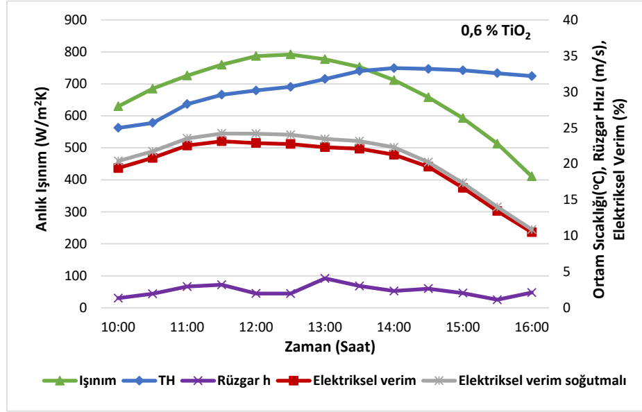
Şekil 7.49. Kanatçiksız-soğutmasız ve ağırlıkça %0,6 oranında levha kanatçıklı \text{TiO}_2 -su soğutmalı-panellere ait elektriksel verimin anlık ışınlam, ortam sıcaklığı ve rüzgâra göre gün boyunca değişimi
