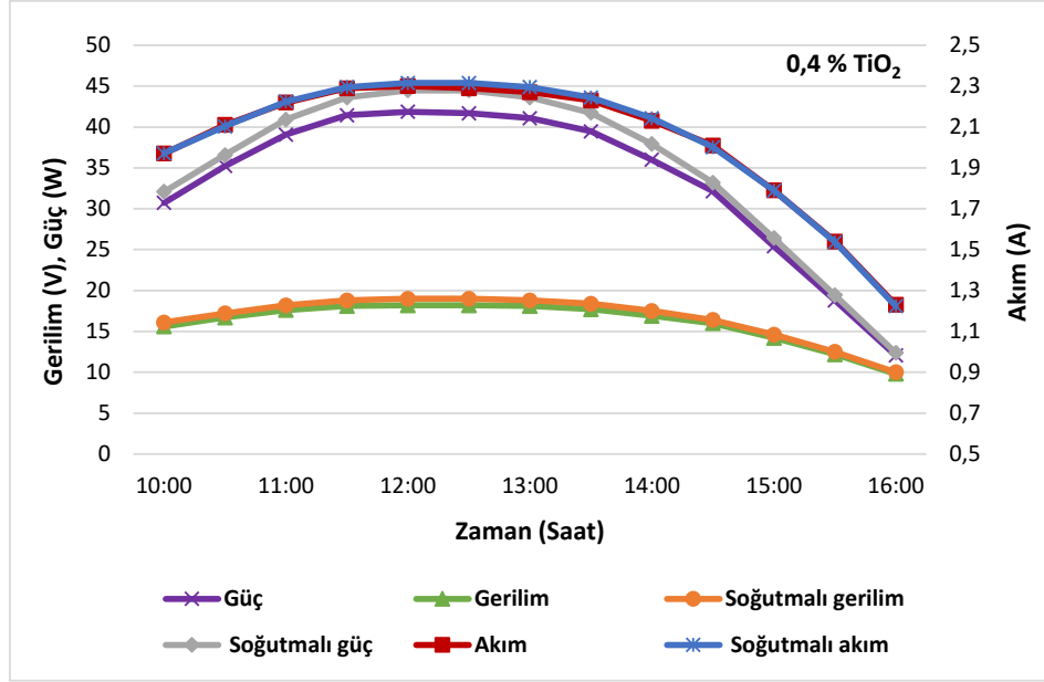
Şekil 7.45. Kanatçıksız ve %0,4 oranında levha kanatçıklı \text{TiO}_2 -su soğutmalı panellerin akım, gerilim ve güç değerlerinin gün boyunca değişimi
