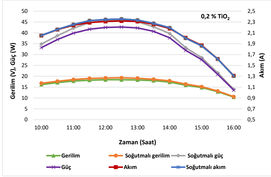
Şekil 7.44. Kanatçıksız ve %0,2 oranında levha kanatçıklı TiO 2 -su soğutmalı panellerin akım, gerilim ve güç değerlerinin gün boyunca değişimi
