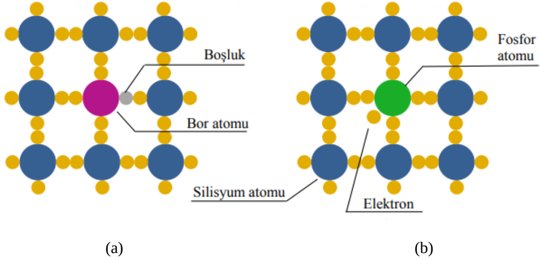
Şekil 3.5. (a) p tipi yarı iletken (b) n tipi yarı iletken [59]
