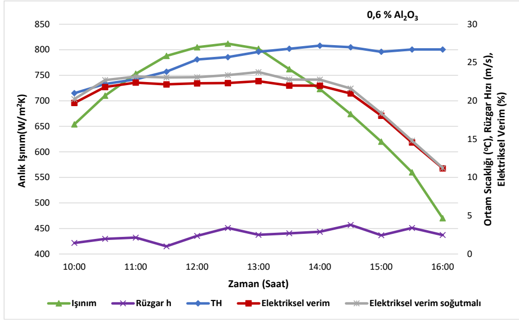
Şekil 7.31. Kanatçiksız-soğutmasız ve ağırlıkça %0,6 oranında levha kanatıklı \text{Al}_2\text{O}_3 -su soğutmalı panellere ait elektriksel verimin anlık ışıınım, ortam sıcaklığı ve rüzgâra göre gün boyunca değişimi
