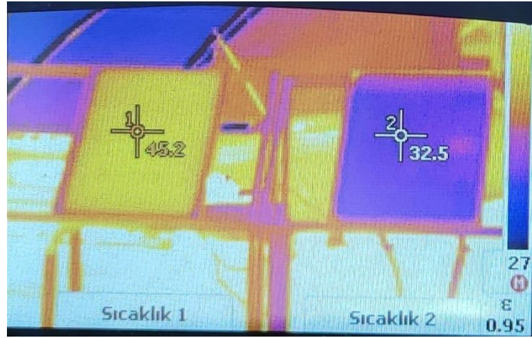
Şekil 7.23. Ağırlıkça %0,4 oranında levha kanatçıklı \text{Al}_2\text{O}_3 -su nanoakışkan soğutmalı ve soğutmasız panellere ait ön taraftan çekilen termal kamera görüntüsü
