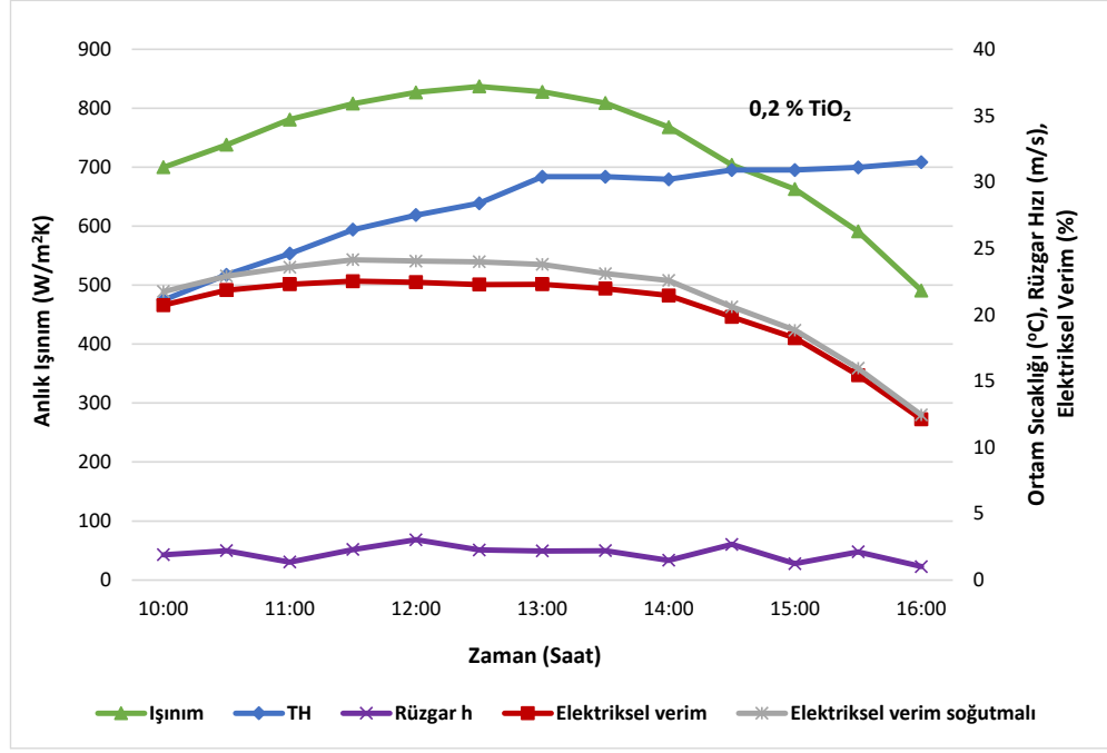
Şekil 7.47. Kanatçıksız-soğutmasız ve ağırlıkça %0,2 oranında levha kanatçıklı TiO 2 -su soğutmalı panellere ait elektriksel verimin anlık ışınlam, ortam sıcaklığı ve rüzgâra göre gün boyunca değişimi
