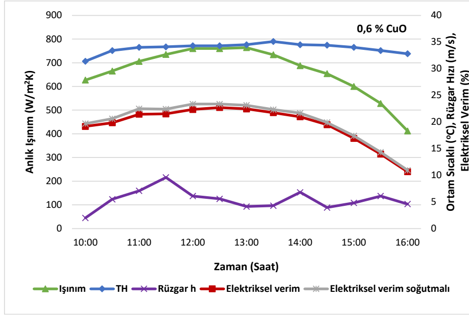
Şekil 7.65. Kanatçıksız-soğutmasız ve ağırlıkça %0,6 oranında levha kanatçıklı CuO-su soğutmalı panellere ait elektriksel verimin anlık ışınlam, ortam sıcaklığı ve rüzgâra göre gün boyunca değişimi
