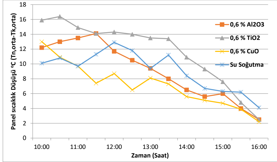
Şekil 7.71. Levha kanatçıklı bir panelde su soğutmalı ve %0,6 oranındaki Al 2 O 3 -su-TiO 2 -su-CuO-su soğutmalı panellerin kanatçıksız panele göre orta noktalarındaki sıcaklık düşüşlerinin gün boyunca değişimi
