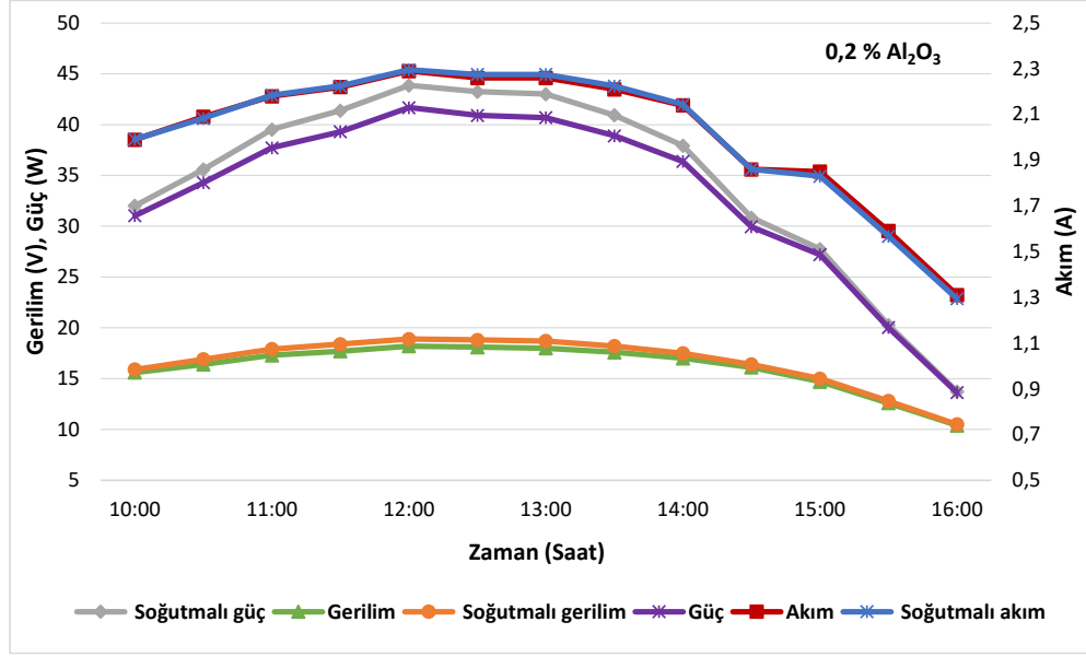
Şekil 7.26. Kanatçıksız ve %0,2 oranında levha kanatçıklı \text{Al}_2\text{O}_3 -su soğutmalı panellerin akım, gerilim ve güç değerlerinin gün boyunca değişimi
