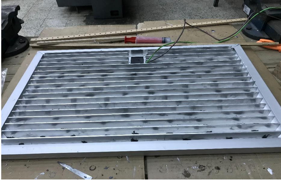
Şekil 6.3. Levha kanatçıkların panele yapıştırılması
