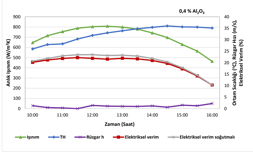
Şekil 7.30. Kanatçıksız-soğutmasız ve ağırlıkça %0,4 oranında levha kanatçıklı \text{Al}_2\text{O}_3 -su soğutmalı panellere ait elektriksel verimin anlık ışıınım, ortam sıcaklığı ve rüzgâra göre gün boyunca değişimi
