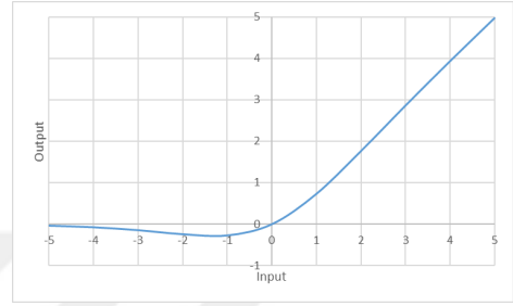
(d) Swish Activation Function
