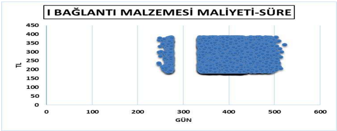
Şekil 5.3 Süre-ı bağlantı malzemesi maliyeti etkileşim grafiği
