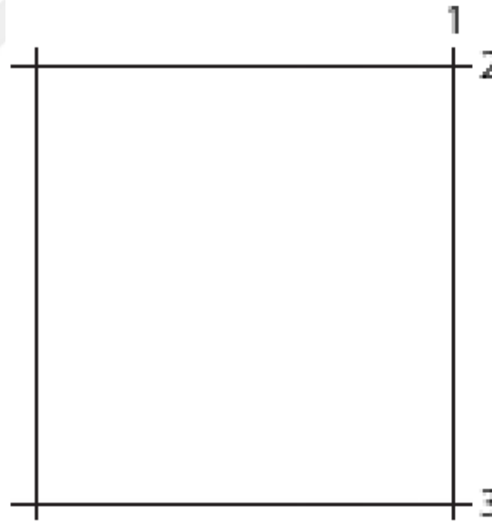
Şekil 3.7: Yüzeylerin oluşturulması
