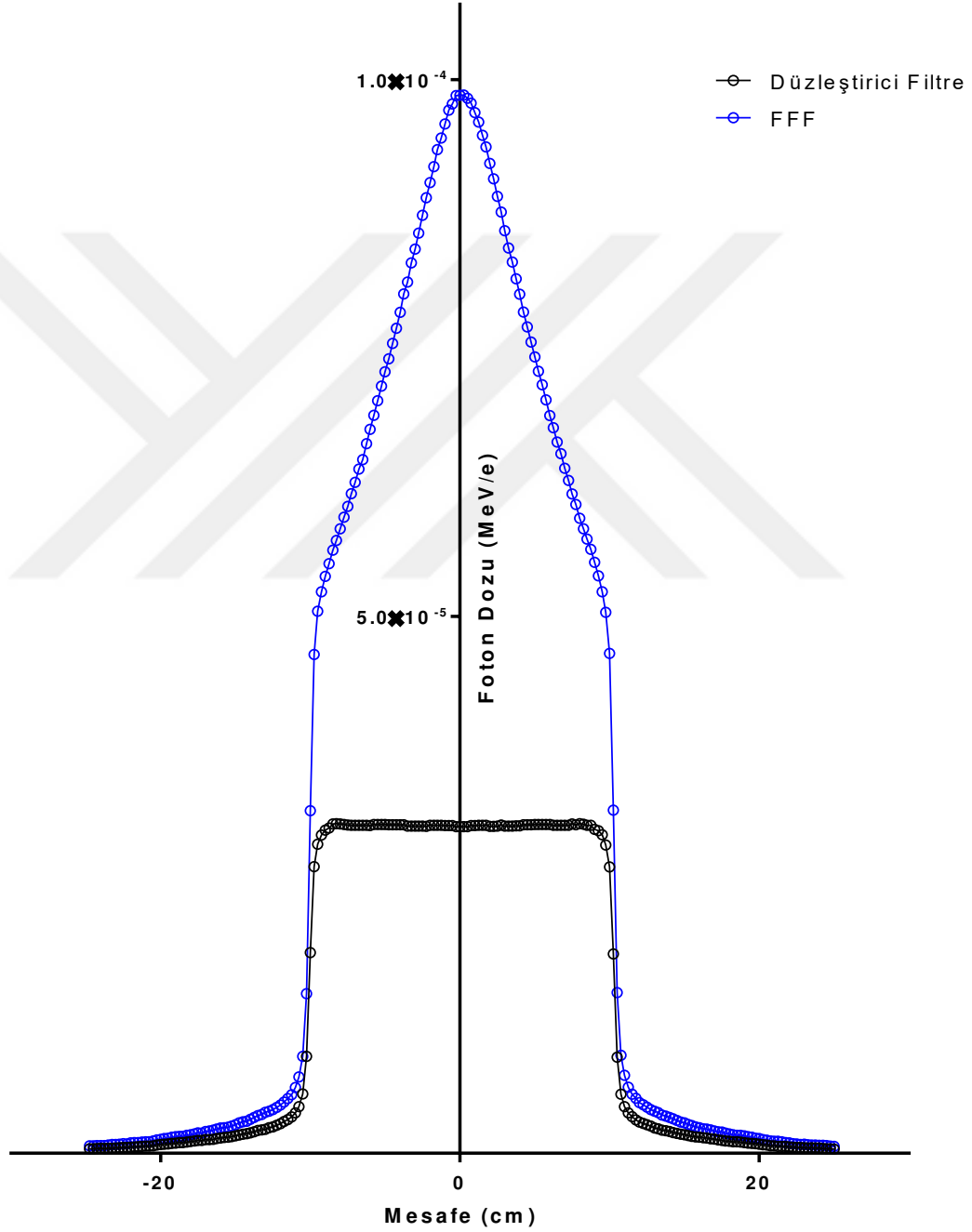
Şekil 4.12: 18 MV foton enerjisi ile 20x20 alan açıklığında filtreli ve filtresiz sistemde birim elektrondan elde edilen doz profili değerleri
