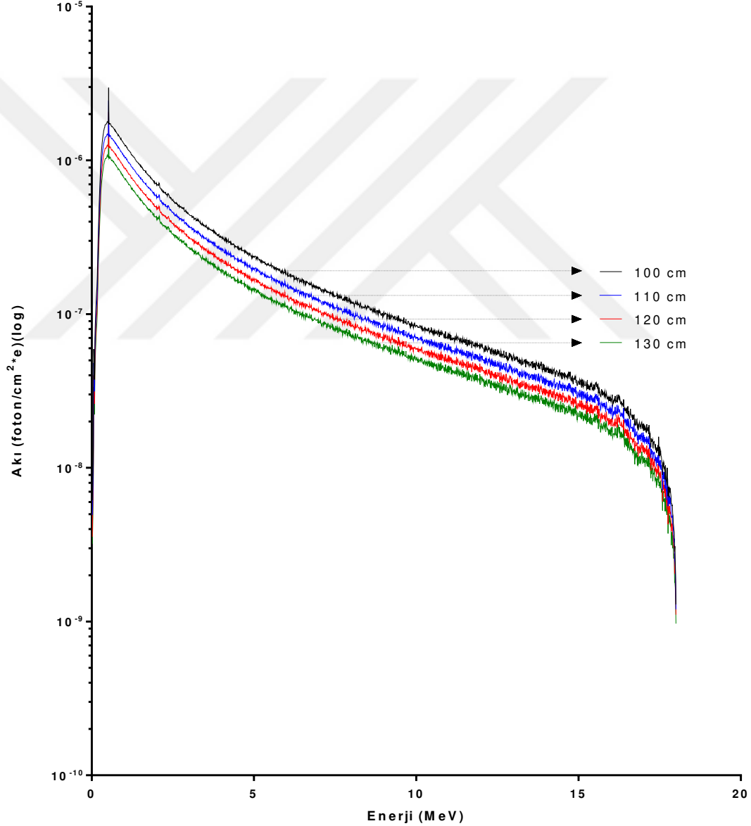
Şekil 4.5: 18 MV foton enerjisinde 10x10 alan açıklığında filtersiz sistemde hedeften farklı uzaklıklarda foton spektrumları
