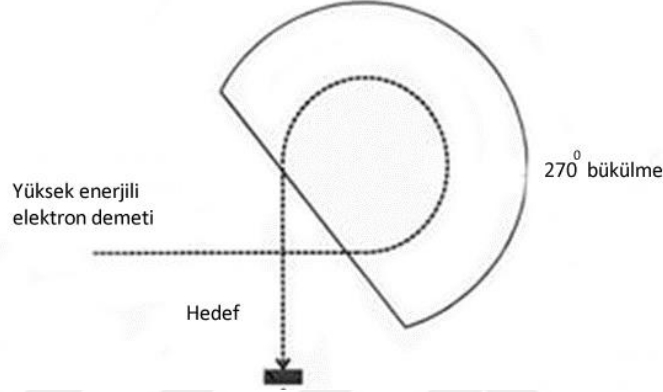
Şekil 2.15: Bükücü mıknatıs 17
