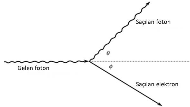
Şekil 2.2. Compton saçılması 6
