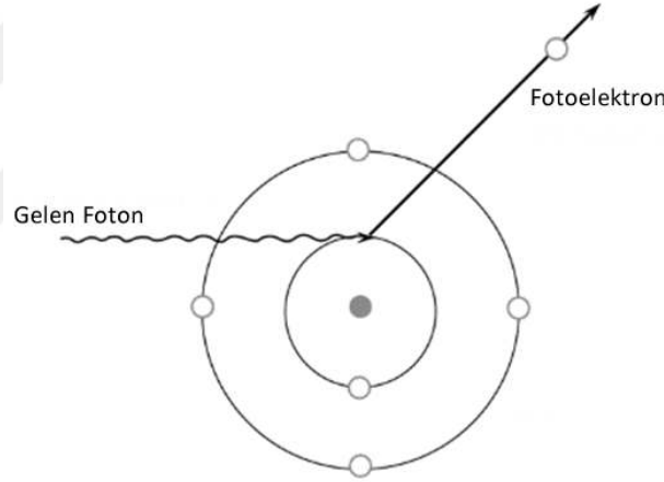
Şekil 2.5: Fotoelektrik olay 5
