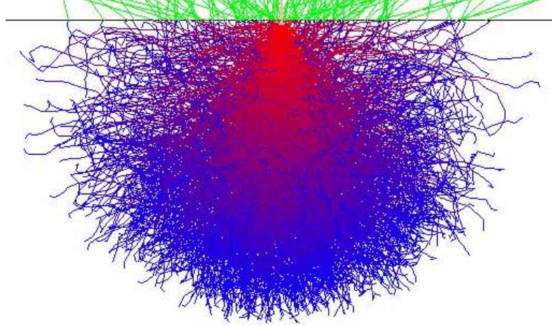
Şekil 2.20: Foton taşınımı 22
