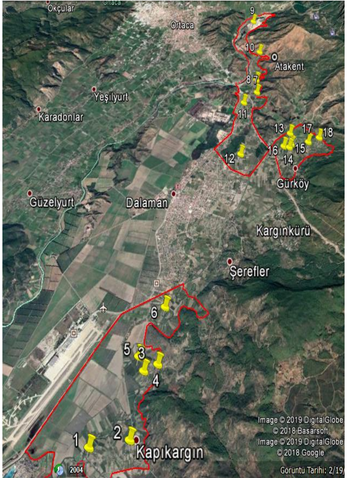
Şekil 3.1. Dalaman İlçesi Kapıkargın, Gürköy ve Atakent Yörelerinden Alınan Su Örneklem Noktaları
